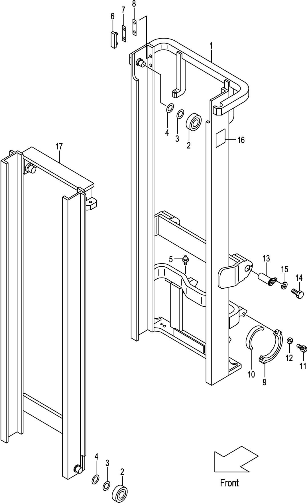
FIG.188 MAST [VM0A7,VM0A9] (M7018310) マスト
