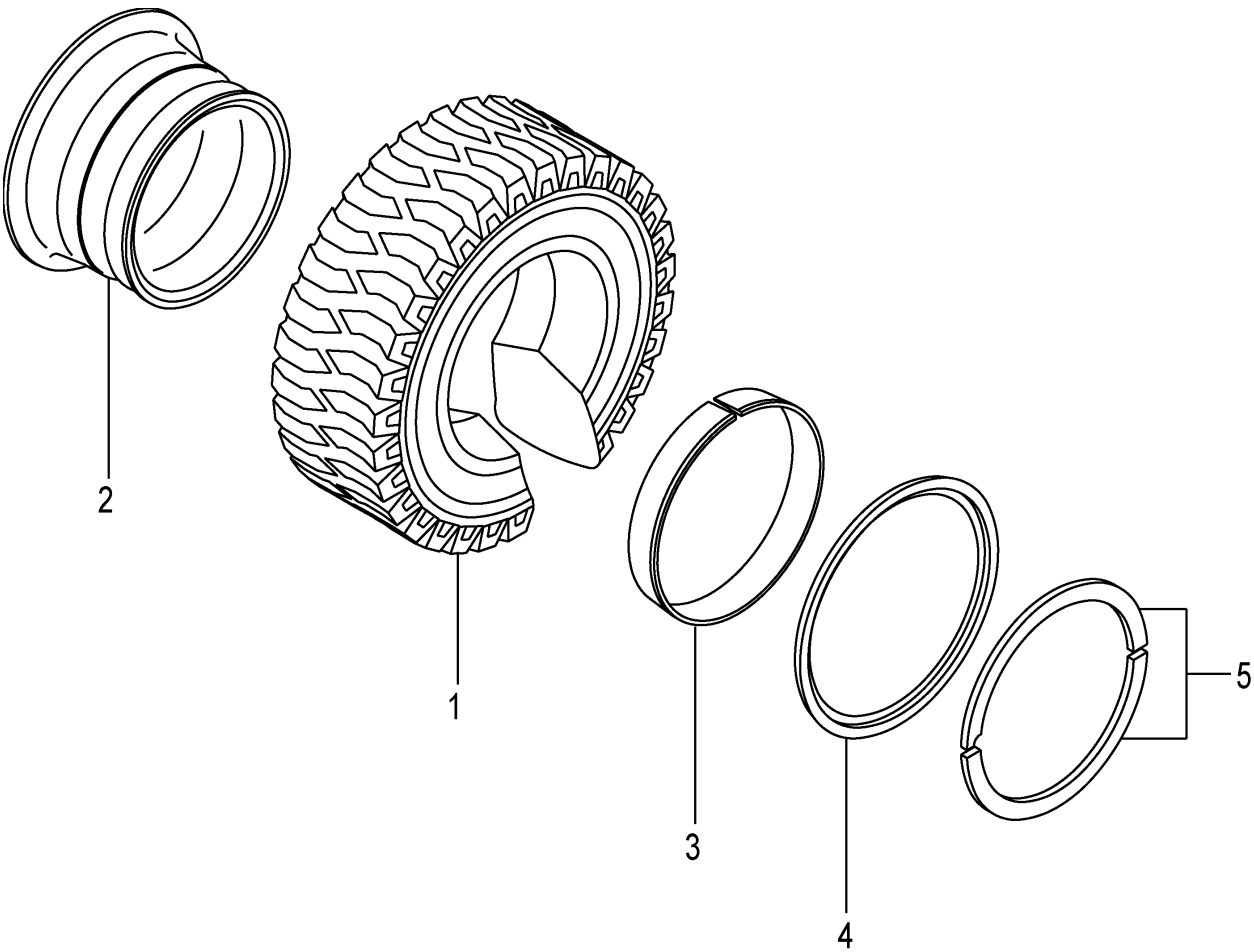
FIG.82 FRONT WHEEL (1.5T):[TUJF/DR F] (F7Z144B0) フロントホイール
