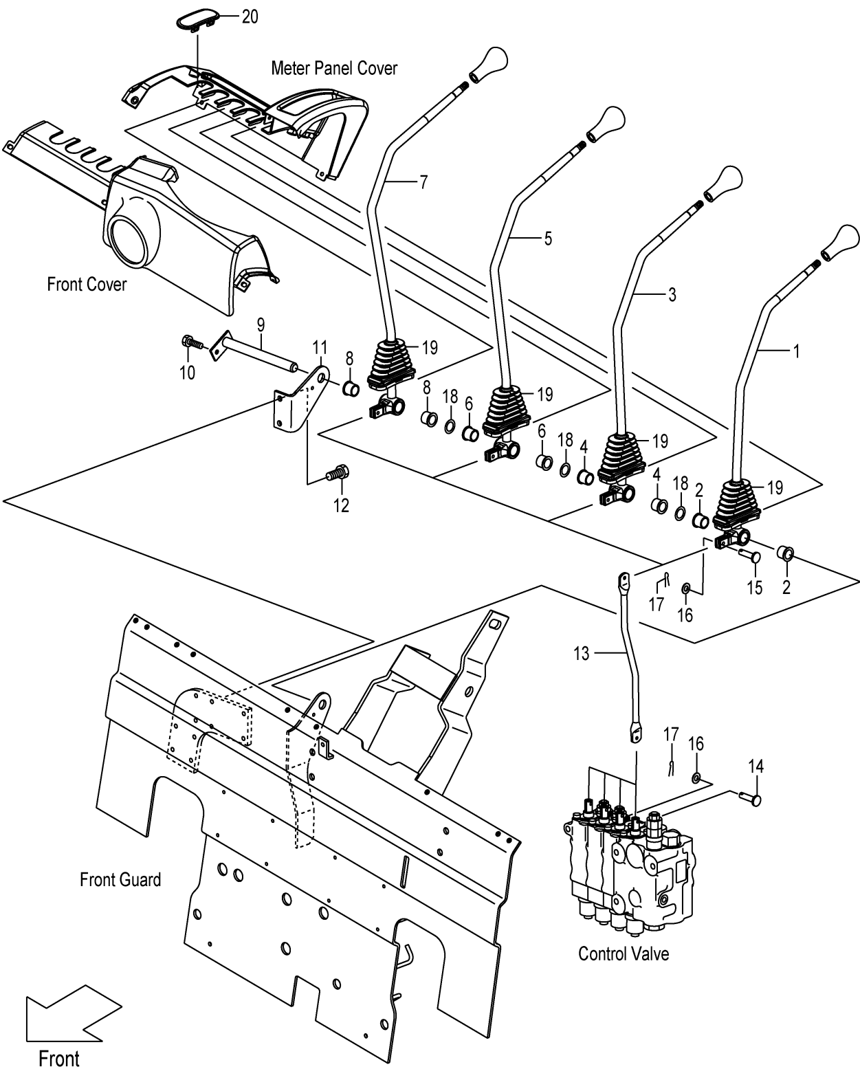
FIG.149 VALVE CONTROL [4SV] (F7Z173C0) バルブコントロール
