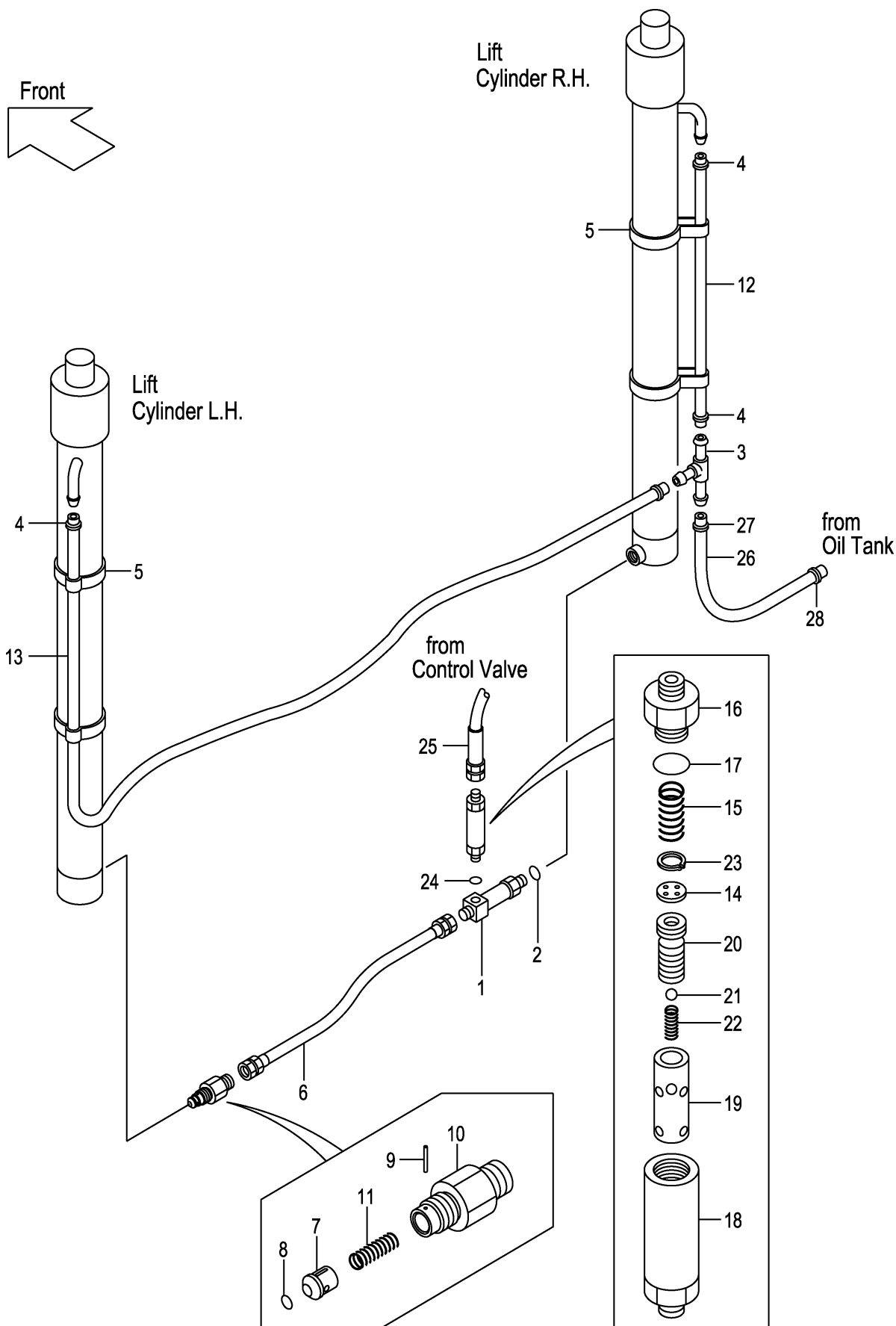
FIG.191 MAST PIPING [VM0A7,VM0A9] (M7018420) マストパイピング
