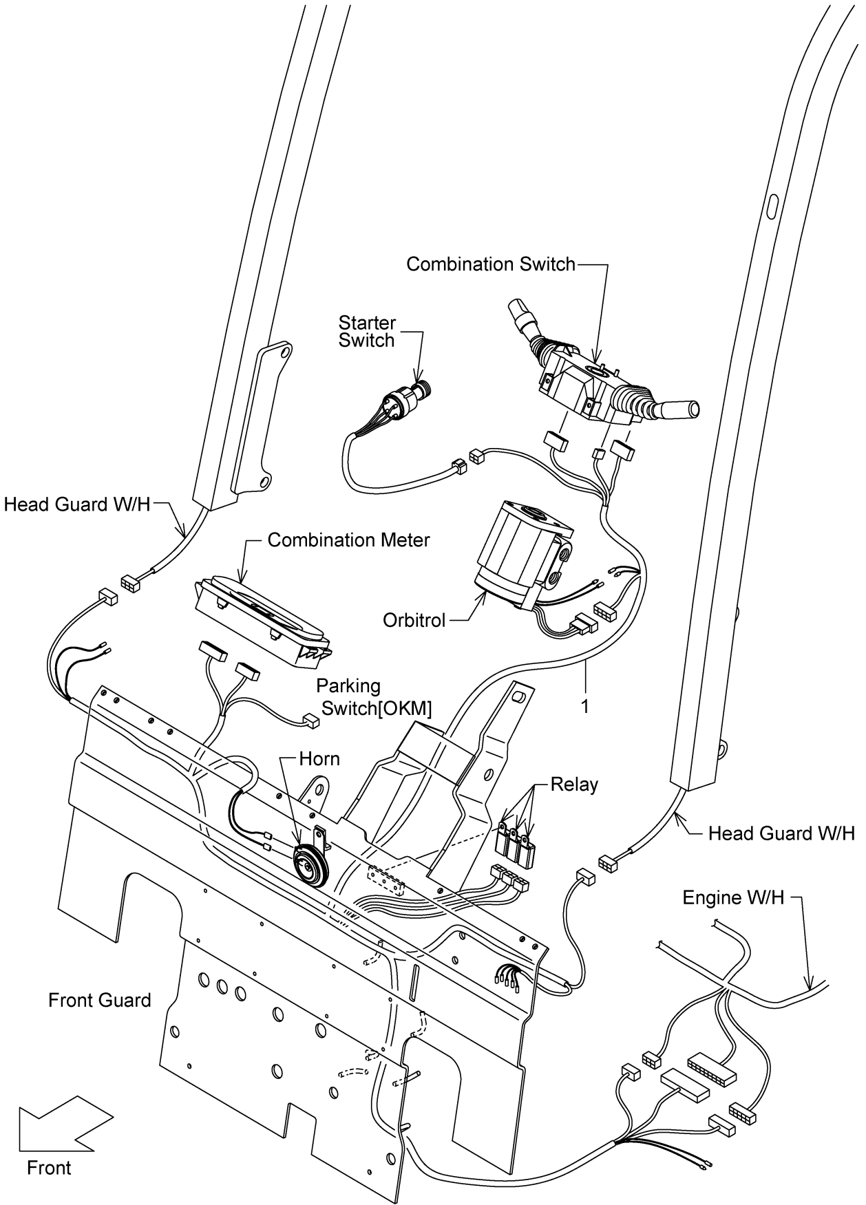
FIG.14 FRONT GUARD WIRE HARNESS (TOR-CON) (F7Z12430) フロントガードワイヤハーネス
