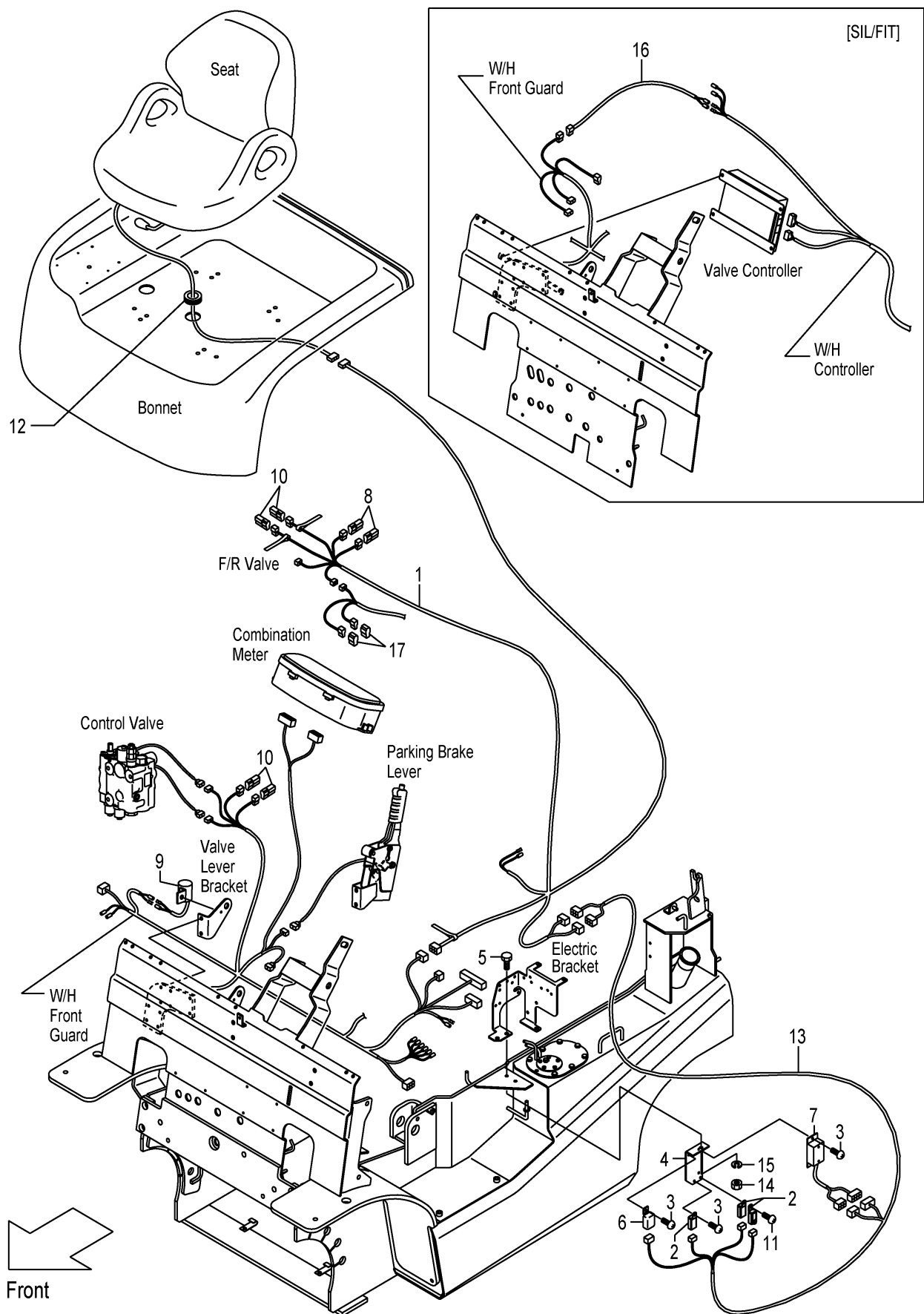
FIG.47 INTERLOCK (TOR-CON):[SIL] (F7Z126L0) インターロック
