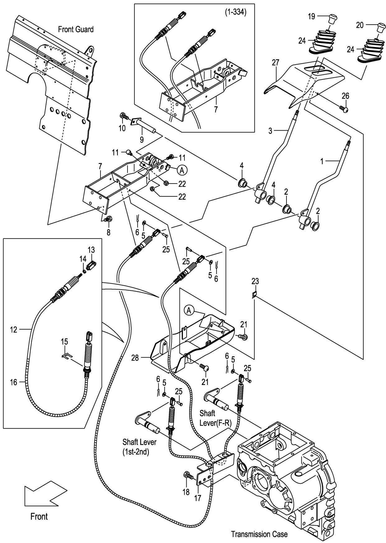
FIG.50 CHANGE LEVER (CLUTCH) (F7Z12540) チェンジレバー
