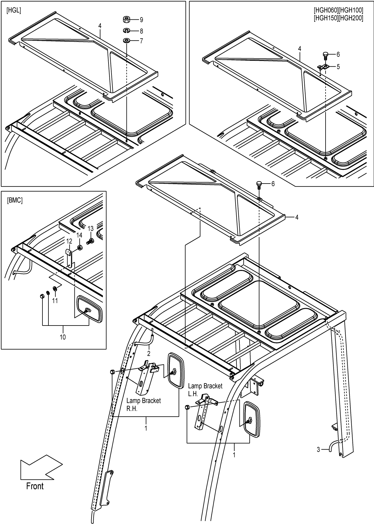
FIG.103 HEAD GUARD PARTS (F7Z151A0) ヘッドガードパーツ
