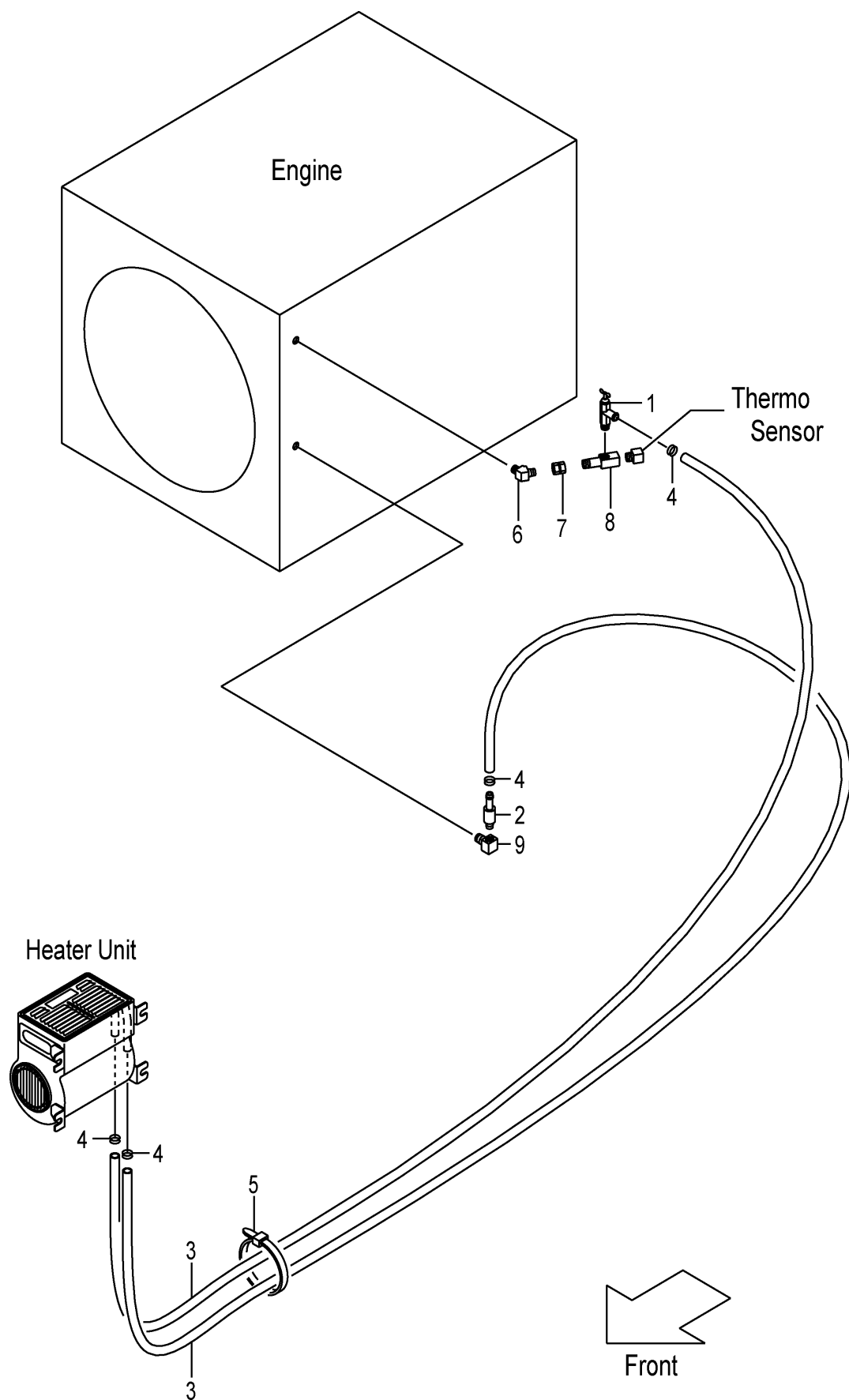
FIG.34 HEATER VALVE & ELBOW [HR] (F7Z124Z0) ヒータバルブ&エルボ
