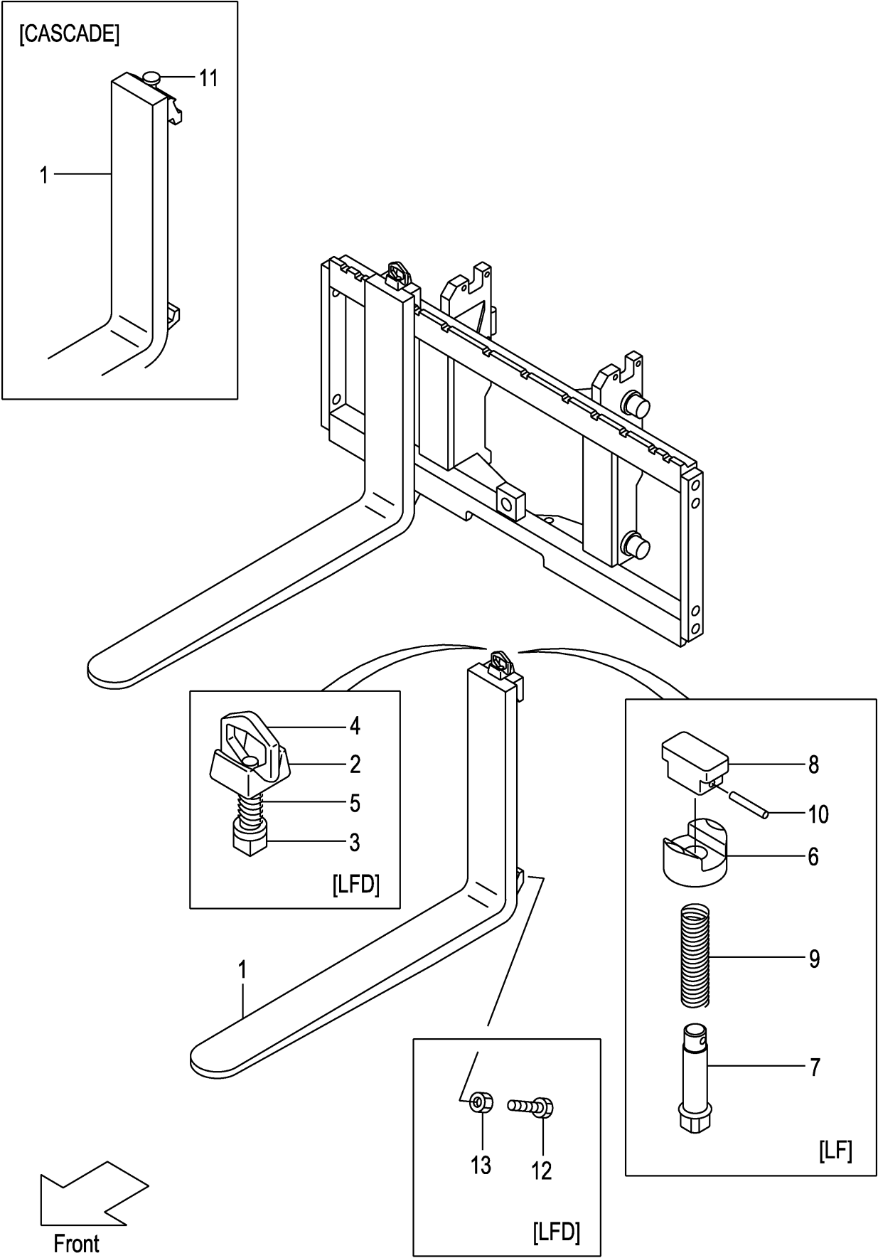
FIG.192 FORK [VFM0A7] (M7018120) フォーク
