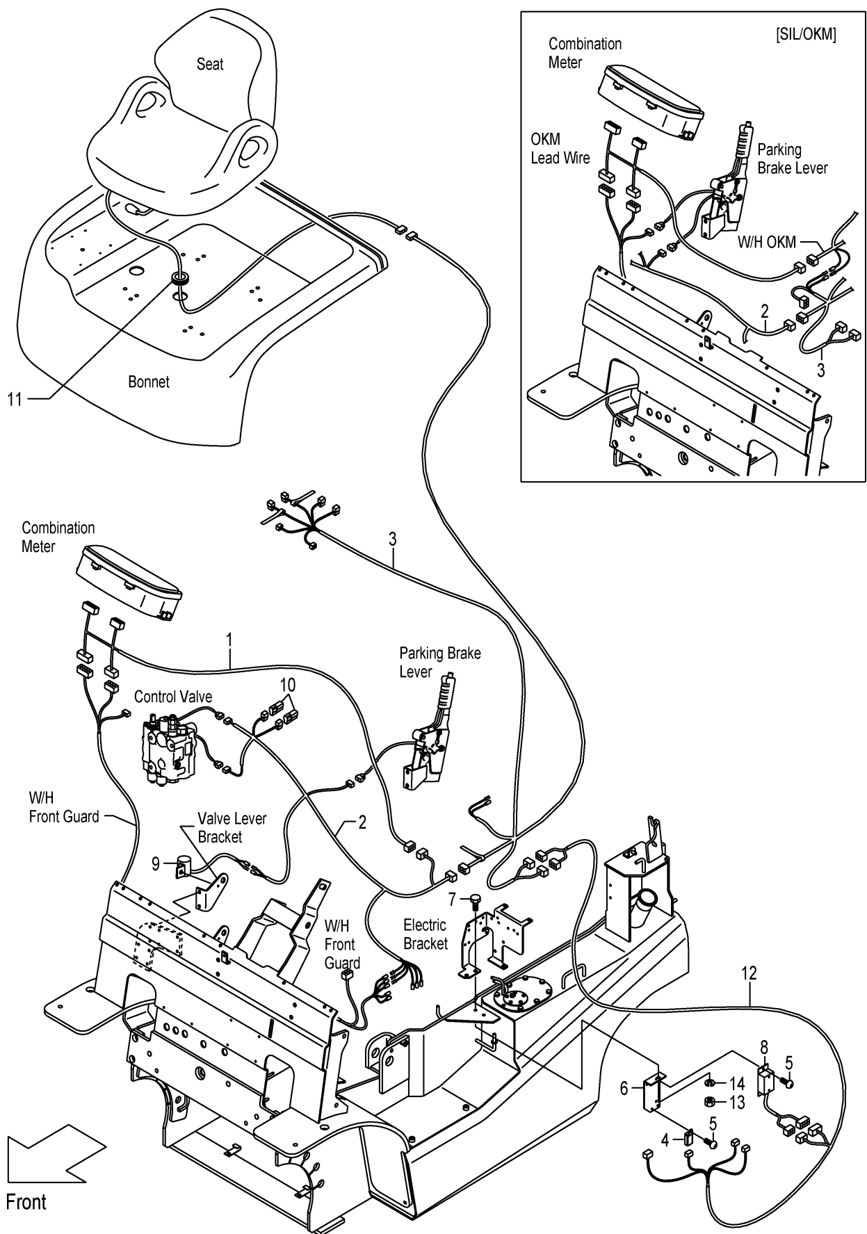
FIG.46 INTERLOCK (CLUTCH):[SIL] (F7Z126K0) インターロック
