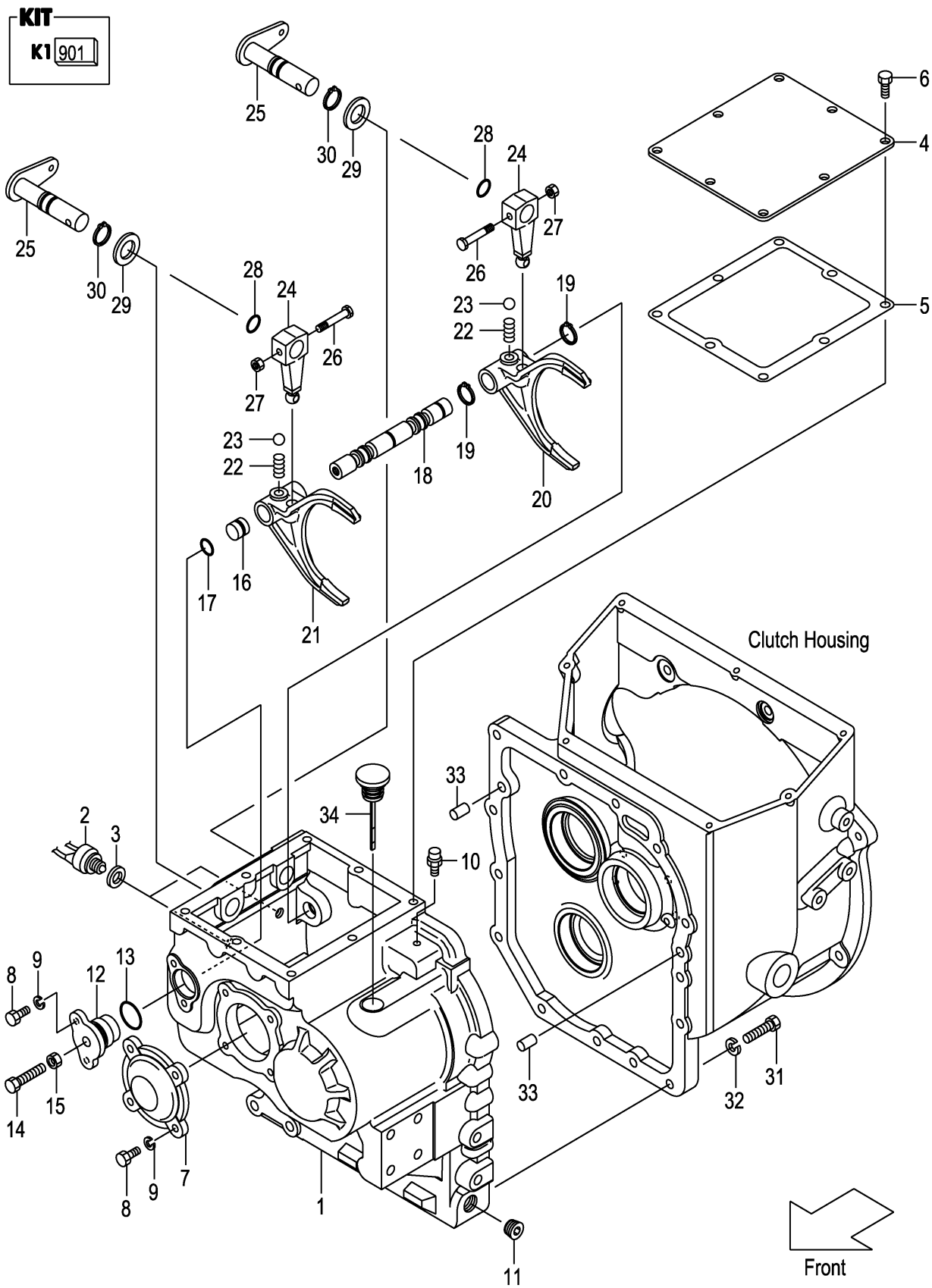
FIG.52 MISSION CASE (CLUTCH) (F7Z12560) ミッションケース
