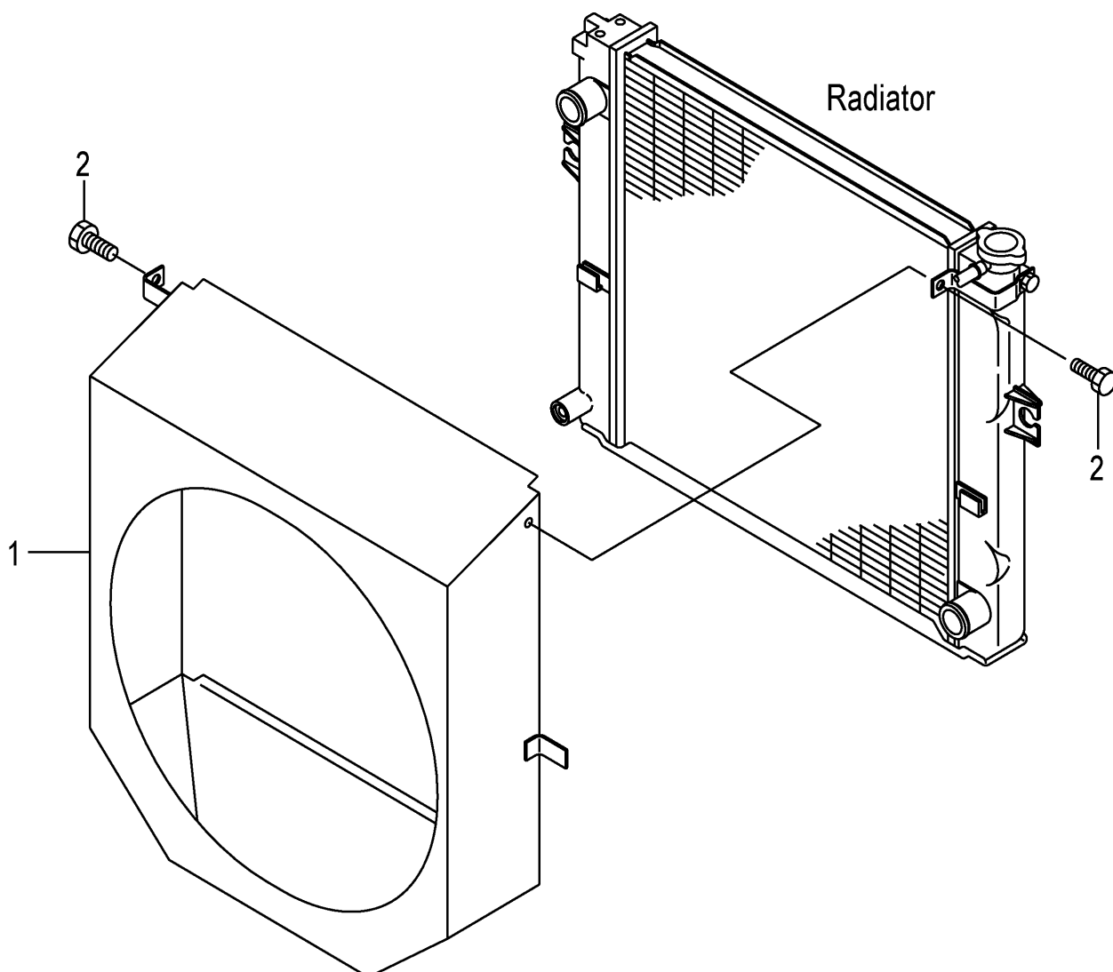
FIG.6 FAN SHROUD (F7Z12140) ファンシェラウド*
