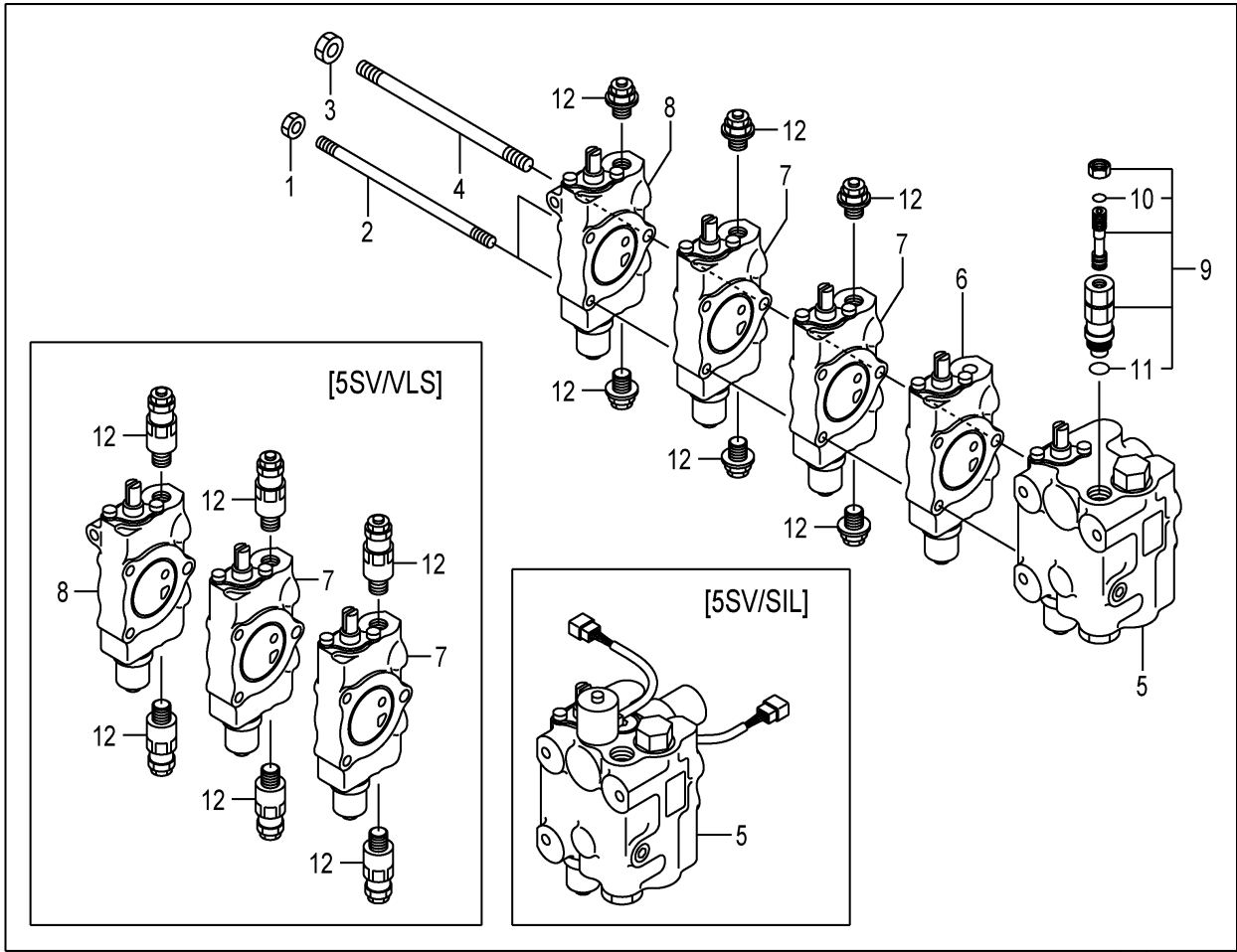
FIG.142 CONTROL VALVE [5SV] (F7Z17340) コントロールバルブ
