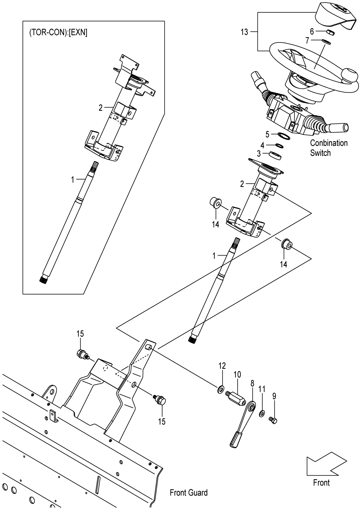
FIG.66 STEERING WHEEL UNIT (F7Z14110) ステアリングホイールユニット
