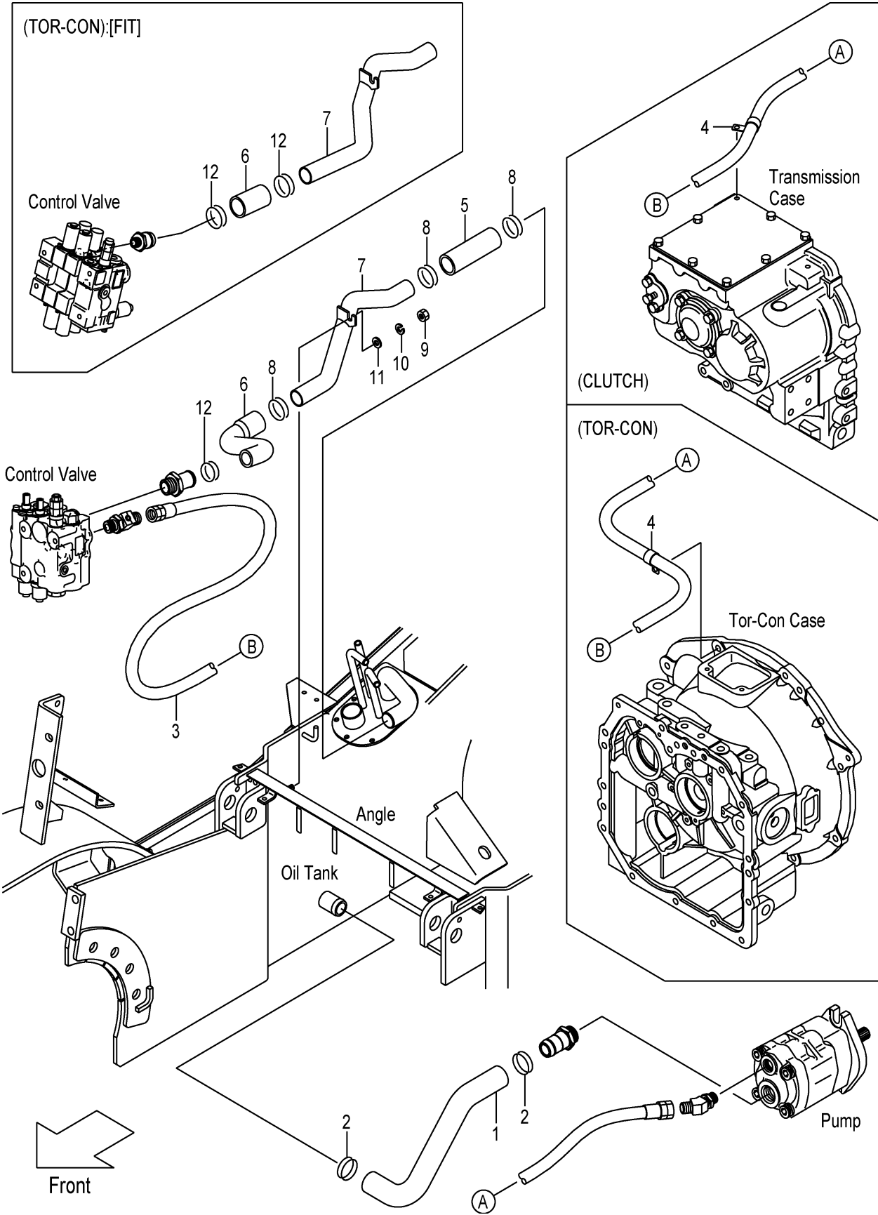
FIG.167 HYDRAULIC LINE (MAIN)(1/4) (F7Z17630) ハイドロリックライン(メイン)(1/4)
