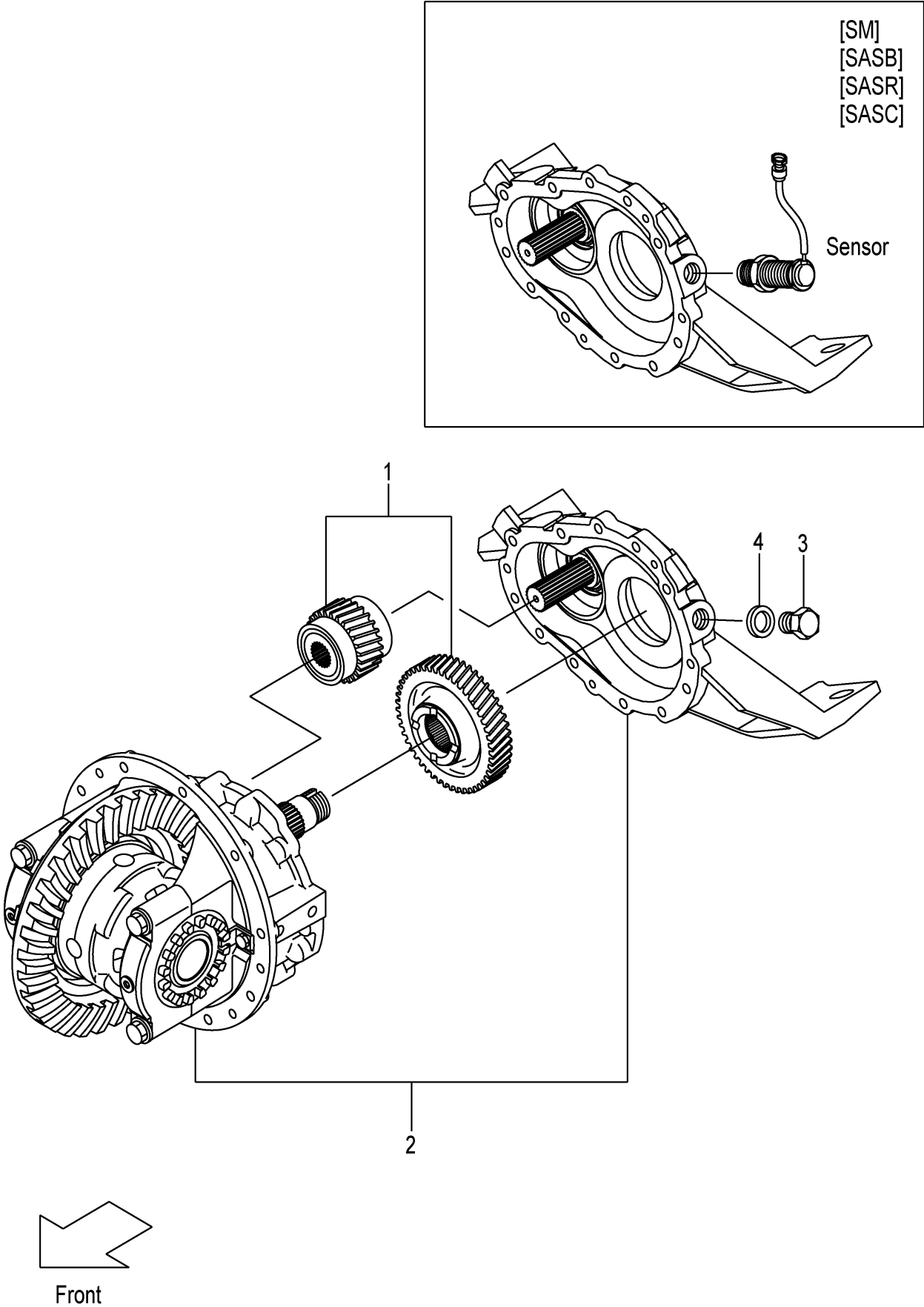
FIG.62 REDUCTION & DIFFERENTIAL (F7Z13510) リダクション&デファレンシャル
