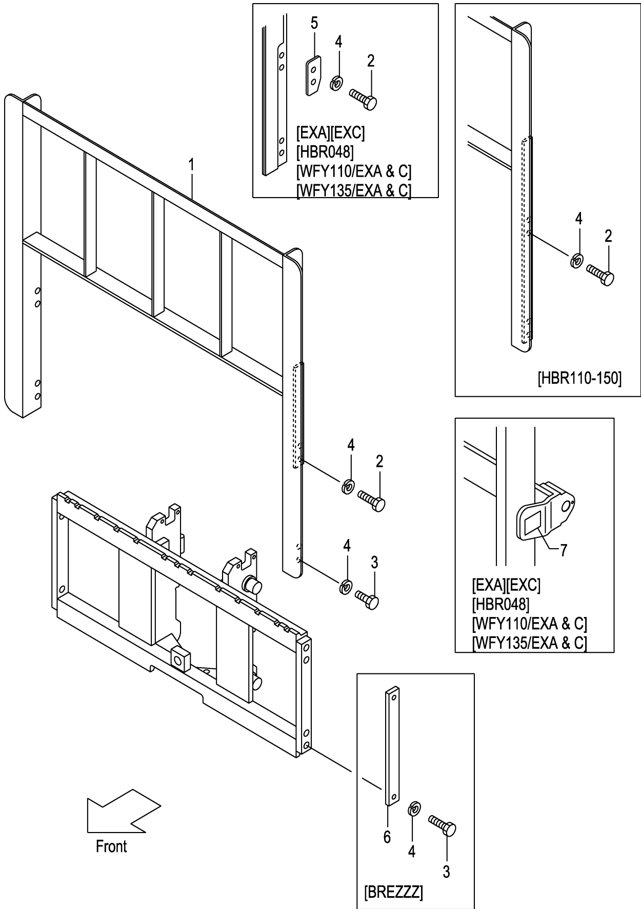
FIG.201 BACKREST [VFHM0A7] (M7018240) バックレスト
