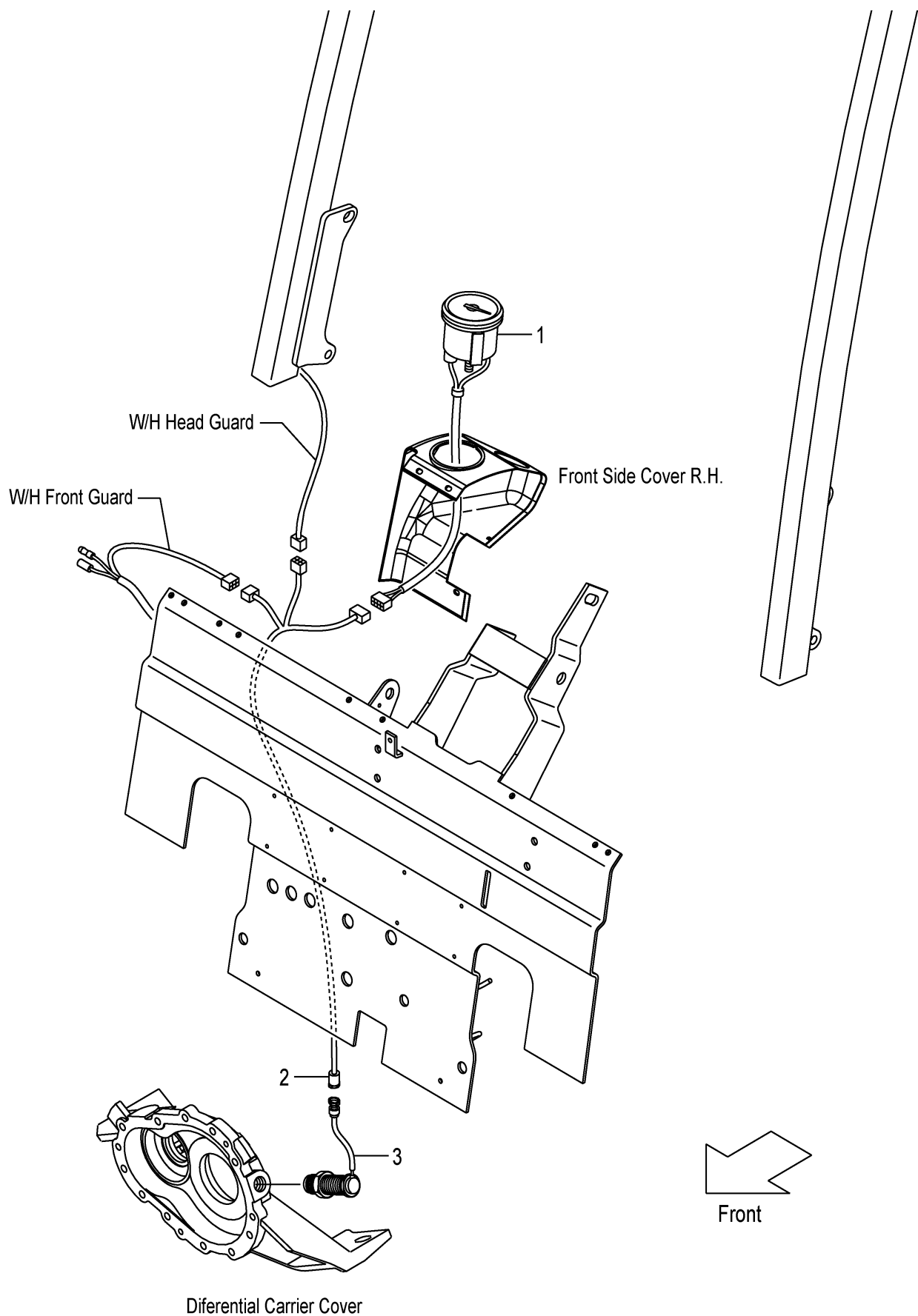
FIG.38 SPEED METER [SM] (F7Z126B0) スピードメータ
