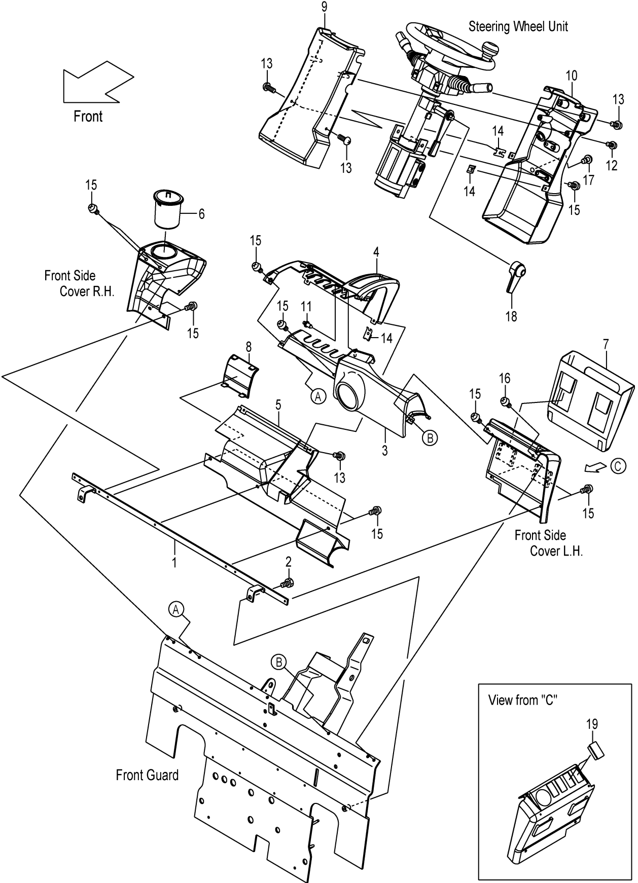
FIG.131 FRONT COVER (TOR-CON) (F7Z16480) フロントカバー
