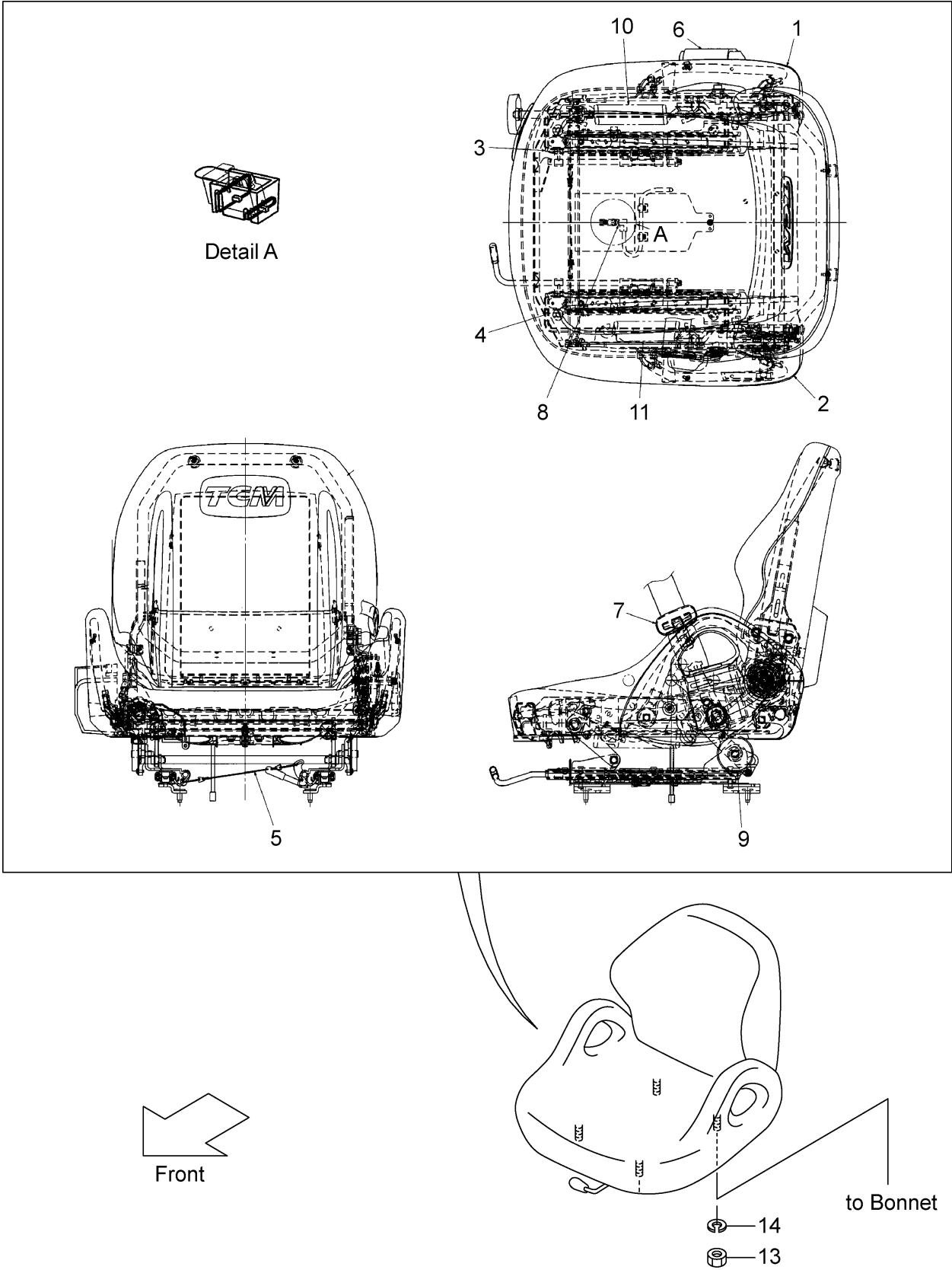
FIG.137 SEAT [OKM][OKM/SIL] (F7Z16840) シート
