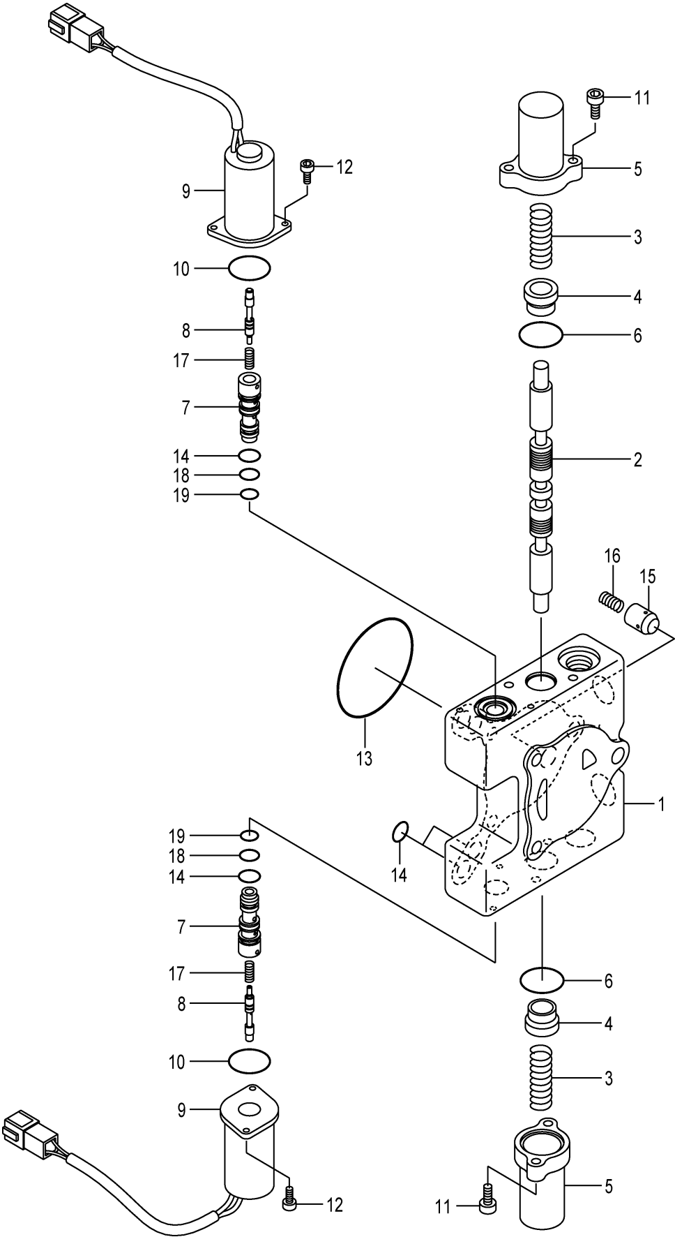
FIG.166 SPOOL SECTION (ATT)(TOR-CON):[3SV/FIT][4SV/FIT] (F7Z173U0) スプールセクション
