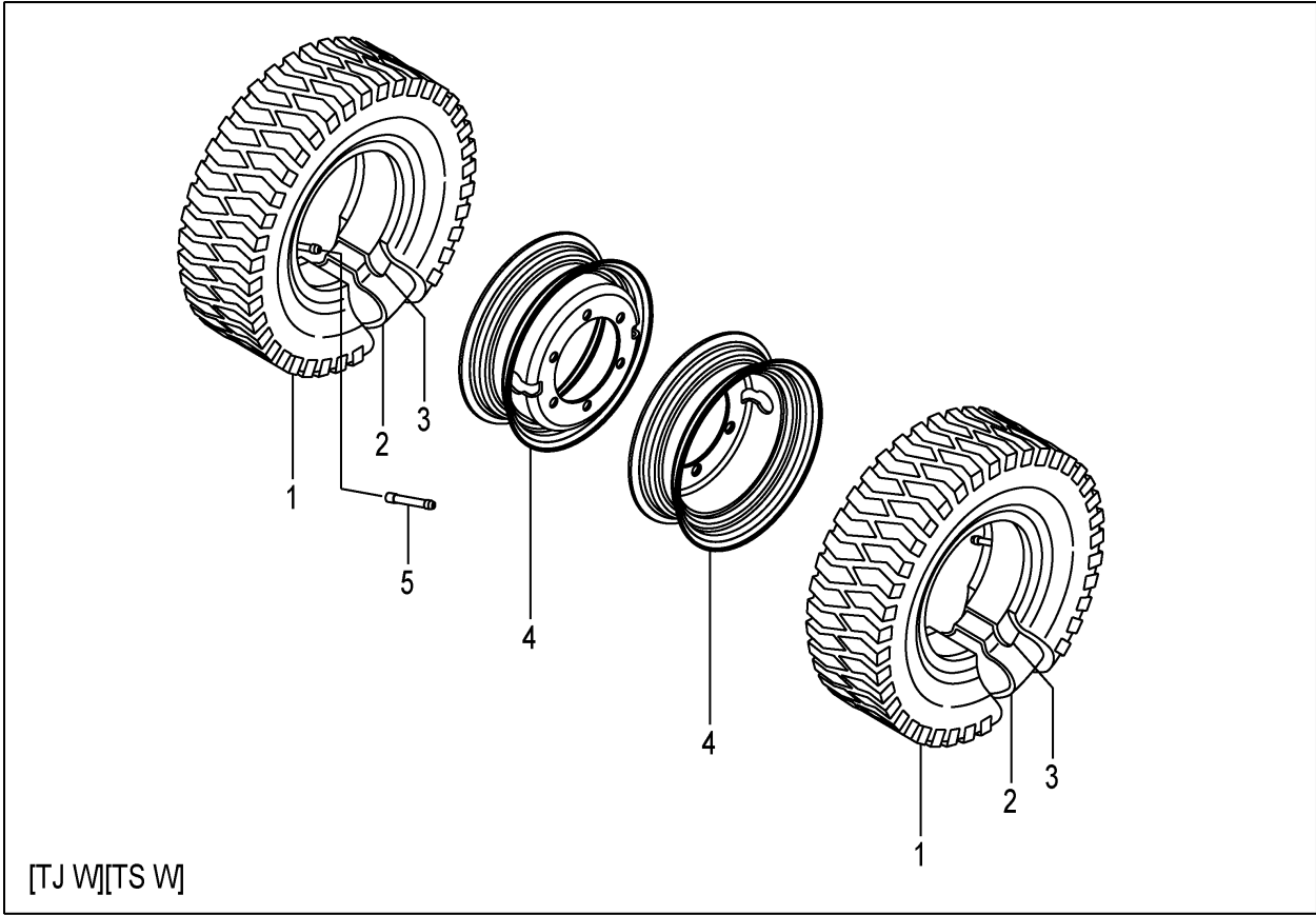
FIG.85 FRONT WHEEL [TJ W][TW][TS W] (F7Z144E0) フロントホイール
