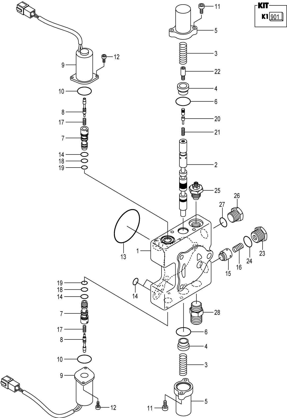
FIG.158 SPOOL SECTION (LIFT)(TOR-CON):[FIT] (F7Z173S0) スプールセクション
