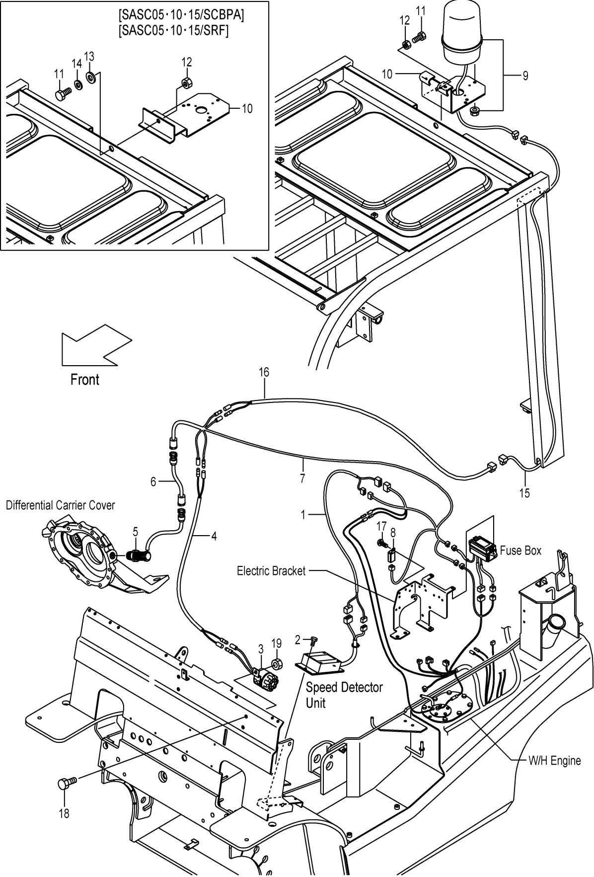
FIG.44 SPEED ALARM SYSTEM [SASC] (F7Z126H0) スピード・アラームシステム
