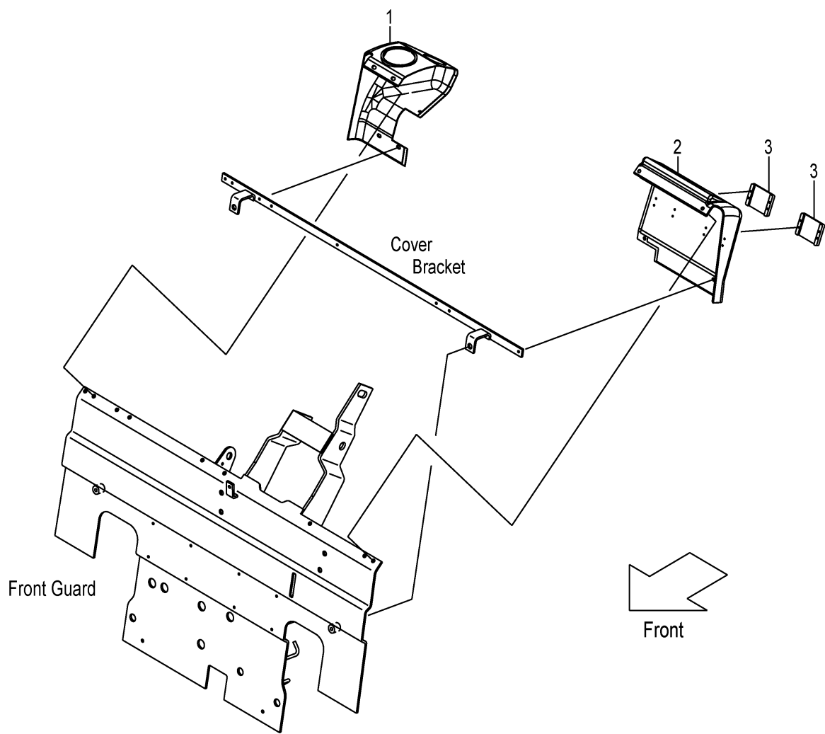
FIG.133 FRONT SIDE COVER (F7Z164C0) フロントサイドカバー
