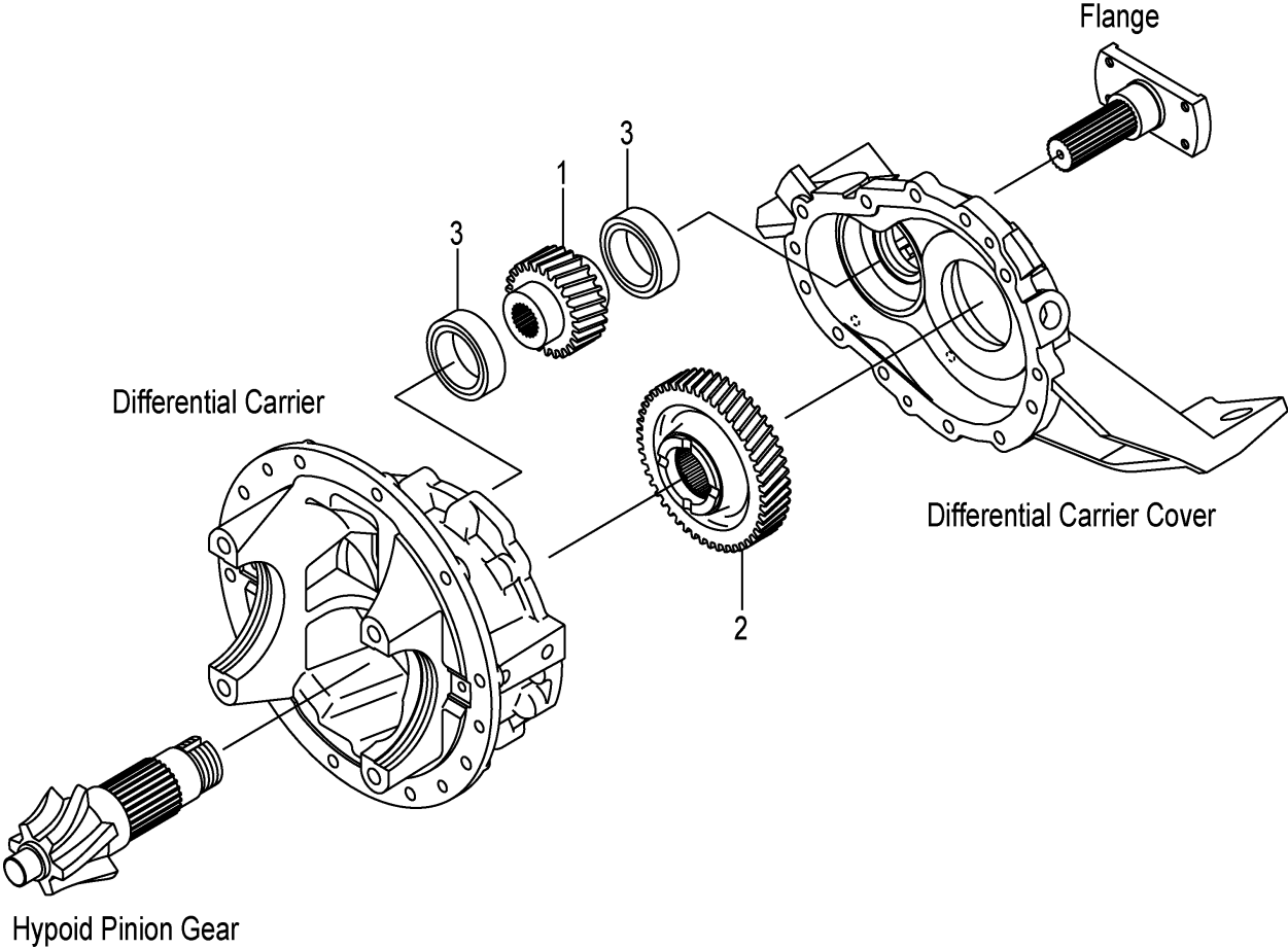
FIG.63 REDUCTION (F7Z13520) リダクション
