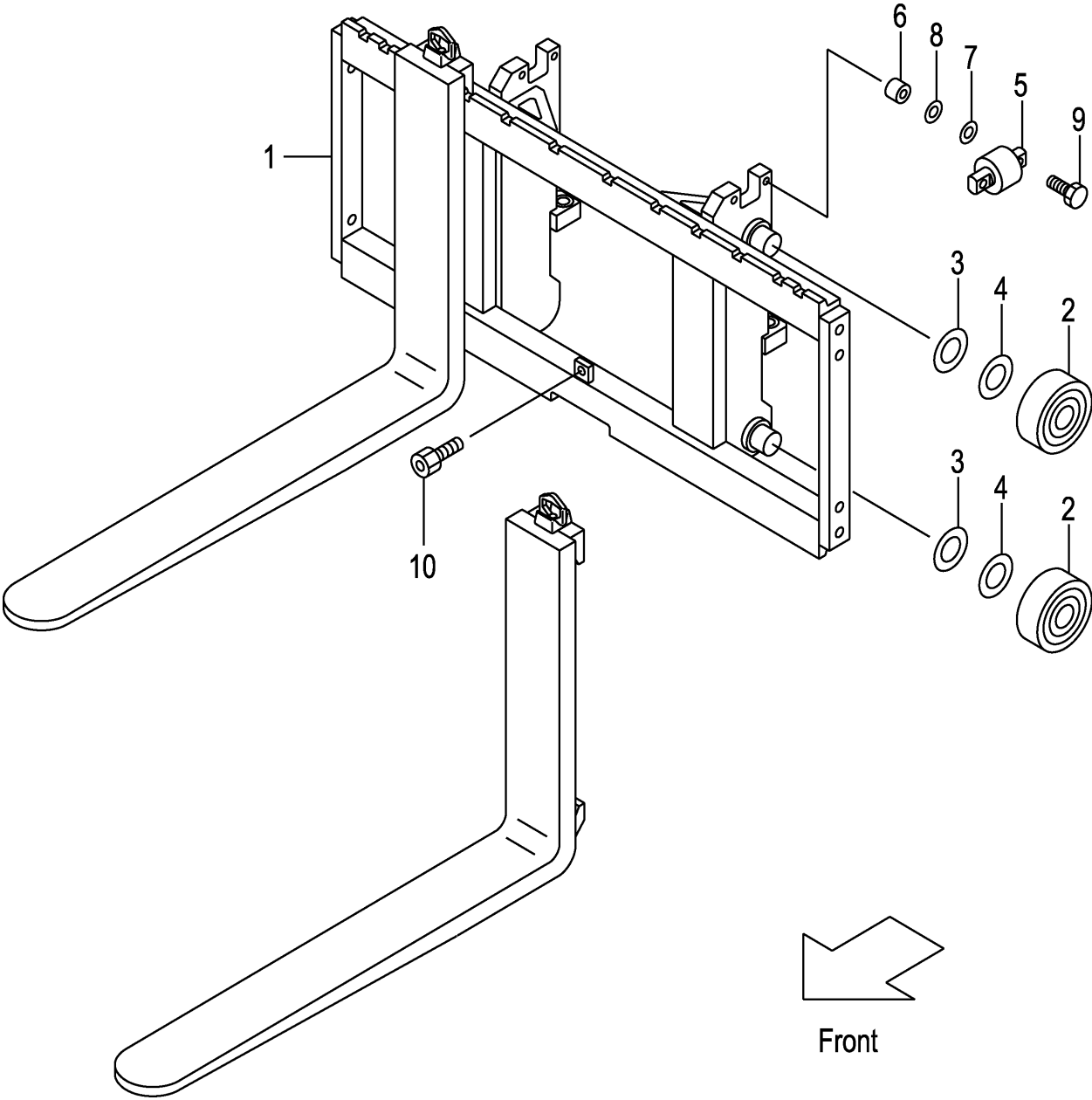
FIG.186 LIFT BRACKET [VM0A7,VM0A9] (M7018210) リフトブラケット
