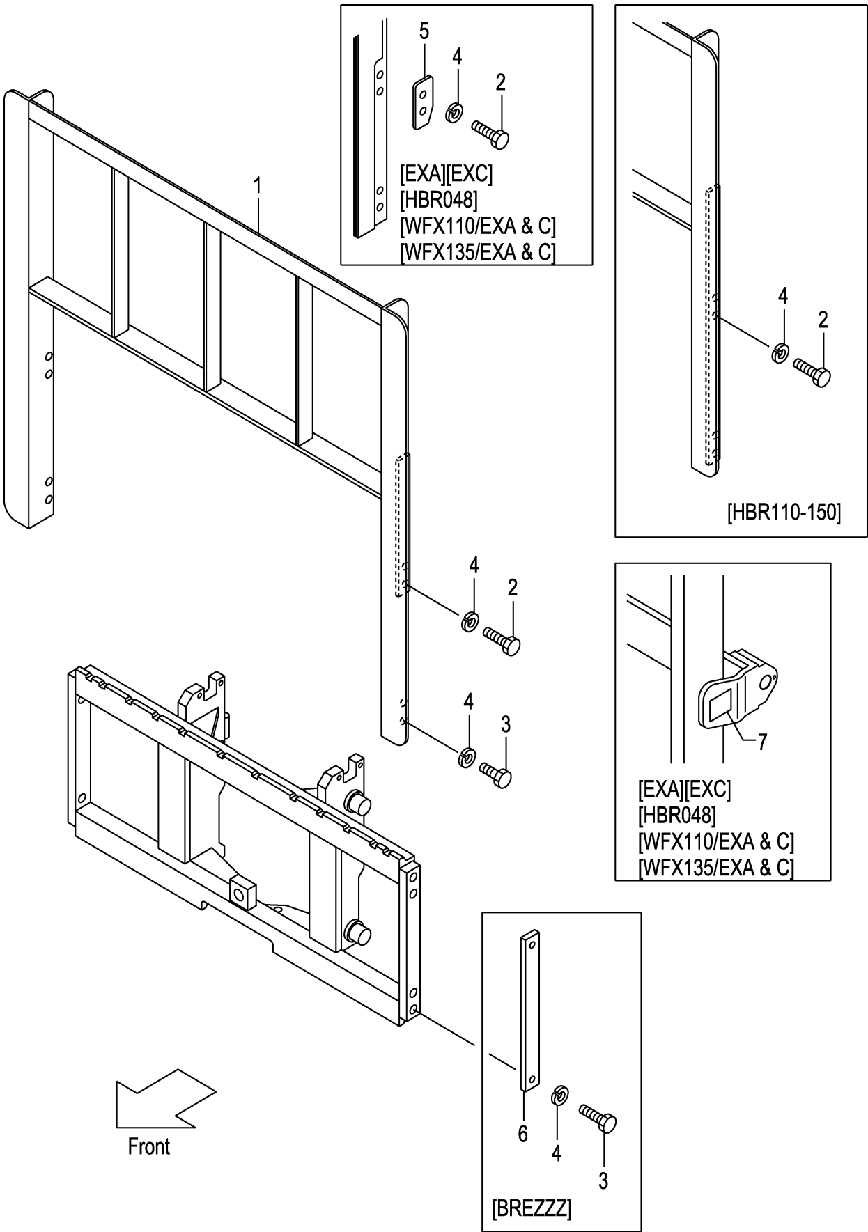
FIG.194 BACKREST [VFM0A7] (M7018230) バックレスト
