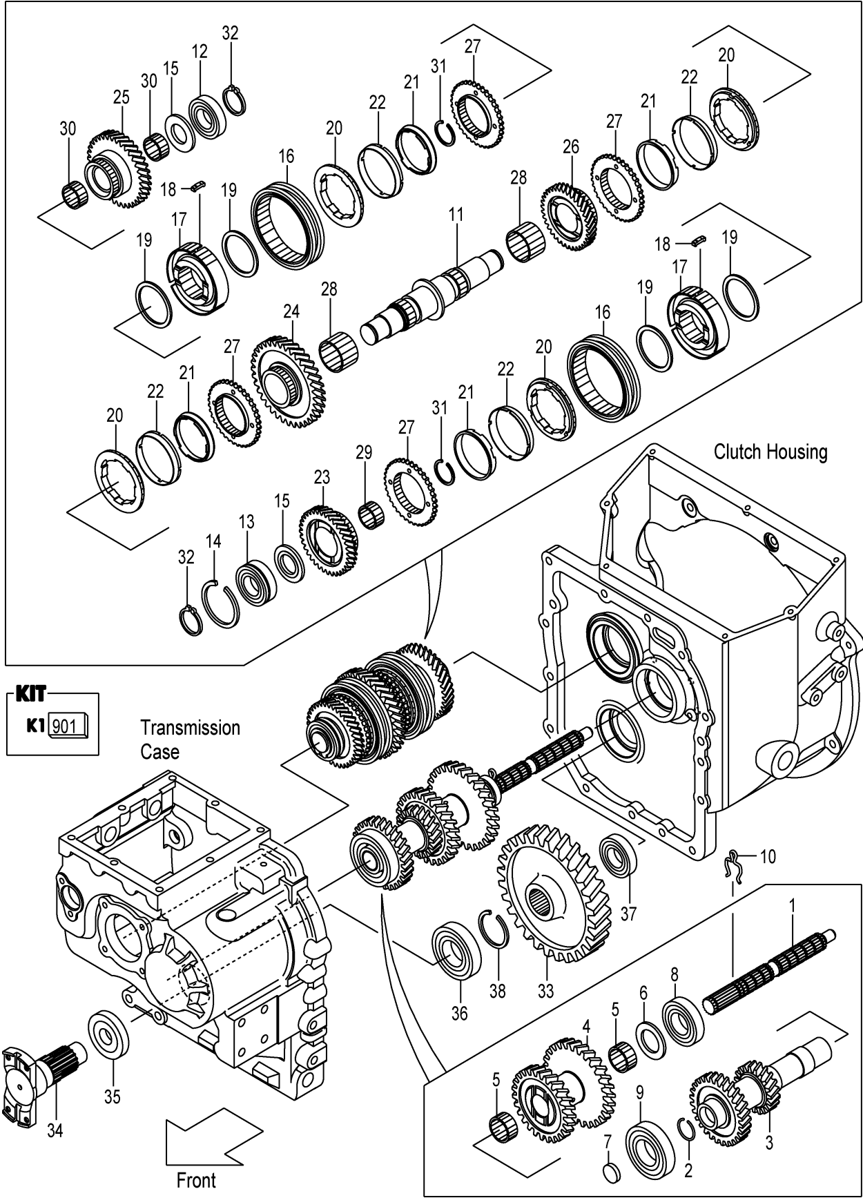
FIG.53 MISSION GEAR (CLUTCH) (F7Z12570) ミッションギヤー
