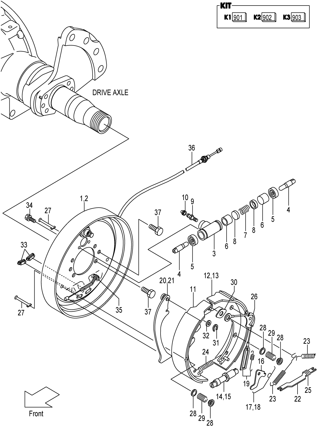
FIG.65 WHEEL BRAKE (F7Z13710) ホイールブレーキ
