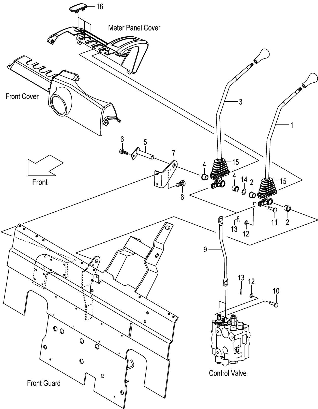
FIG.147 VALVE CONTROL (F7Z173A0) バルブコントロール
