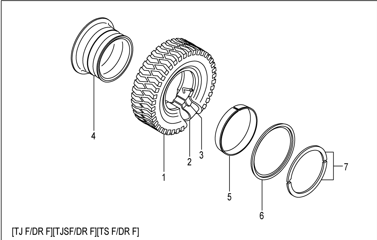
FIG.79 FRONT WHEEL (1.5T):[(TJ F,TJSF,TF,TS F)/DR F] (F7Z14480) フロントホイール
