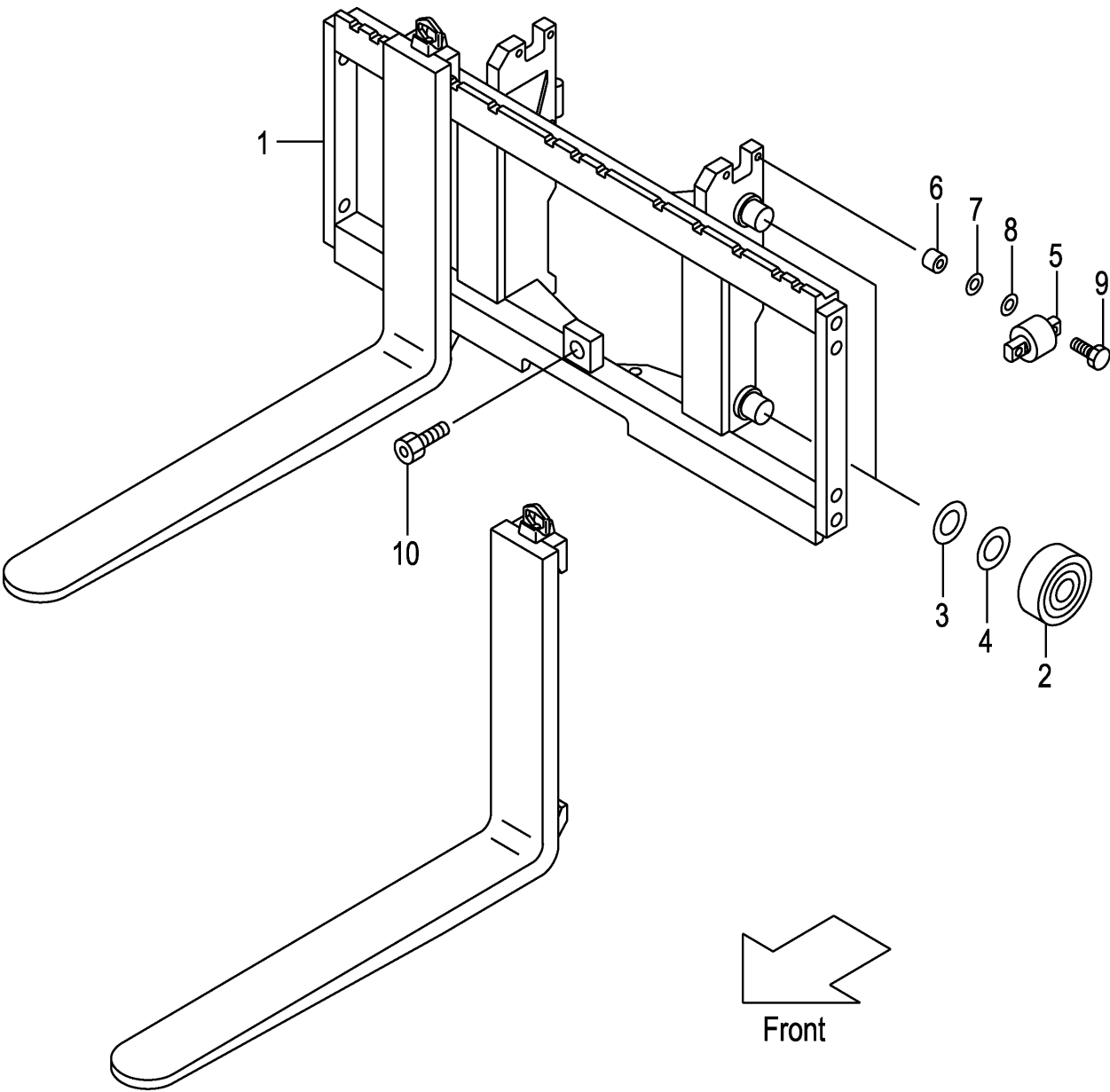
FIG.193 LIFT BRACKET [VFM0A7] (M7010610) リフトブラケット
