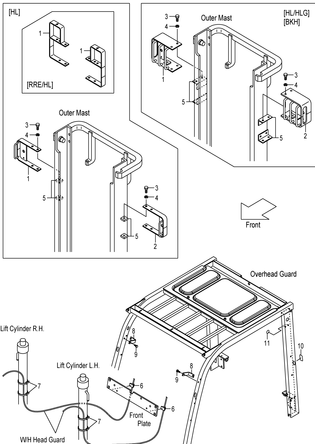
(F7Z15140) フロントランプブラケット
