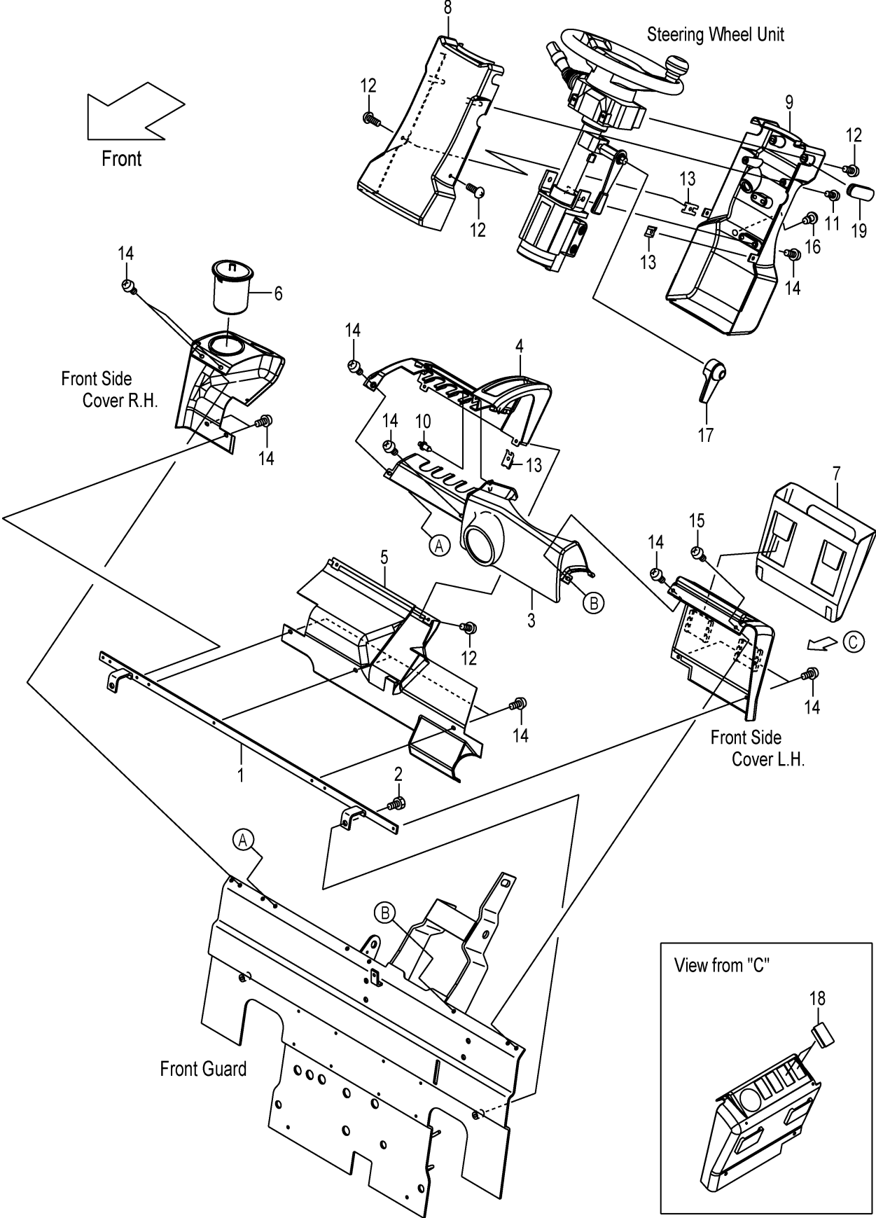
FIG.130 FRONT COVER (CLUTCH) (F7Z16470) フロントカバー
