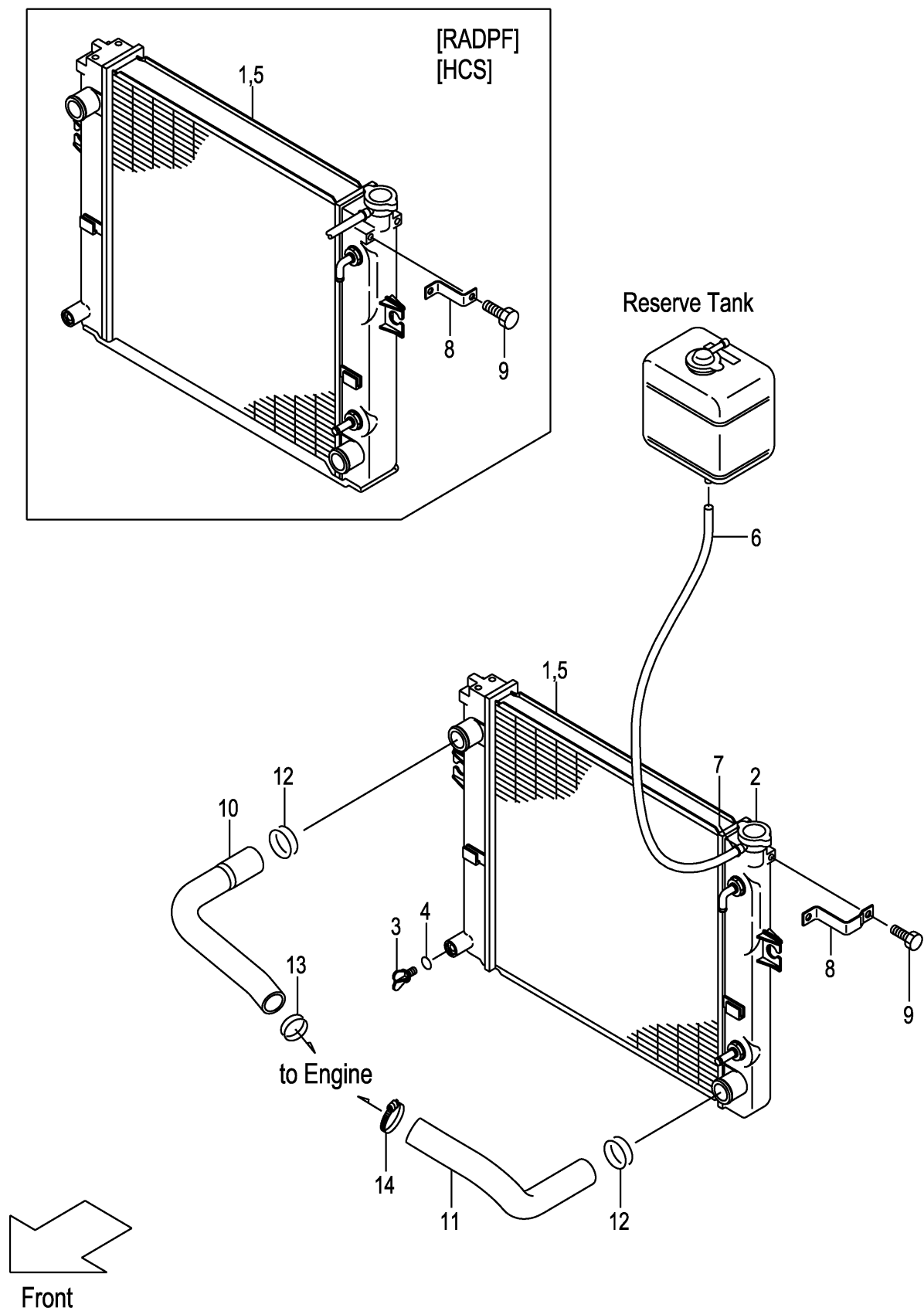
FIG.5 COOLING UNIT (F7Z12120) クーリングユニット
