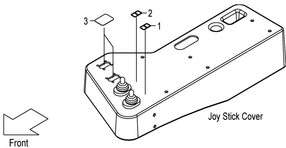
FIG.155 VALVE CONTROL KNOB (TOR-CON):[FIT] (F7Z173K0) バルブコントロールノブ
