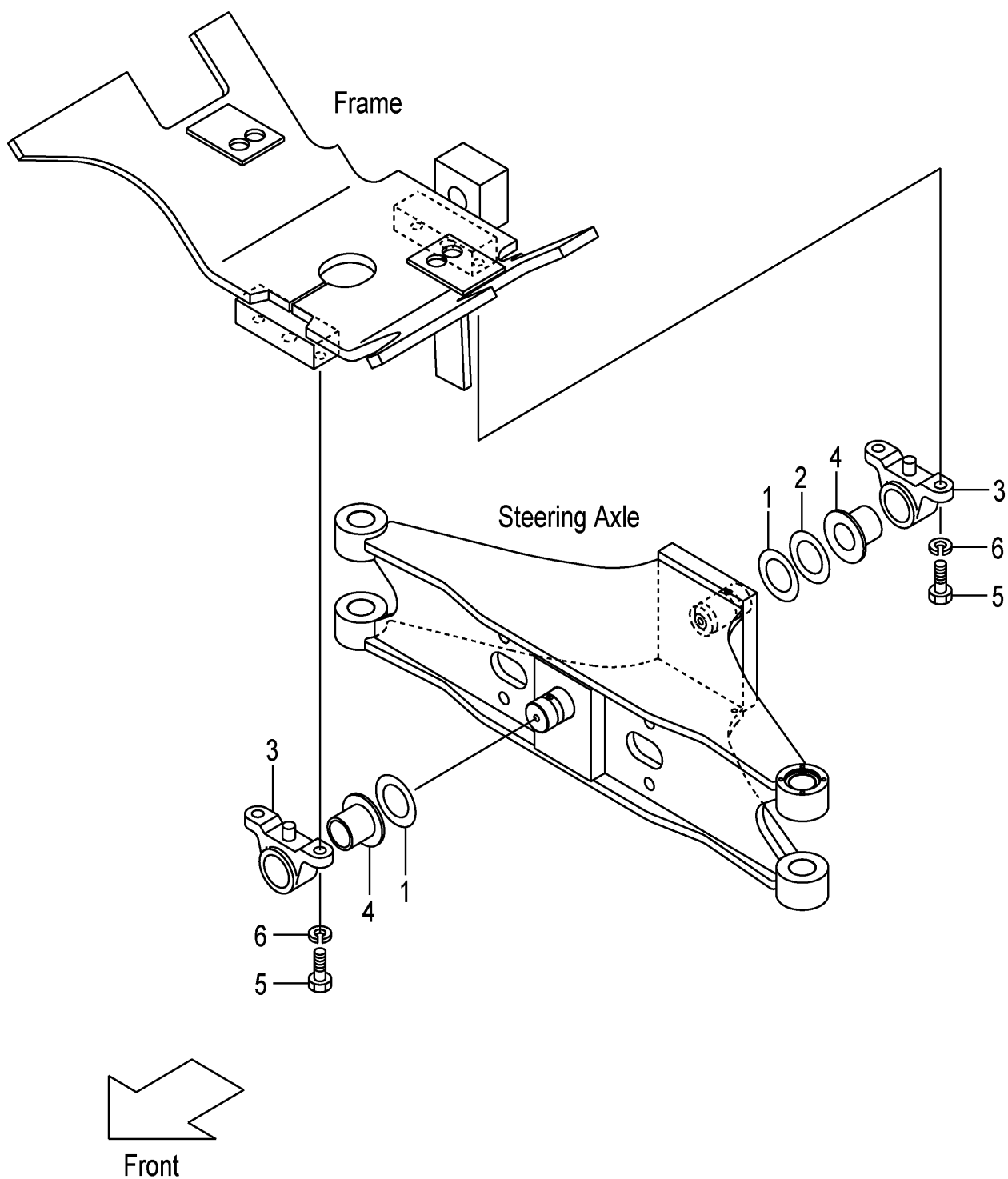
FIG.71 AXLE SUPPORT (F7Z14340) アクسلサポート
