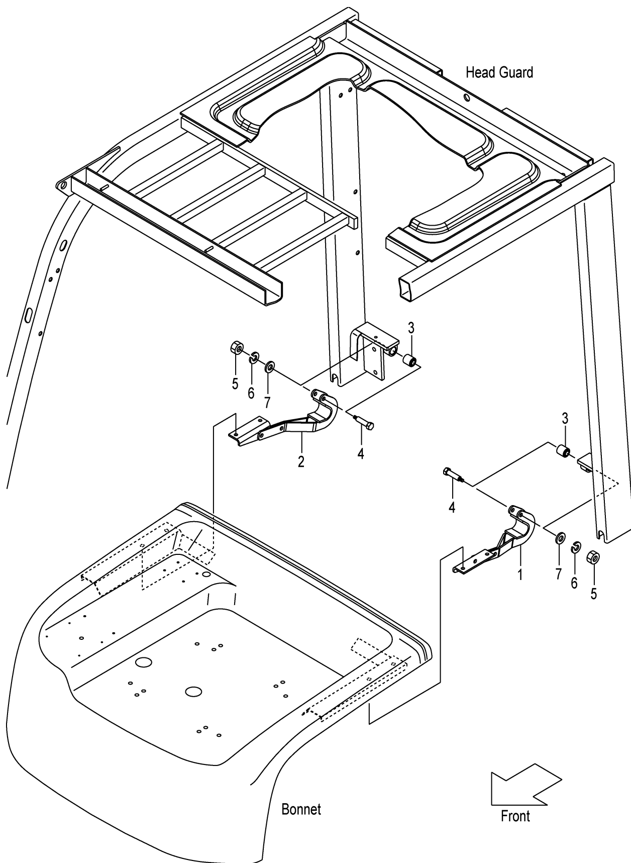
FIG.127 BONNET HINGE (F7Z16440) ホンネットヒンジ
