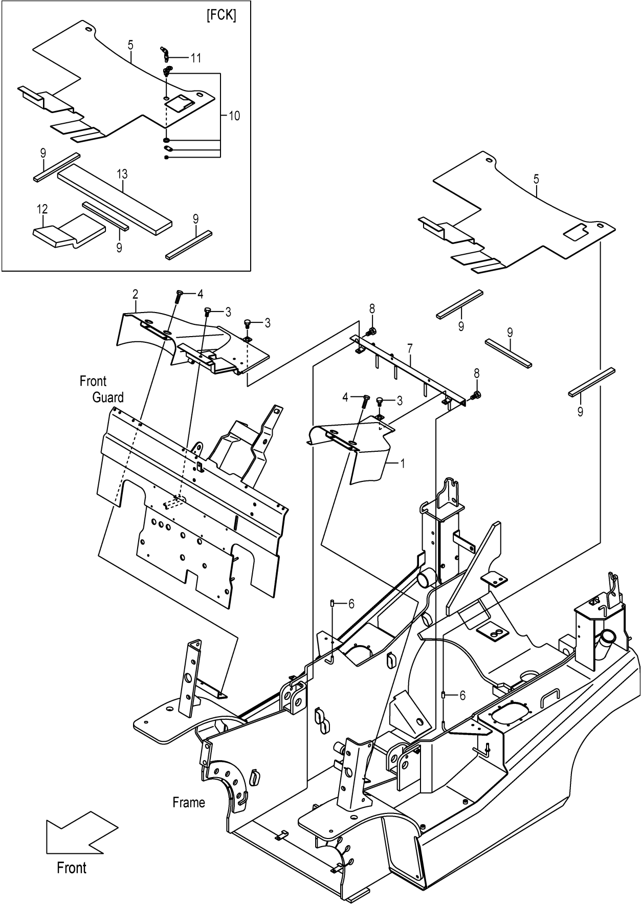
FIG.128 FLOOR BOARD (F7Z16450) フロアボード
