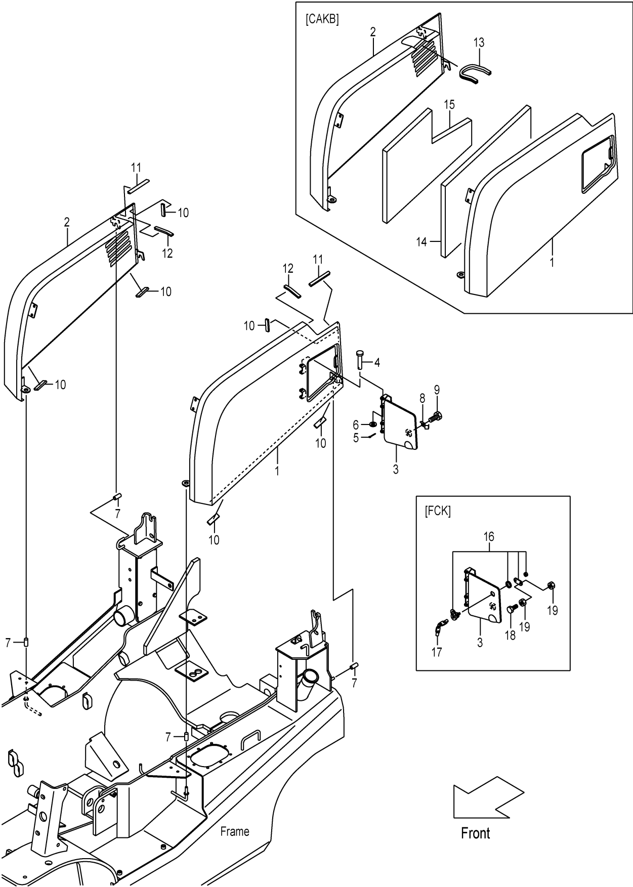
FIG.132 SIDE COVER (F7Z164A0) サイドカバー
