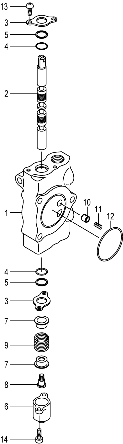
FIG.164 SPOOL SECTION (ATT)[4SV][5SV] (F7Z173Q0) スプールセクション
