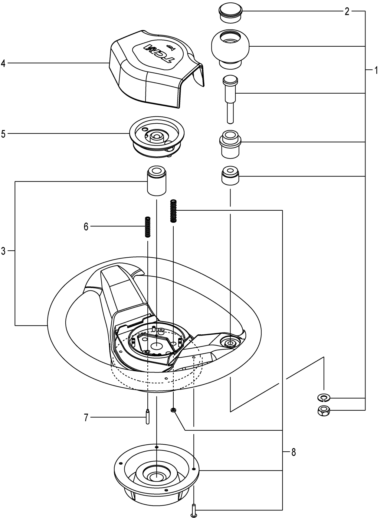
FIG.67 STEERING WHEEL (F7Z14120) ステアリングホイール
