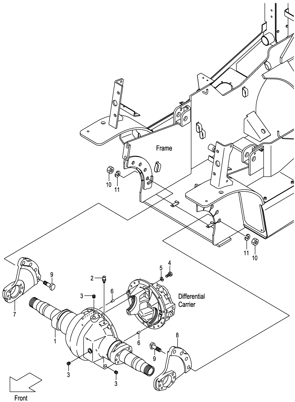
FIG.59 DRIVE AXLE (F7Z13010) ドライブ・アクスル
