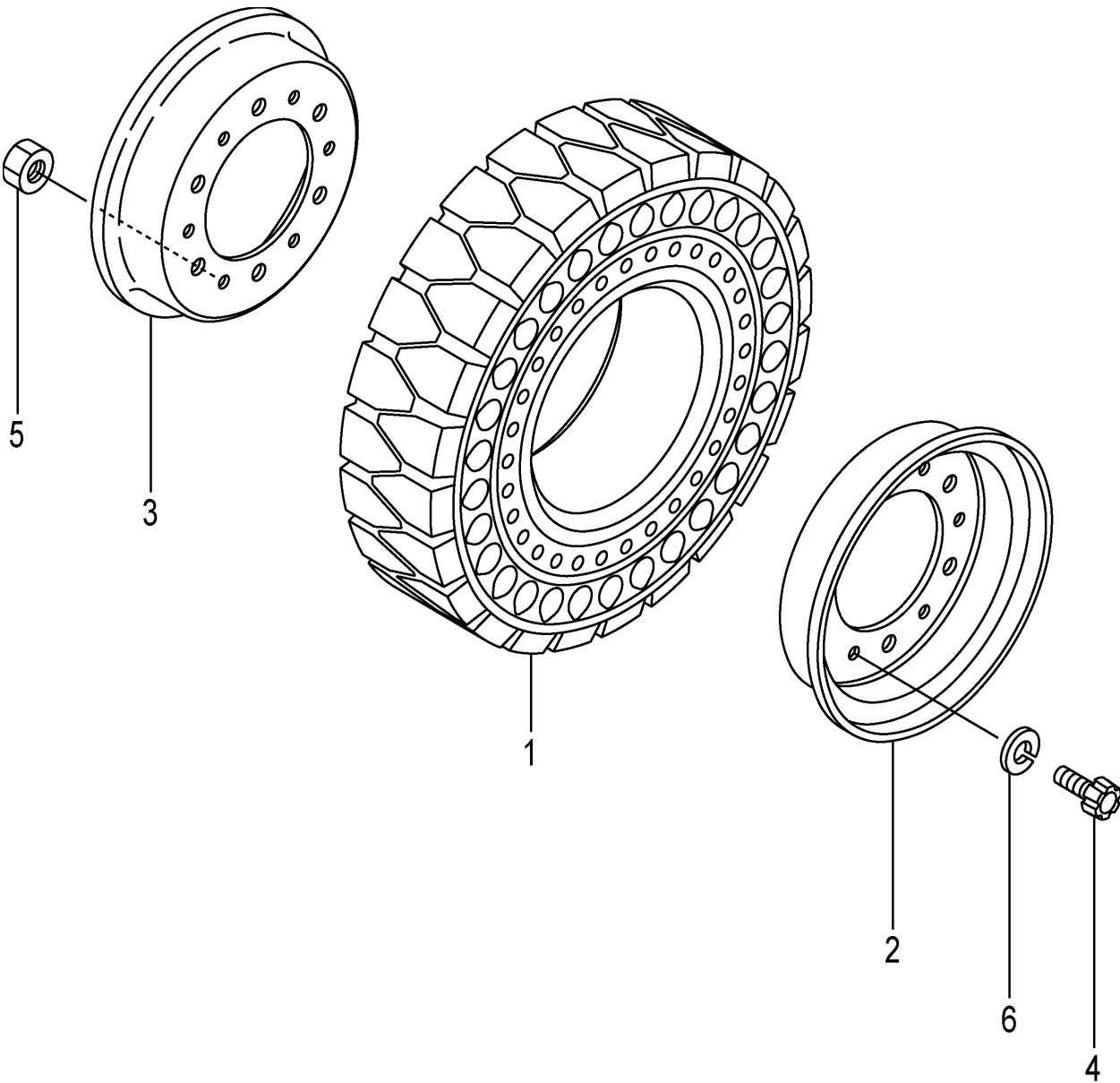
FIG.83 FRONT WHEEL (1.5T):[TRAF] (F7Z144C0) フロントホイール
