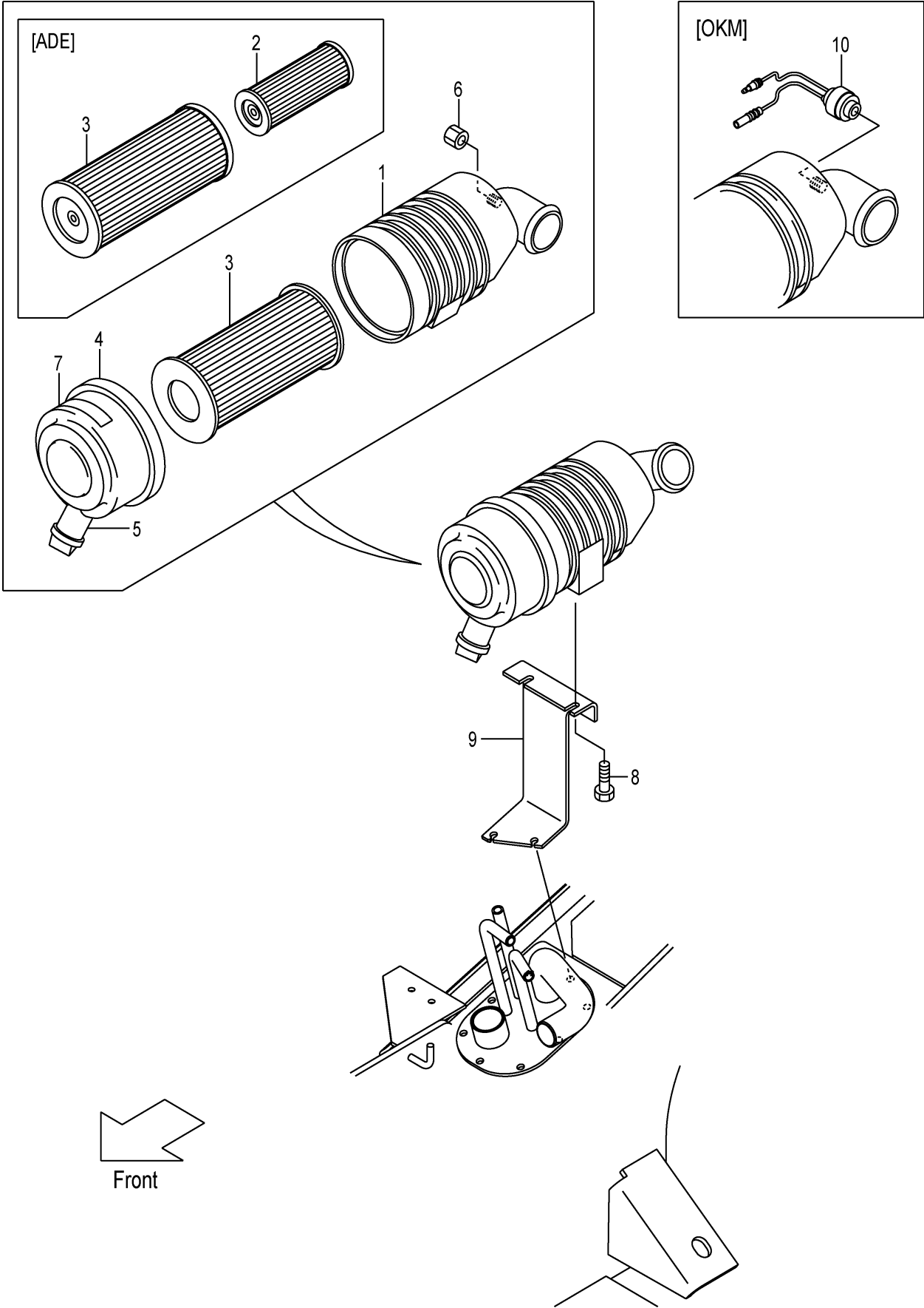
FIG.2 AIR CLEANER (F7Z11040) エアークリーナ
