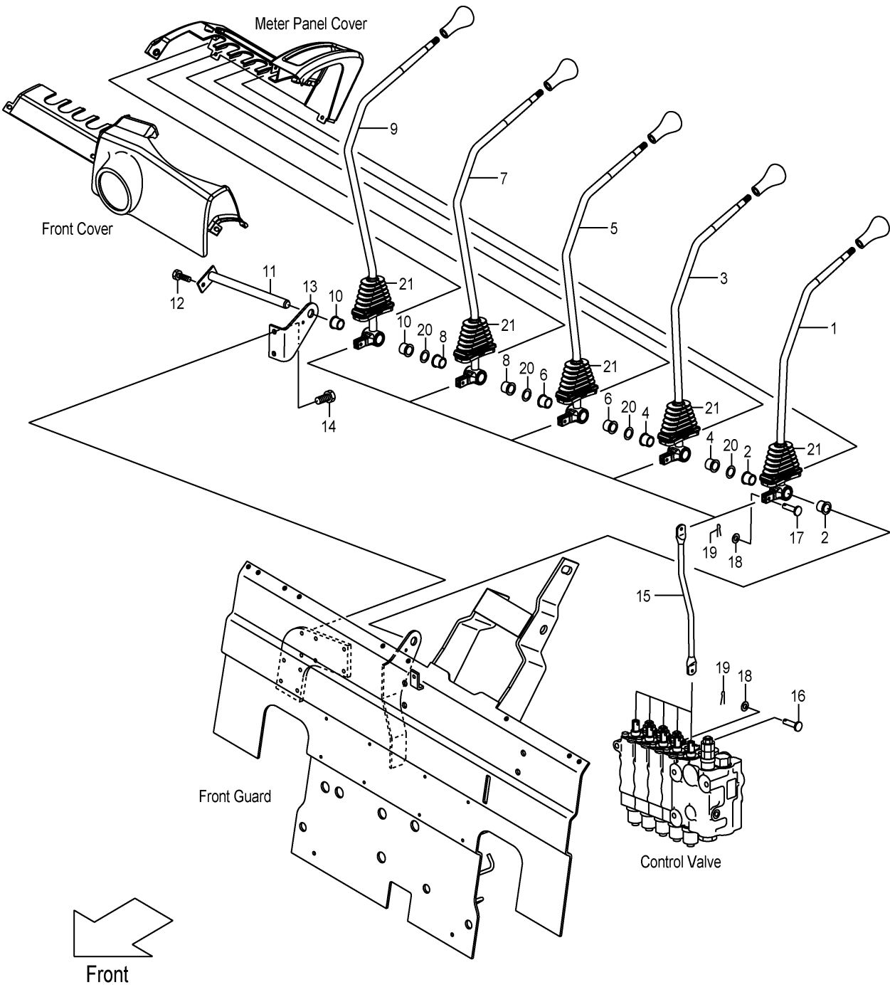
FIG.150 VALVE CONTROL [5SV] (F7Z173D0) バルブコントロール
