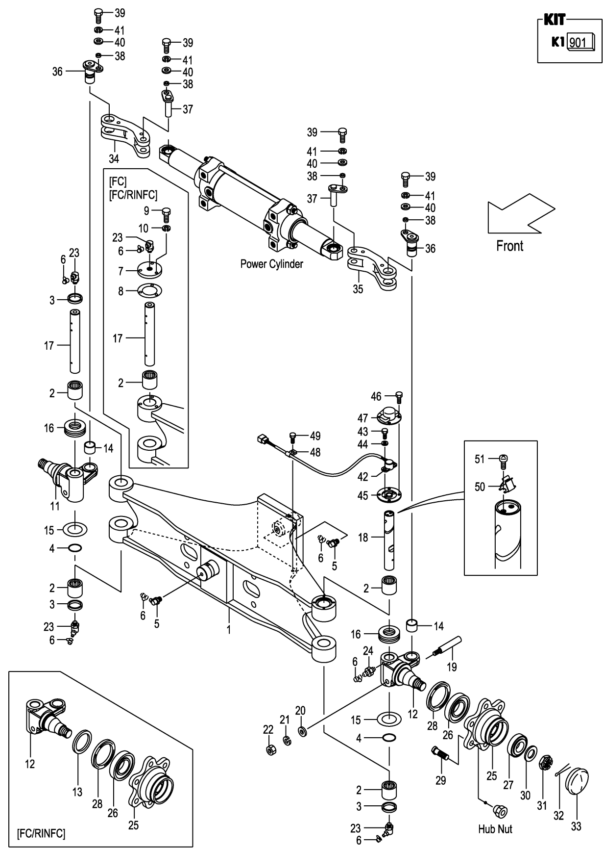
FIG.70 STEERING AXLE (F7Z14310) ステアリングアクスル
