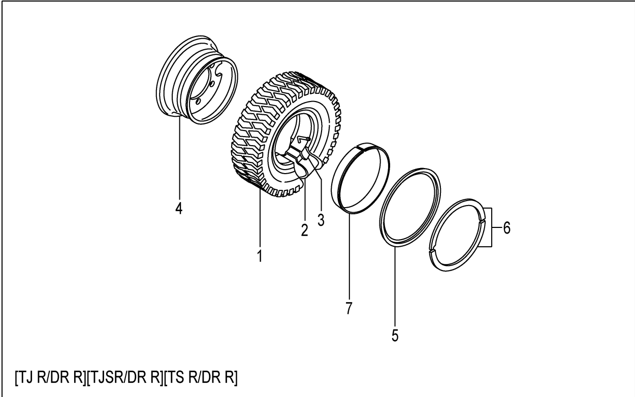
FIG.92 REAR WHEEL [(TJ R,TJSR,TR,TS R)/DR R] (F7Z144M0) リヤホイール
