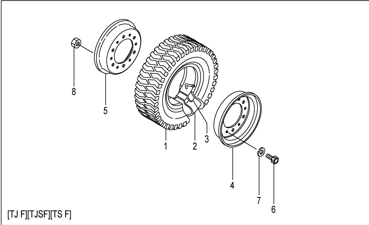
FIG.77 FRONT WHEEL (1.5T):[TJ F][TJSF][TF][TS F] (F7Z14460) フロントホイール
