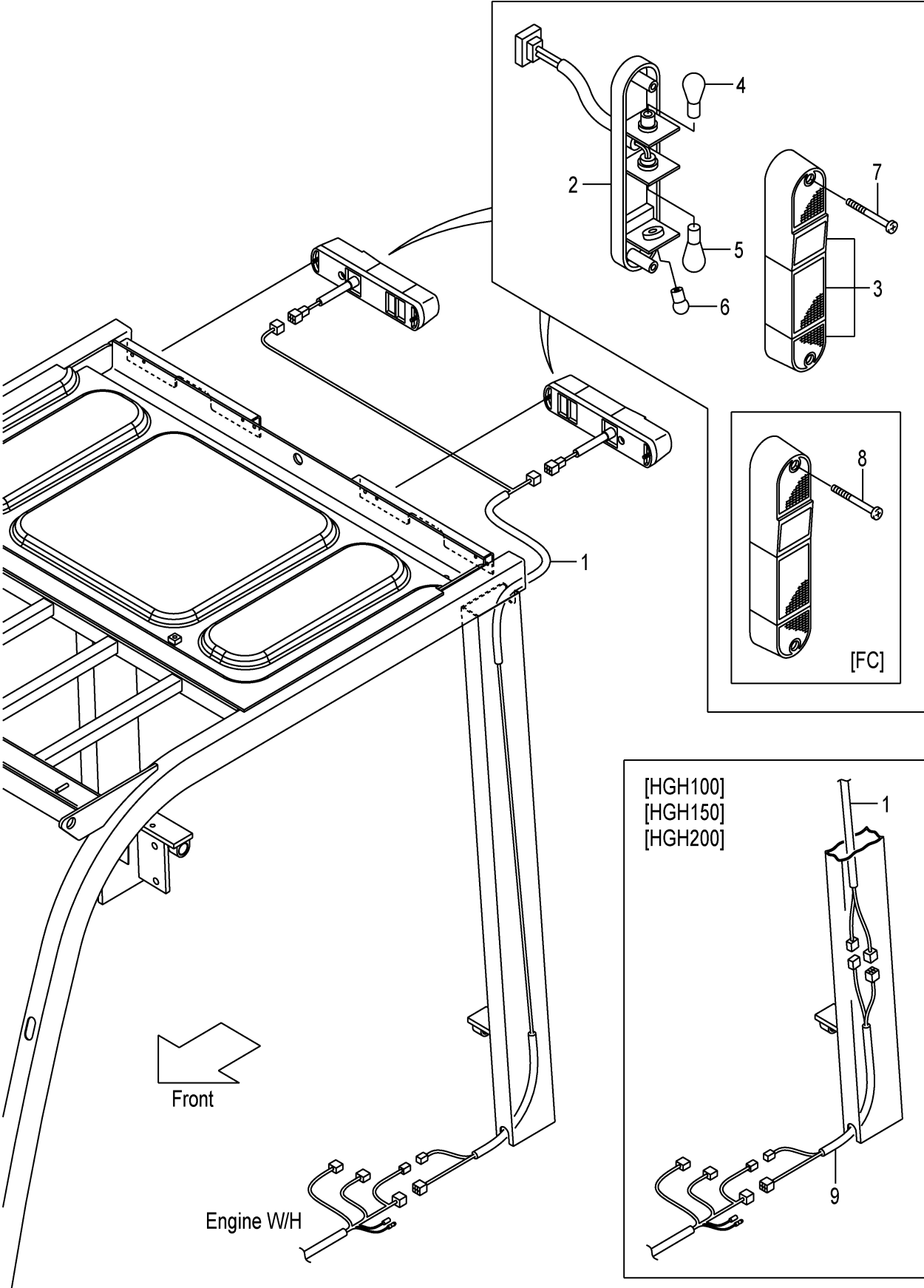
FIG.21 REAR COMBINATION LAMP (F7Z124H0) リヤコンビネーションランプ
