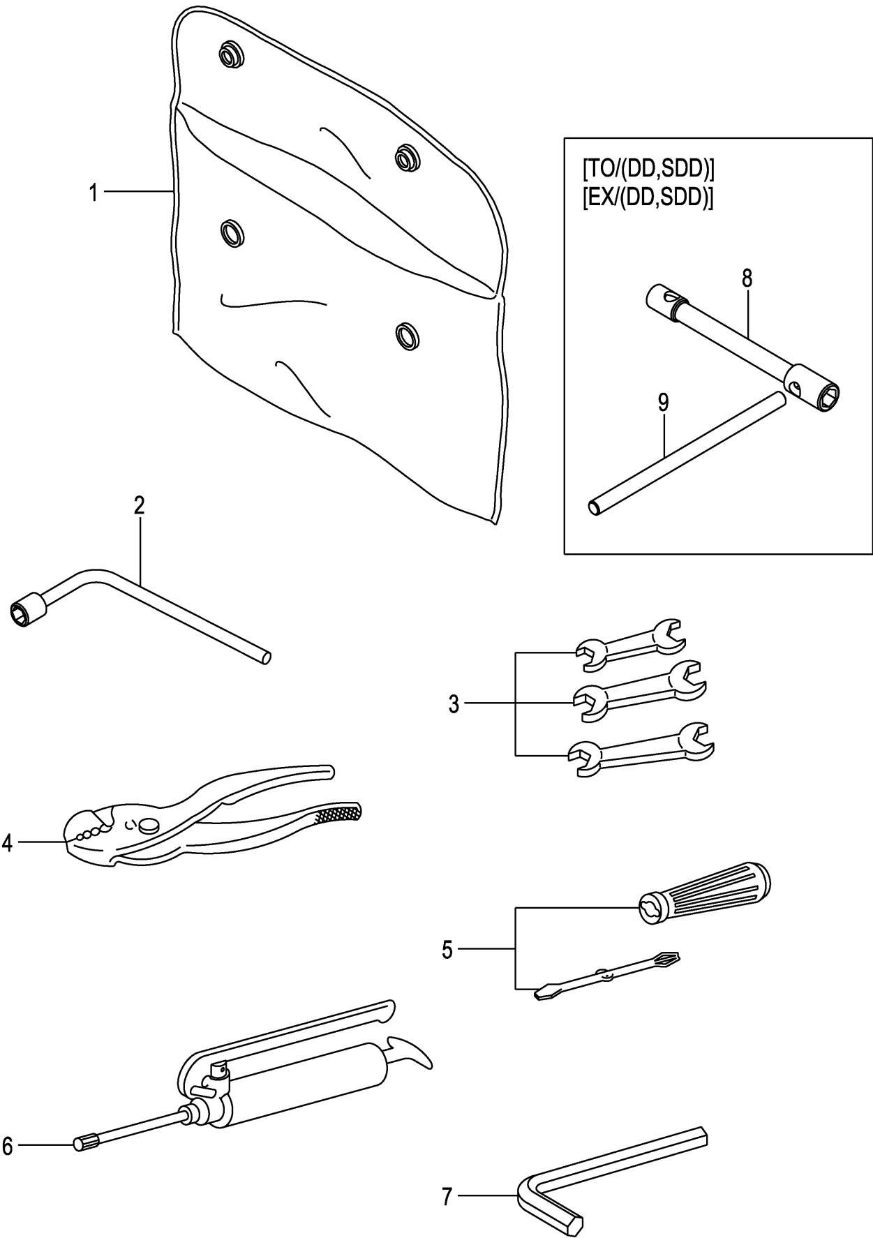
FIG.177 SERVICE TOOL [TO][EX] (F7Z19210) サービスツール
