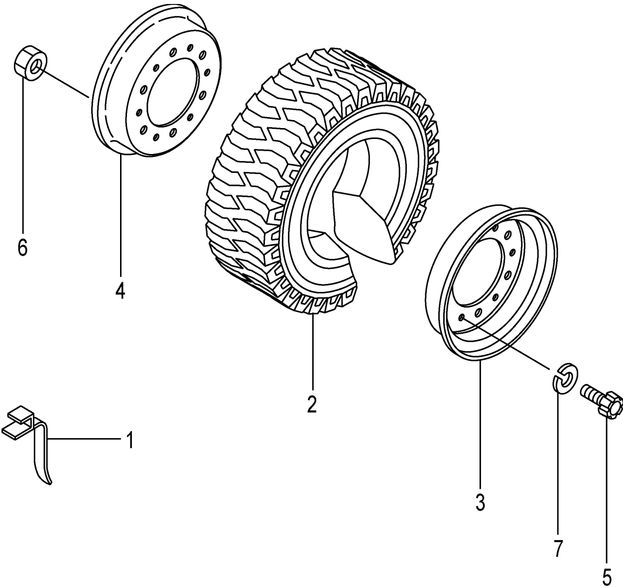
FIG.93 REAR WHEEL [TSUR][TUJR][TUSR][TUWR][TUGR] (F7Z144N0) リヤホイール
