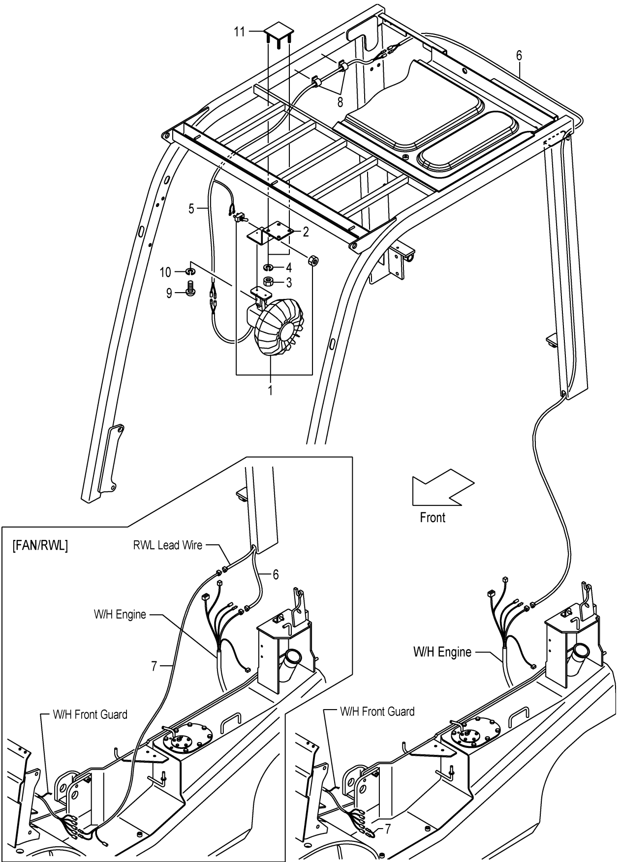
FIG.35 FAN [FAN] (F7Z12650) ファン
