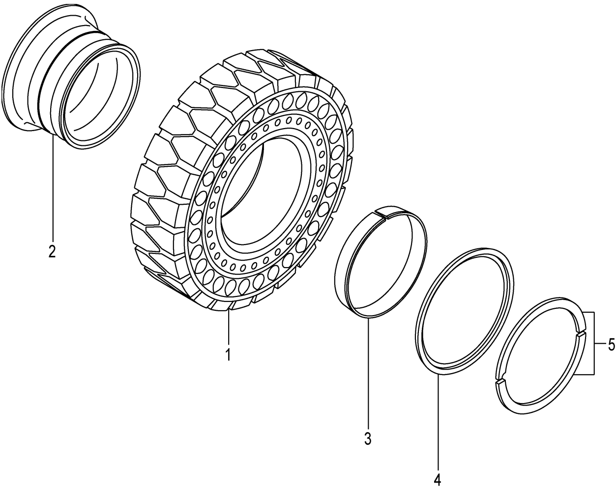
FIG.84 FRONT WHEEL (1.8T):[TRAF] (F7Z144D0) フロントホイール
