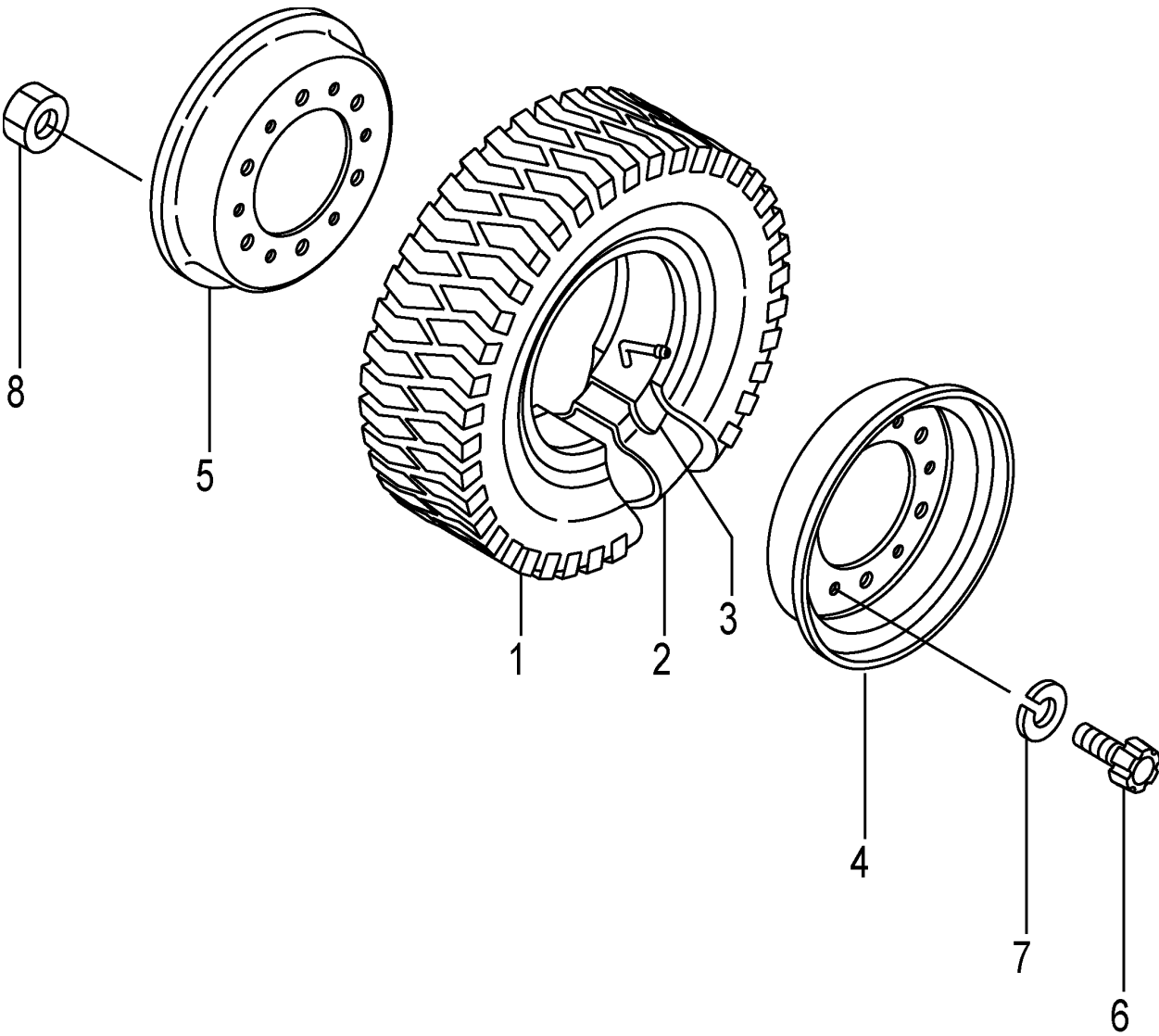
FIG.89 REAR WHEEL (F7Z144J0) リヤホイール
