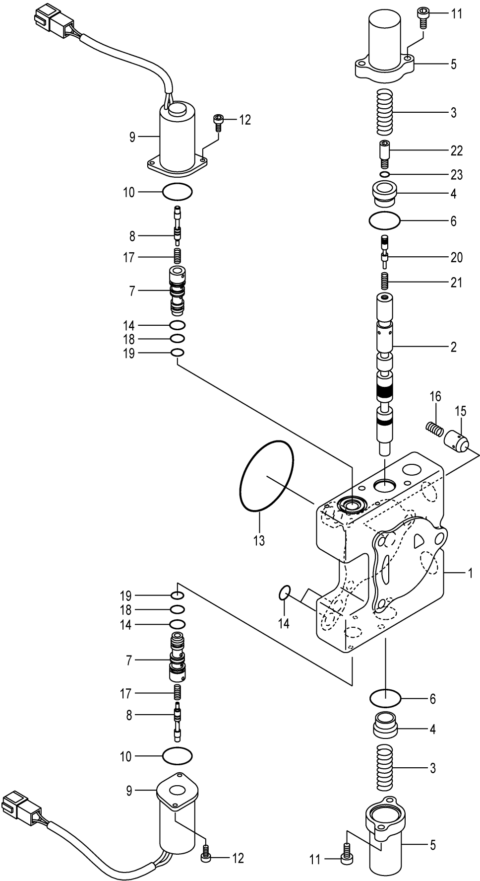
FIG.161 SPOOL SECTION (TILT)(TOR-CON):[FIT] (F7Z173T0) スプールセクション
