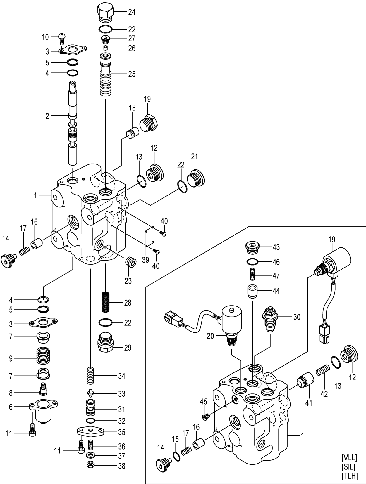
FIG.157 SPOOL SECTION (LIFT) (F7Z173M0) スプールセクション
