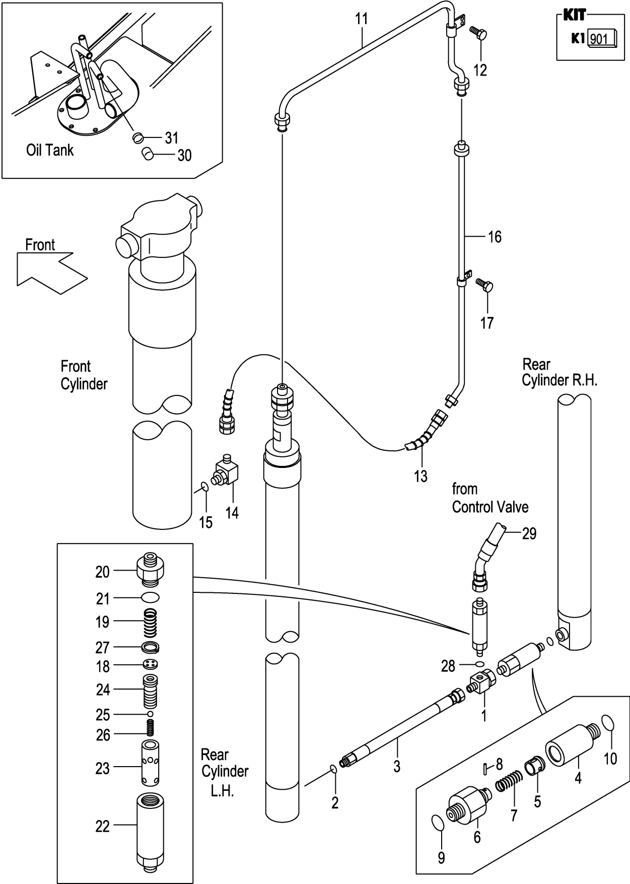
FIG.198 MAST PIPING [VFM0A7] (M7010530) マストパイピング
