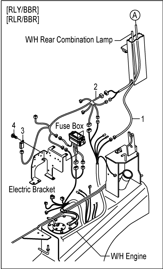
FIG.30 REVOLVING LIGHT WIRE HARNESS [RLY][RLR] (F7Z124W0) リボルビングライトワイヤハーネス
