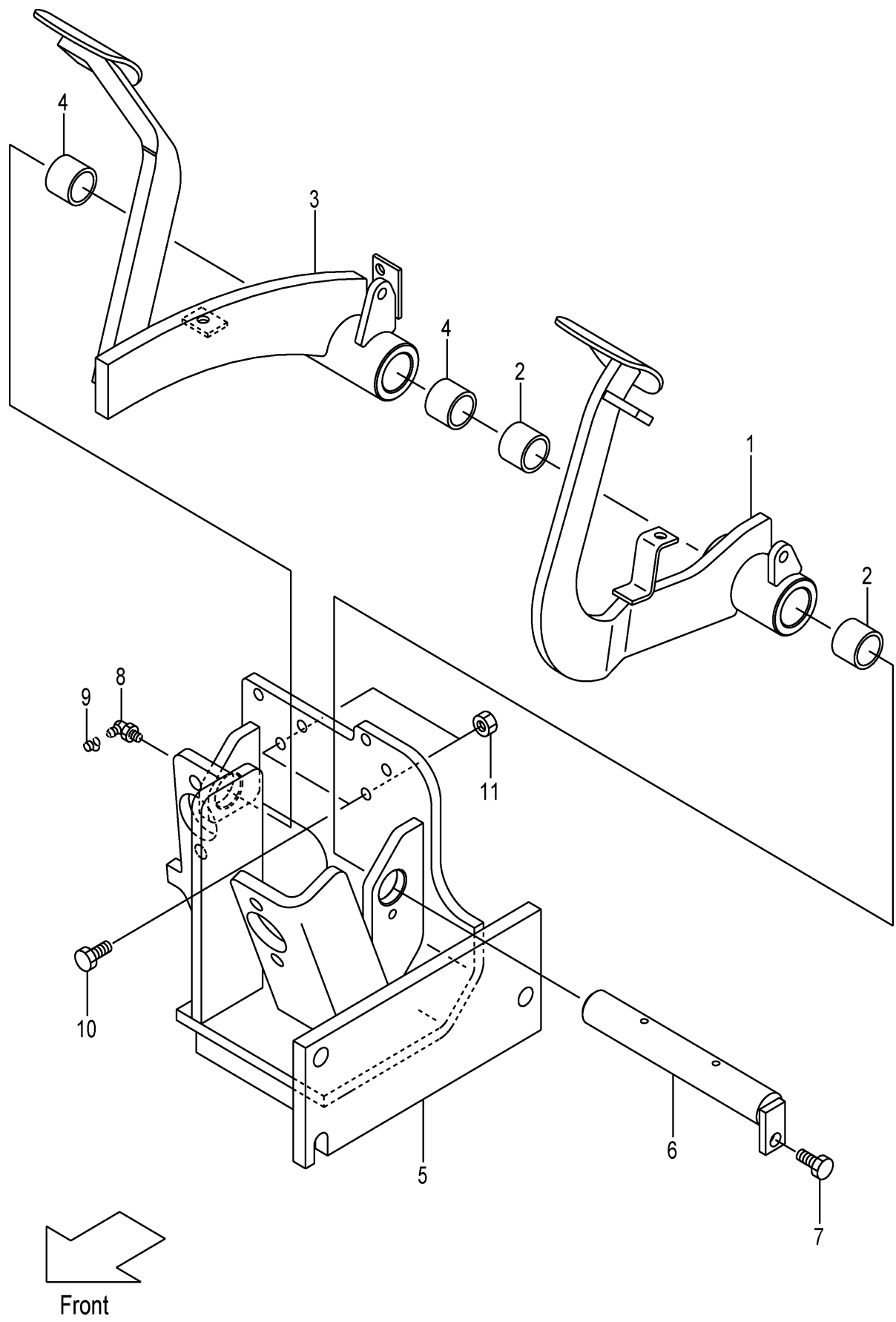
FIG.107 FOOT PEDAL (CLUTCH) (F7Z15410) フットペダル
