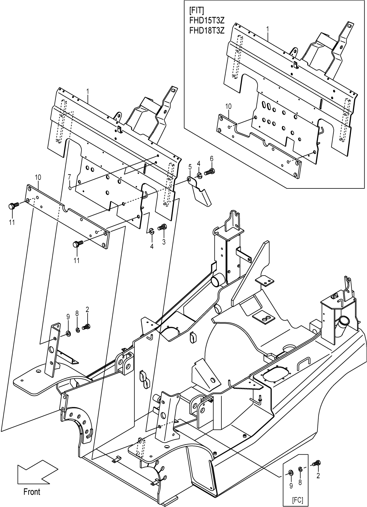
FIG.124 FRONT GUARD (F7Z16410) フロントガード
