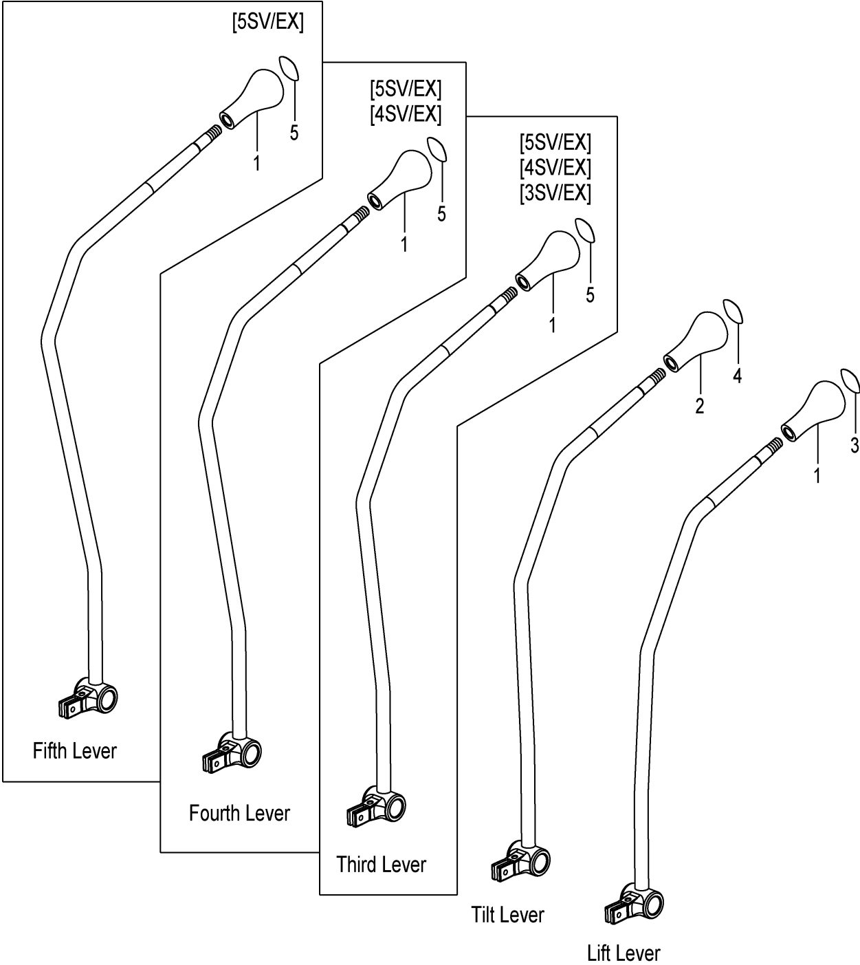
FIG.154 VALVE CONTROL KNOB (F7Z173J0) バルブコントロールノブ
