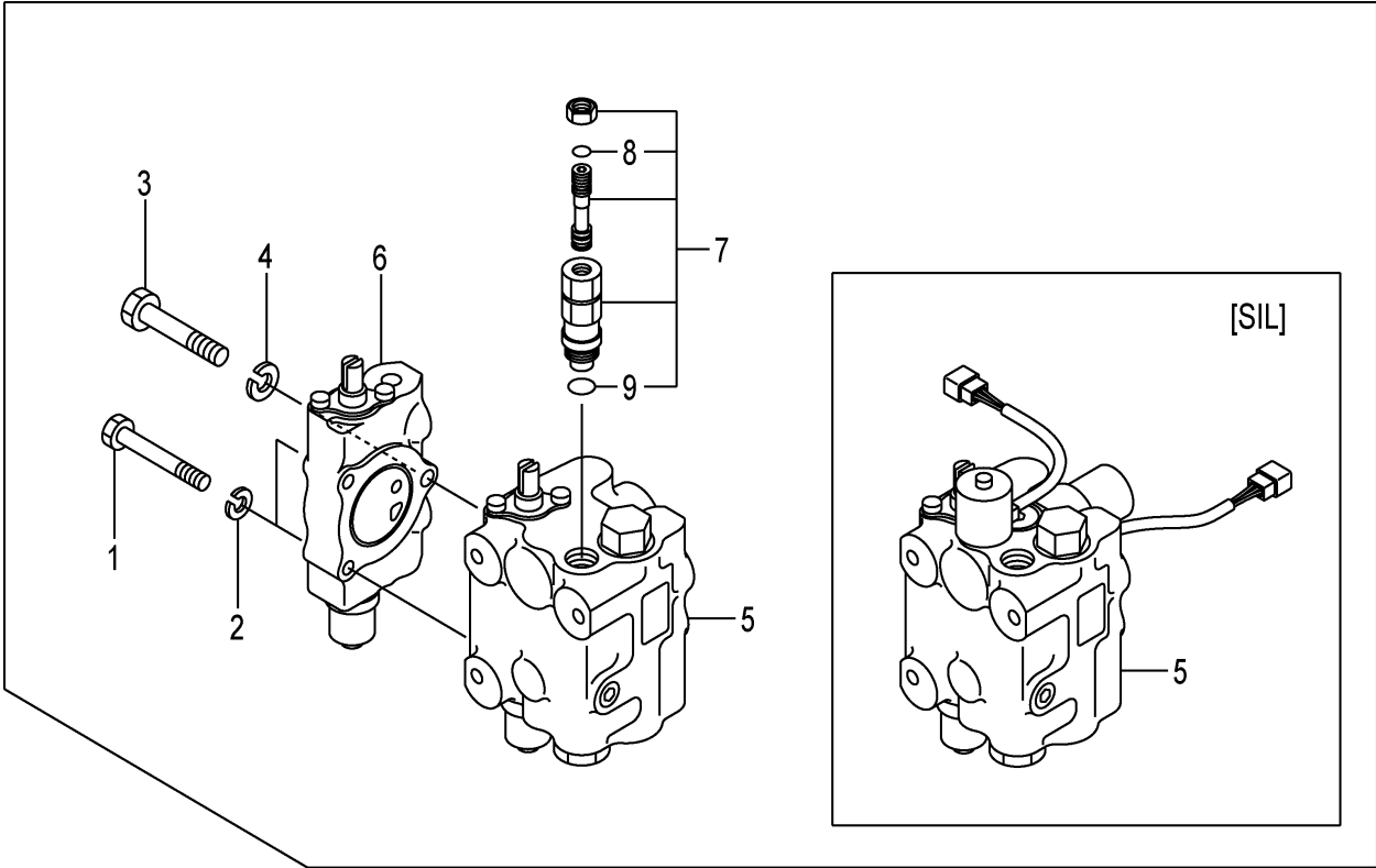
FIG.139 CONTROL VALVE (F7Z17310) コントロールバルブ
