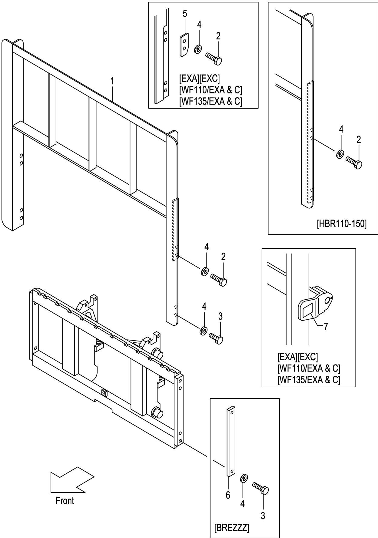
FIG.187 BACKREST [VM0A7,VM0A9] (M7018220) バックレスト
