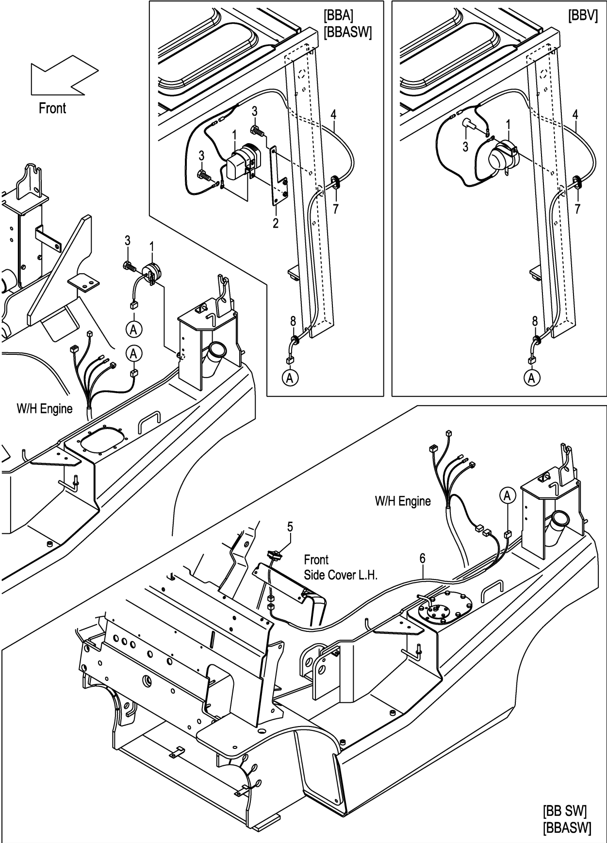
FIG.32 BACK BUZZER (F7Z124X0) バックブザー
