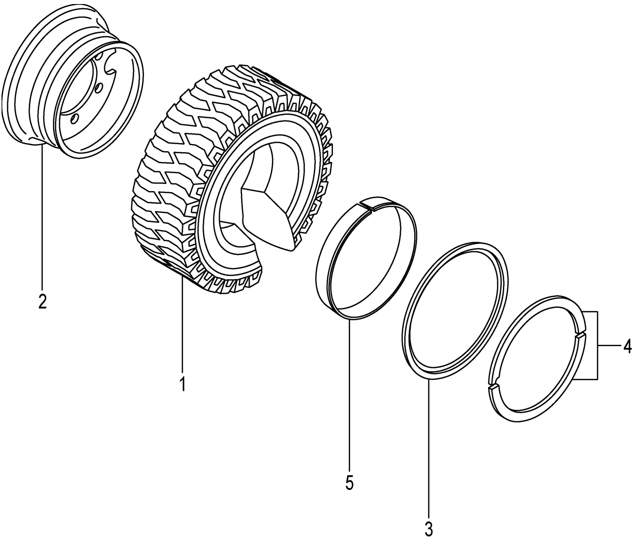
FIG.94 REAR WHEEL [TUJR/DR R] (F7Z144P0) リヤーホイール
