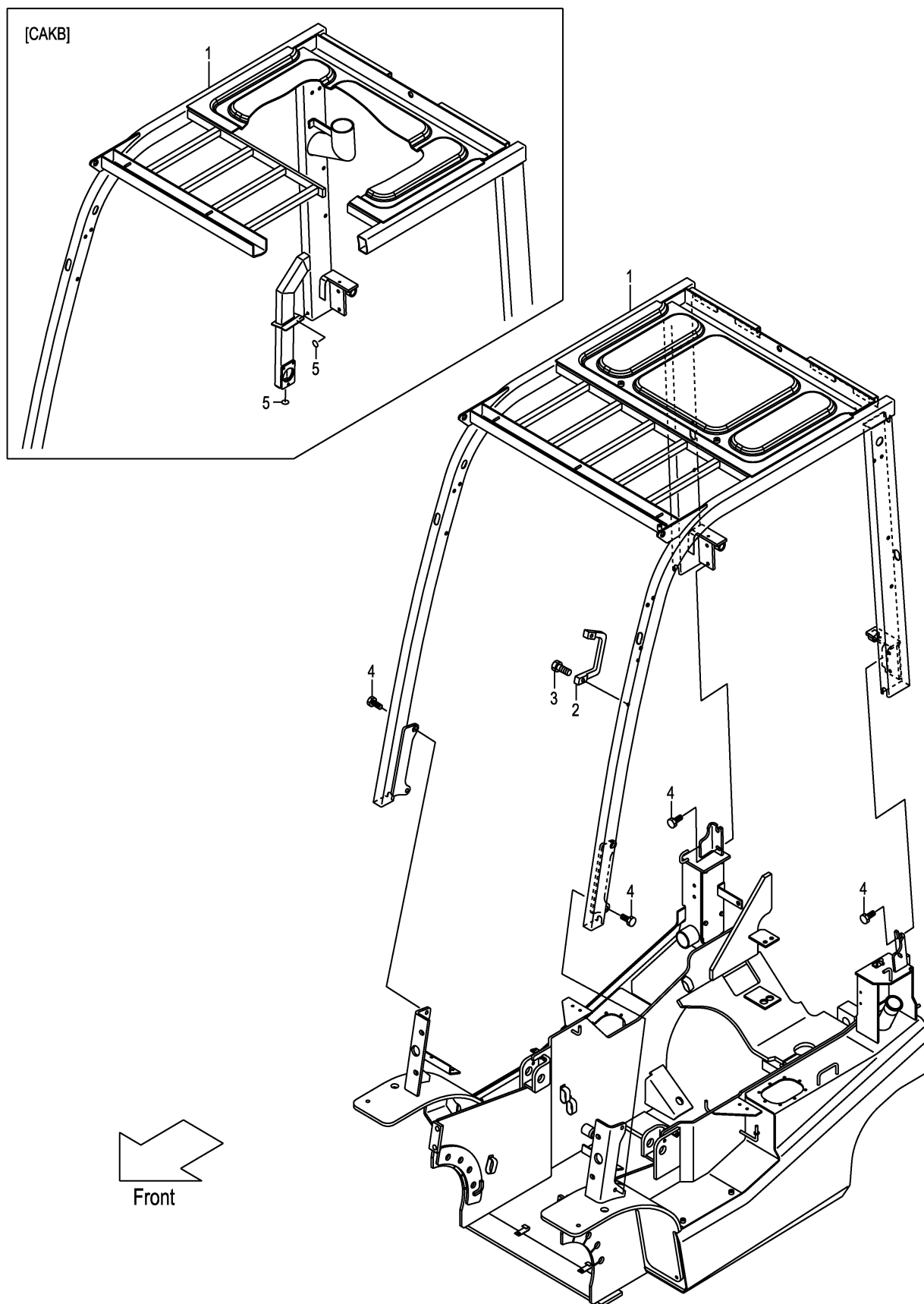
FIG.98 OVERHEAD GUARD (F7Z15110) オーバヘッドガード
