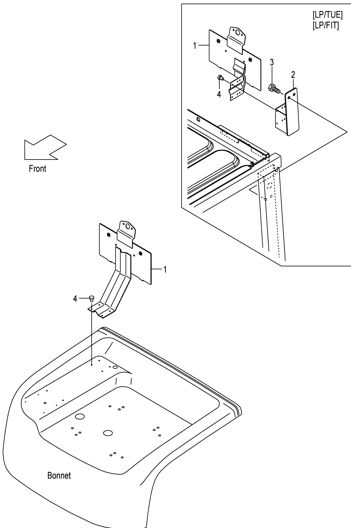
FIG.22 LICENSE LAMP [LP] (F7Z124N0) ライセンスランプ°
