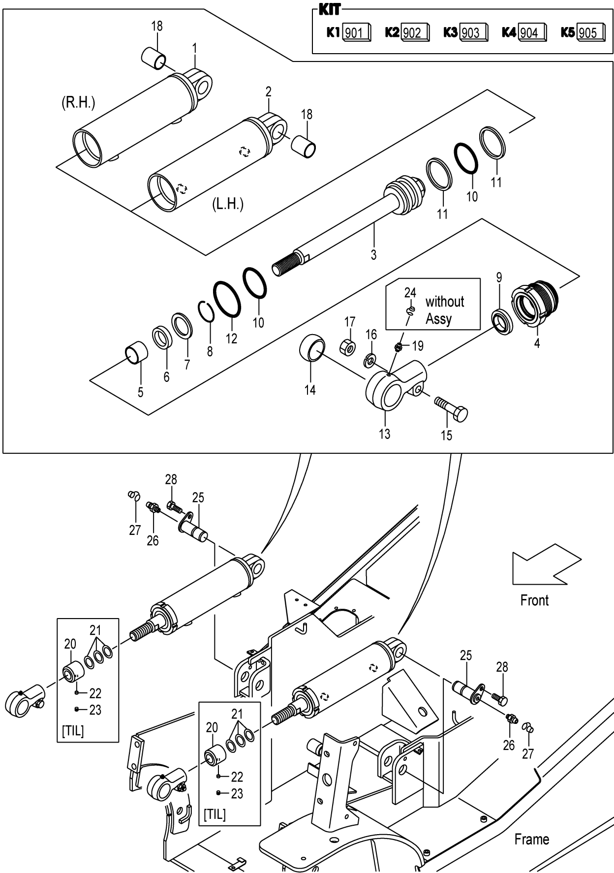
FIG.172 TILT CYLINDER (F7Z18510) ティルトシリンダ
