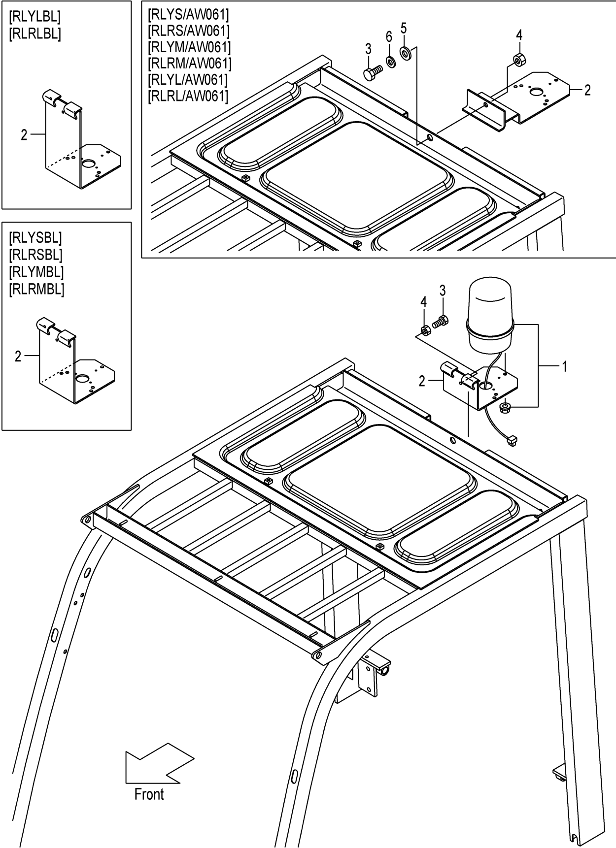
FIG.29 REVOLVING LIGHT [RLY][RLR] (F7Z124V0) リボルビングライト
