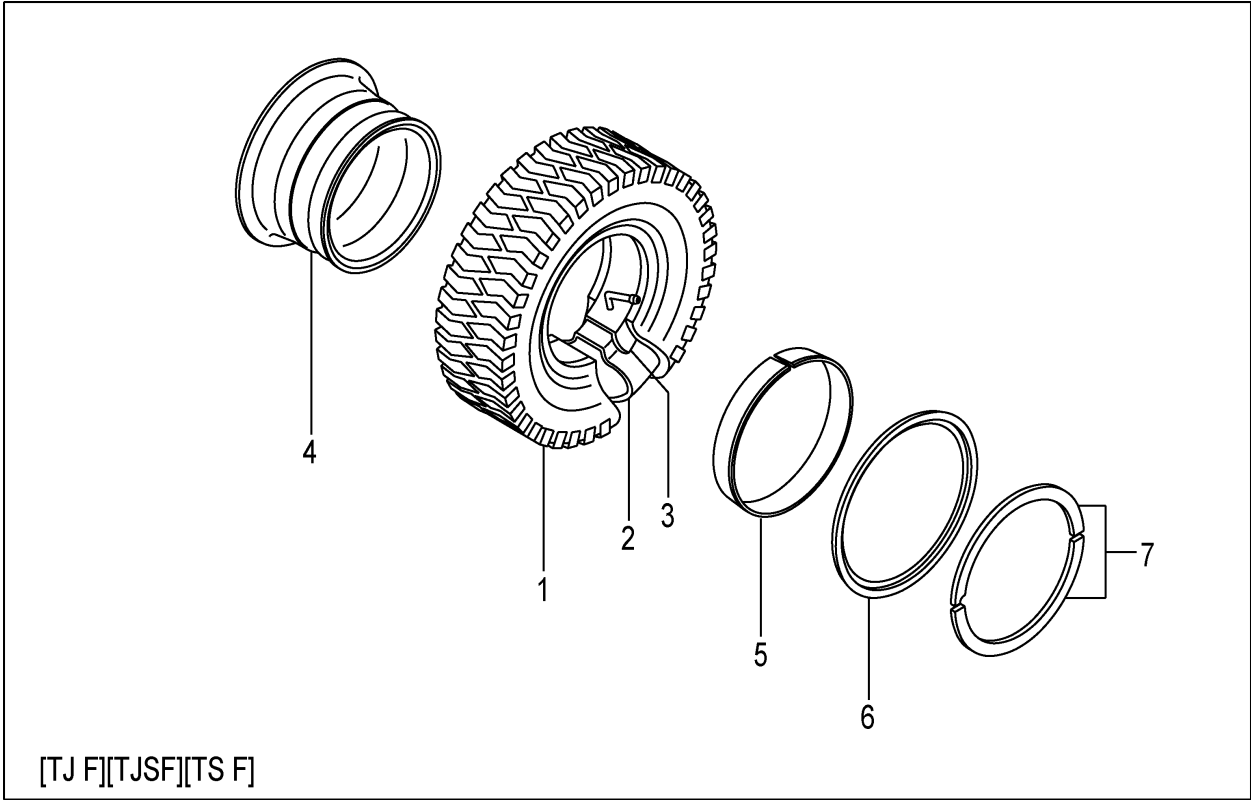
FIG.78 FRONT WHEEL (1.8T):[TJ F][TJSF][TF][TS F] (F7Z14470) フロントホイール
