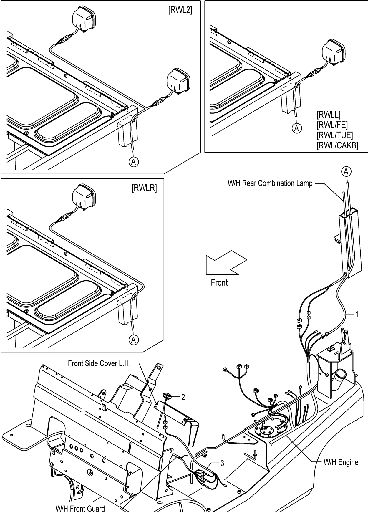
FIG.27 REAR WORKING LIGHT WIRE HARNESS [RWL] (F7Z124T0) リヤワーキングライトワイヤハーネス
