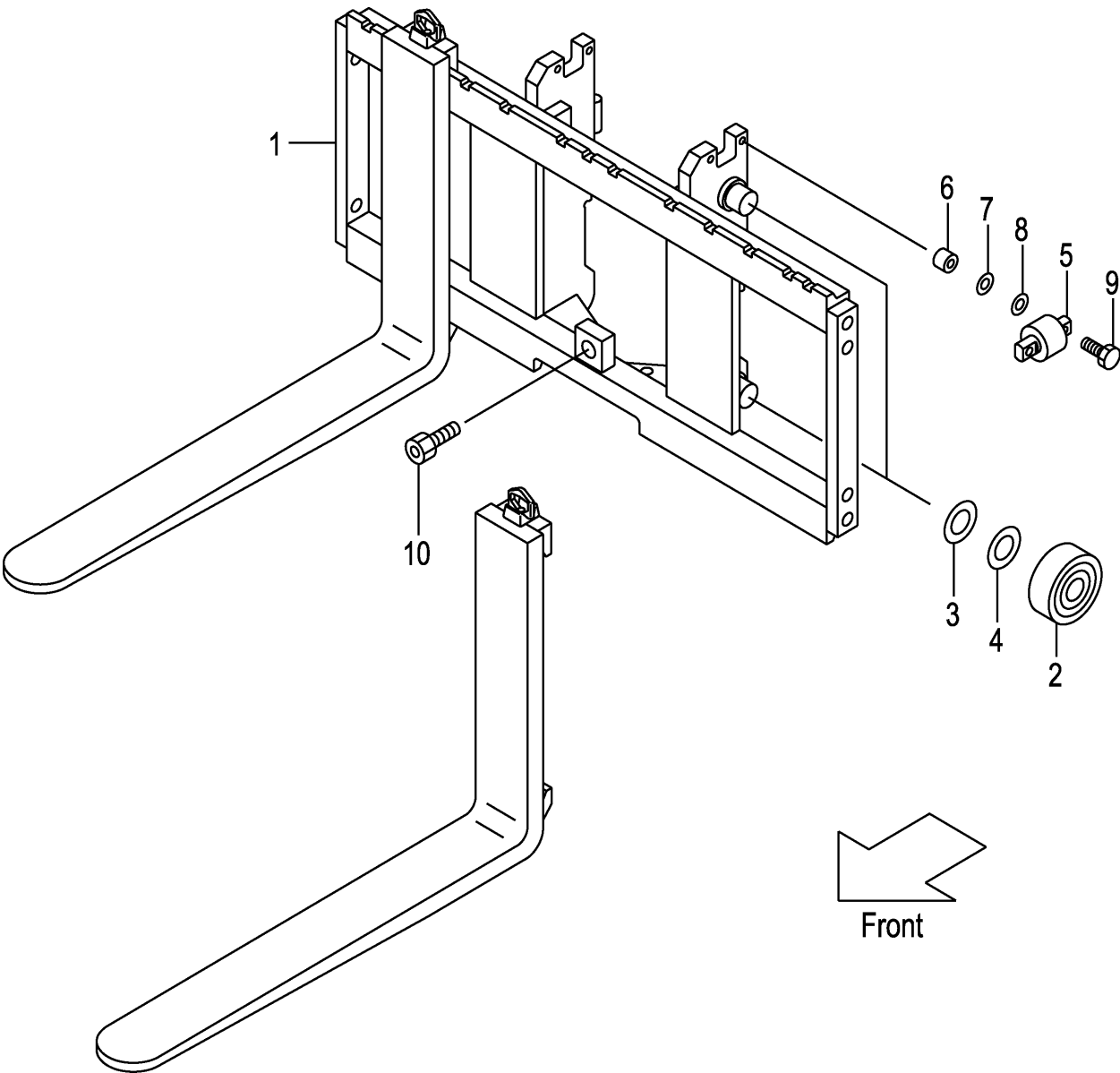
FIG.200 LIFT BRACKET [VFHM0A7] (M7010910) リフトブラケット
