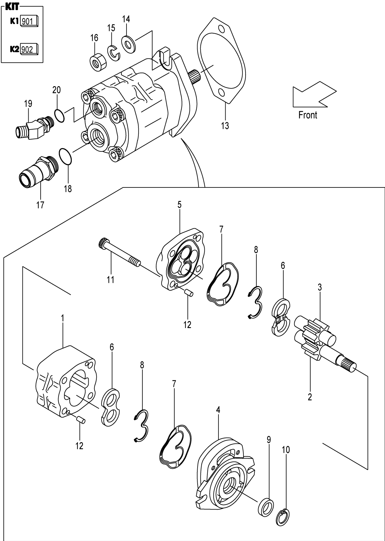
FIG.138 PUMP UNIT (F7Z17120) ポンプユニット
