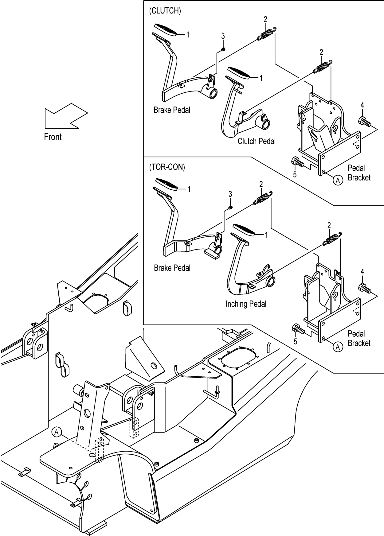
FIG.113 FOOT PEDAL PARTS (F7Z154E0) フットペダルパーツ
