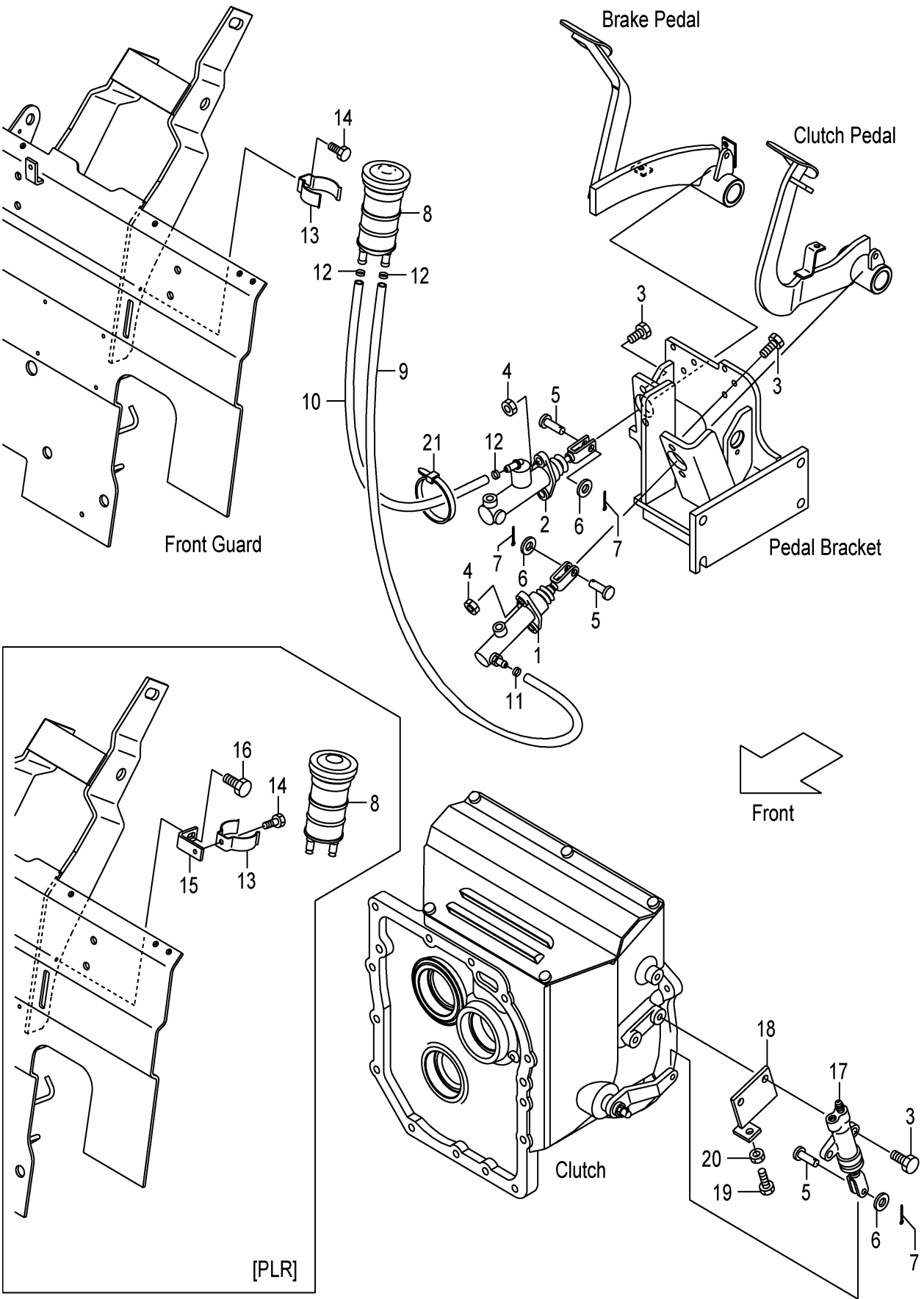
FIG.109 FOOT PEDAL CYLINDER (CLUTCH) (F7Z15440) フットペダルシリンダ
