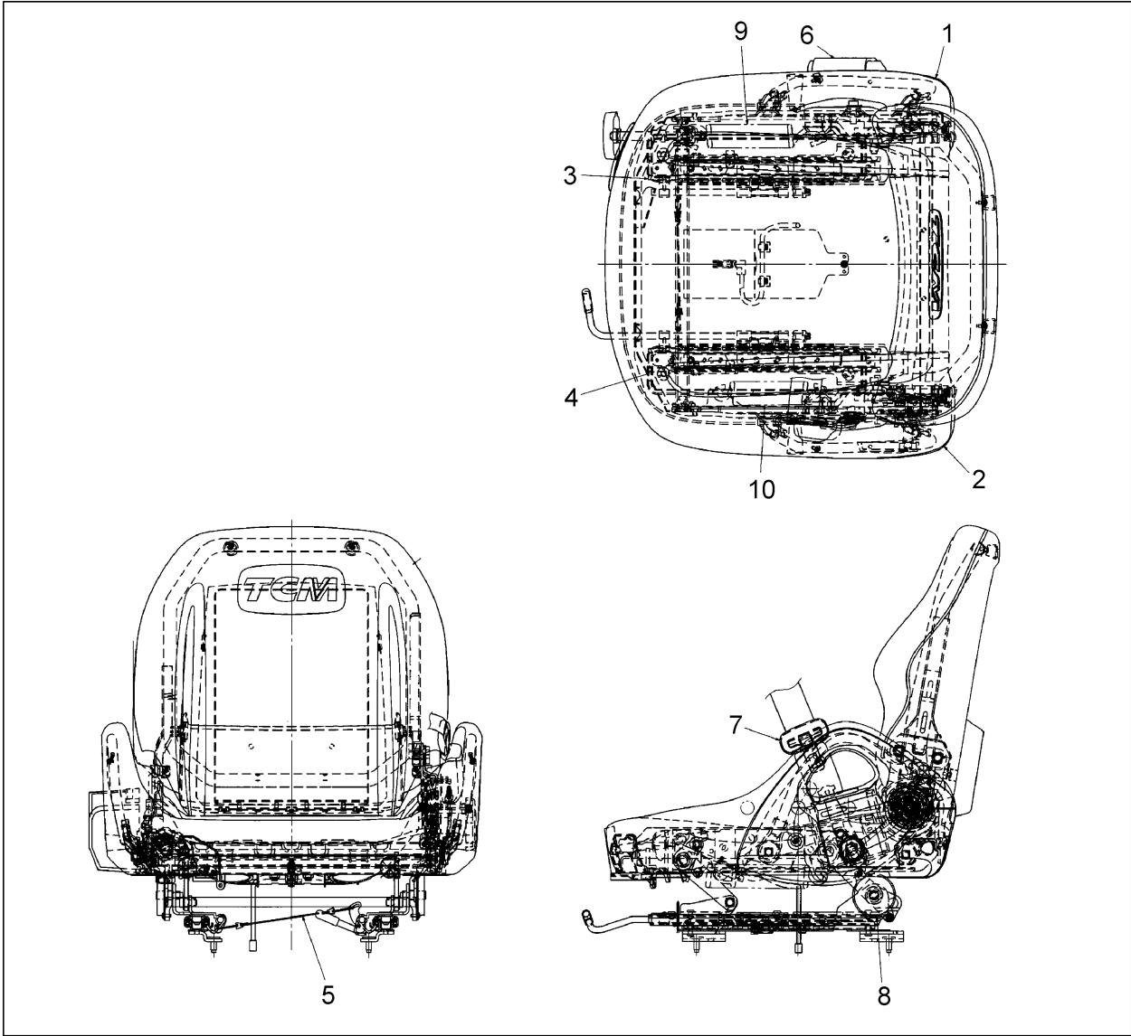
FIG.134 SEAT (F7Z16810) シート
