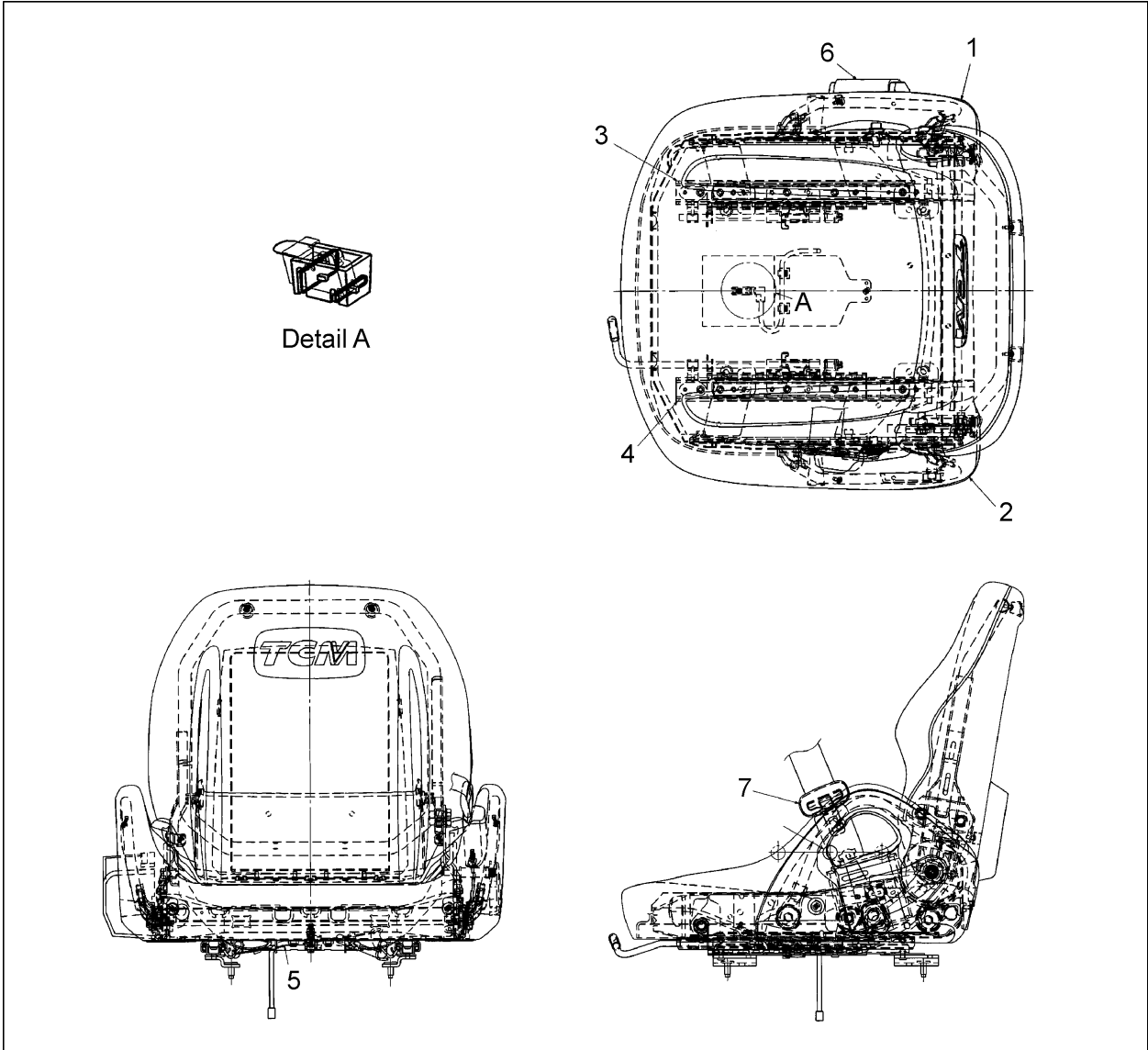
FIG.135 SEAT [HGL] (F7Z16820) シート
