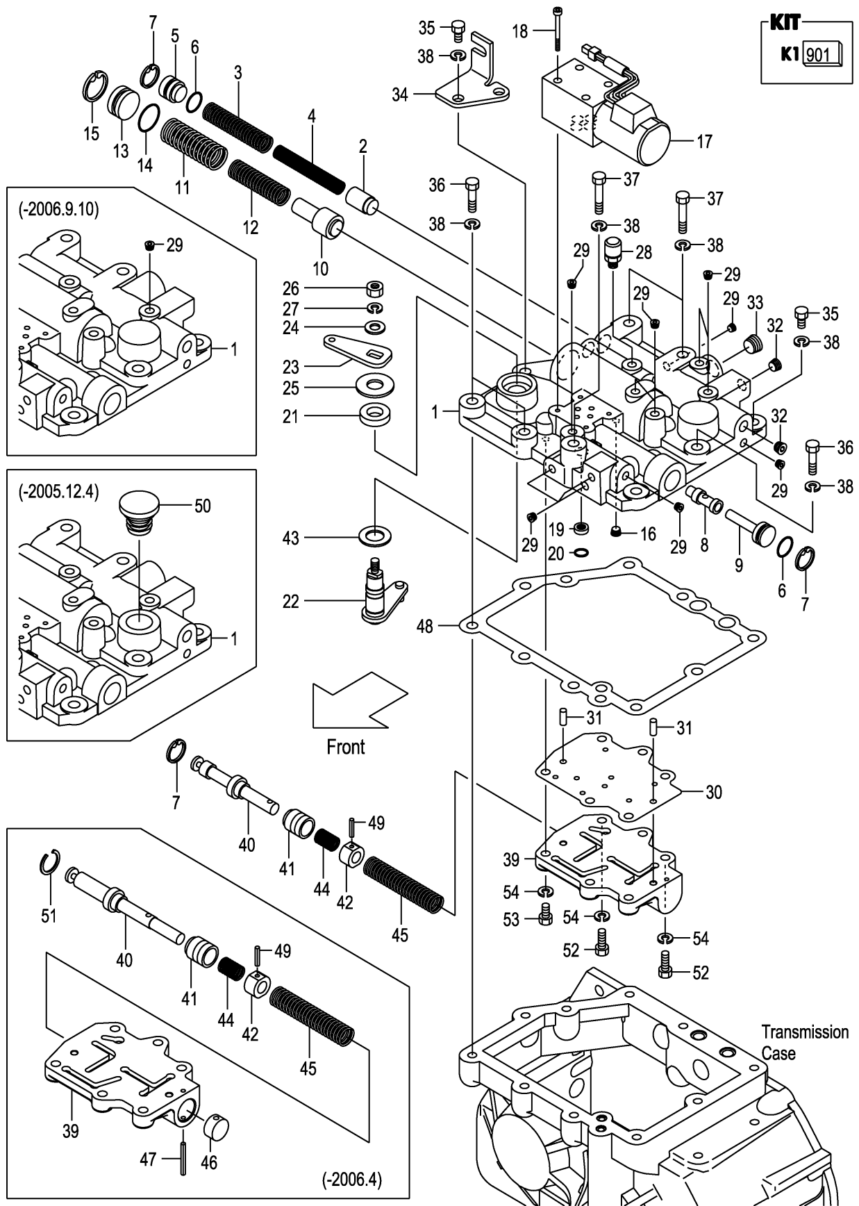
FIG.58 CONTROL VALVE (TOR-CON) (F7Z125C0) コントロールバルブ
