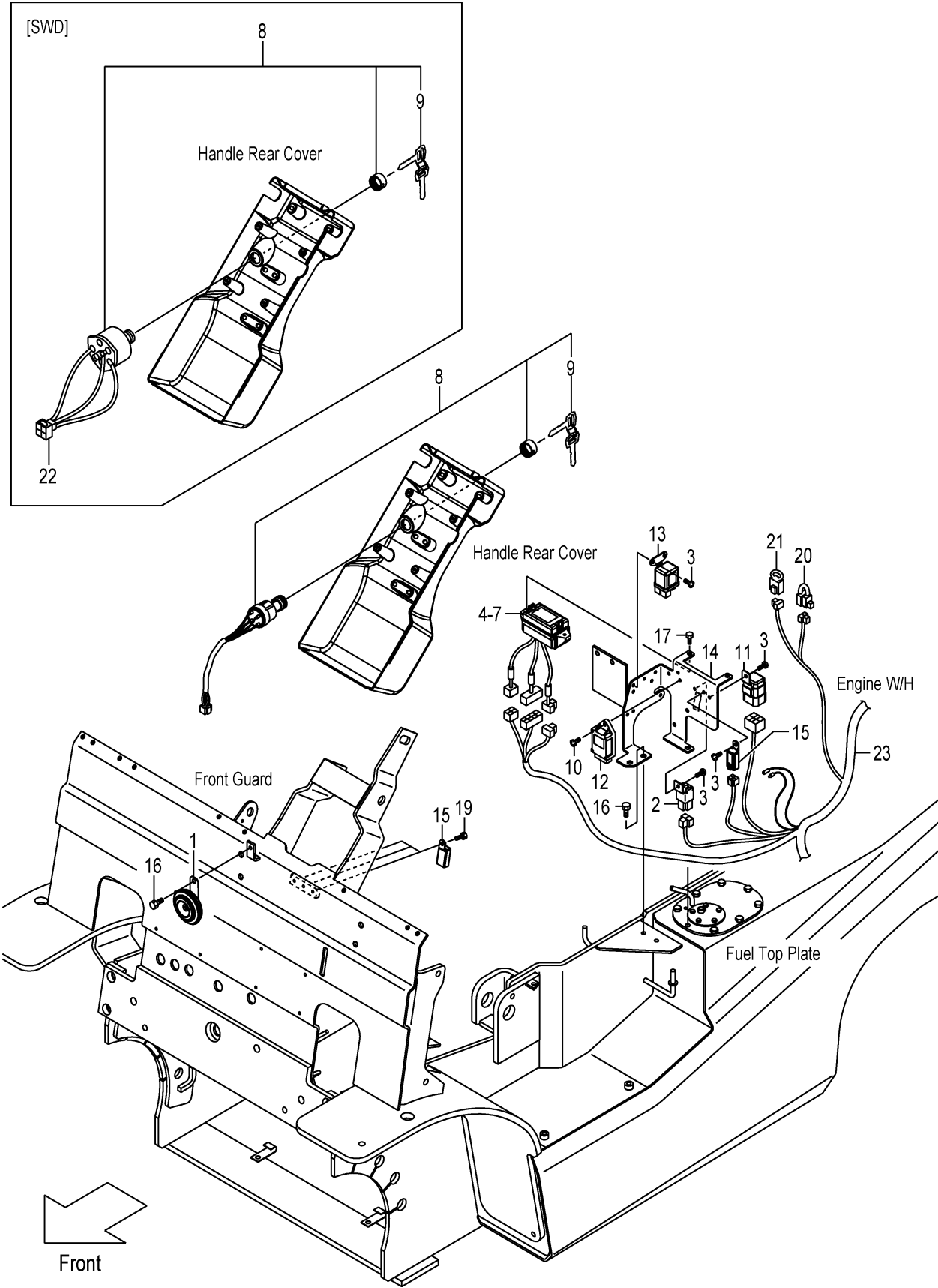
FIG.18 ELECTRIC PARTS (TOR-CON) (F7Z12490) エレクトリックパーツ
