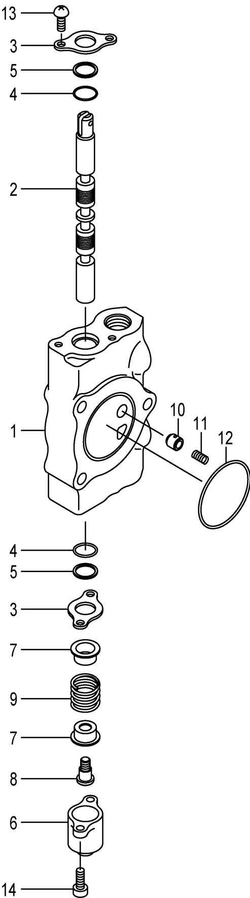
FIG.163 SPOOL SECTION (ATT)[3SV][4SV][5SV] (F7Z173P0) スプールセクション
