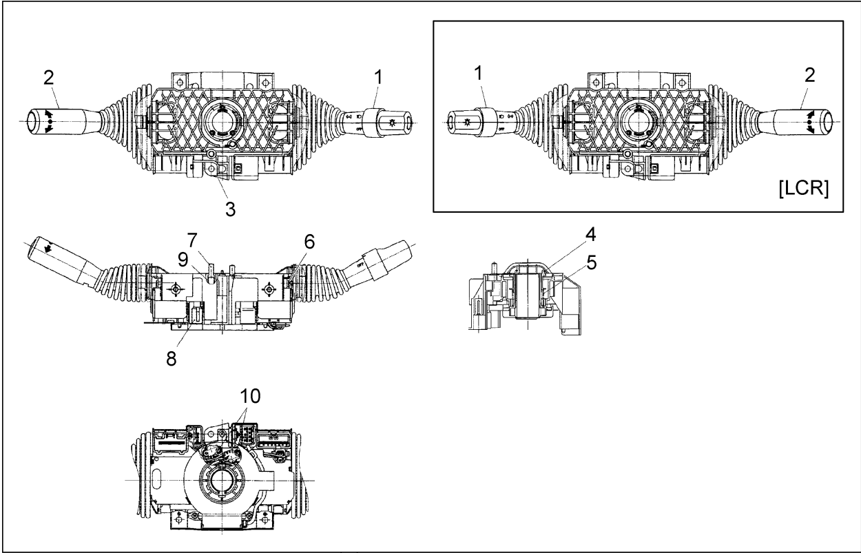
FIG.16 COMBINATION SWITCH (TOR-CON) (F7Z12450) コンビネーションスイッチ
