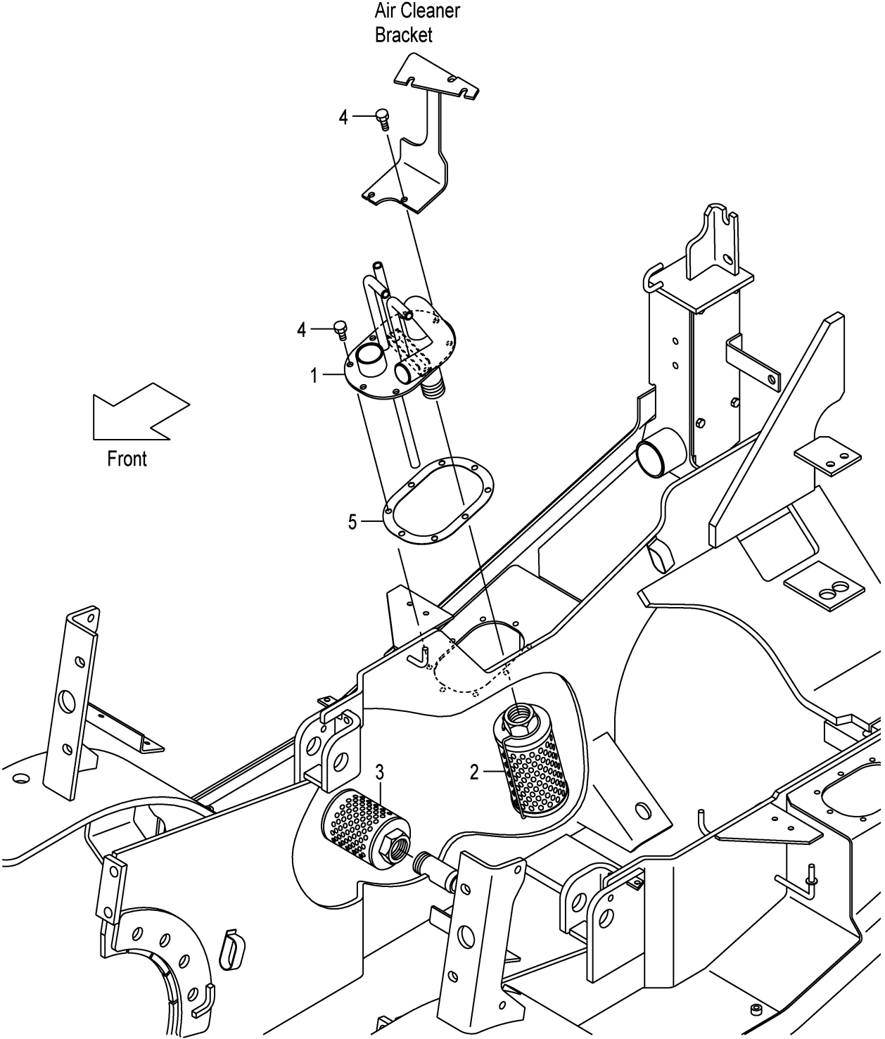
FIG.119 OIL TANK (F7Z16120) オイルタンク
