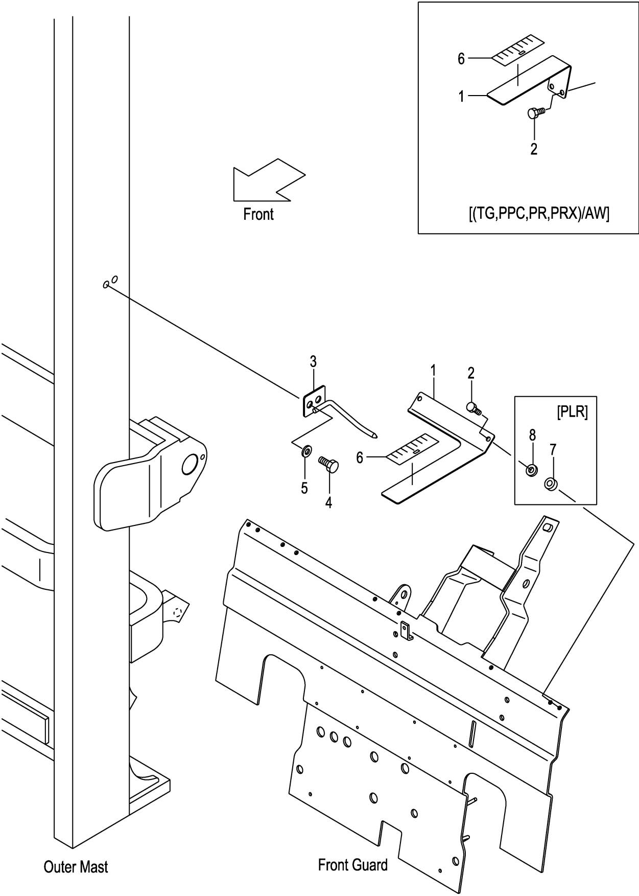
FIG.189 TILT GAUGE [VM0A7,VM0A9/(TG,PPC,PR,PRX,PLR)] (M7018320) ティルトゲージ
