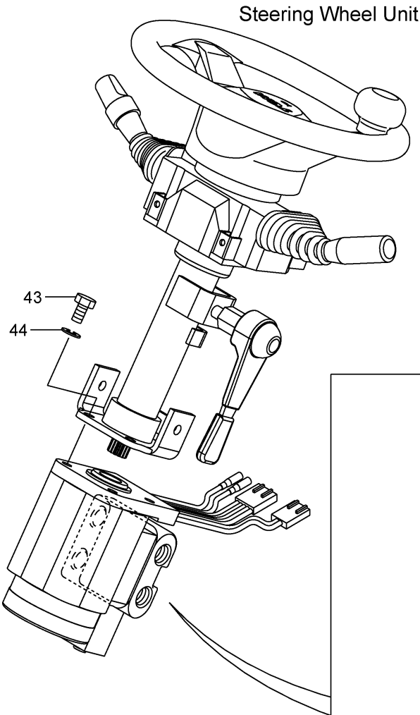
FIG.68 ORBITROL (F7Z14130) オービットロール
