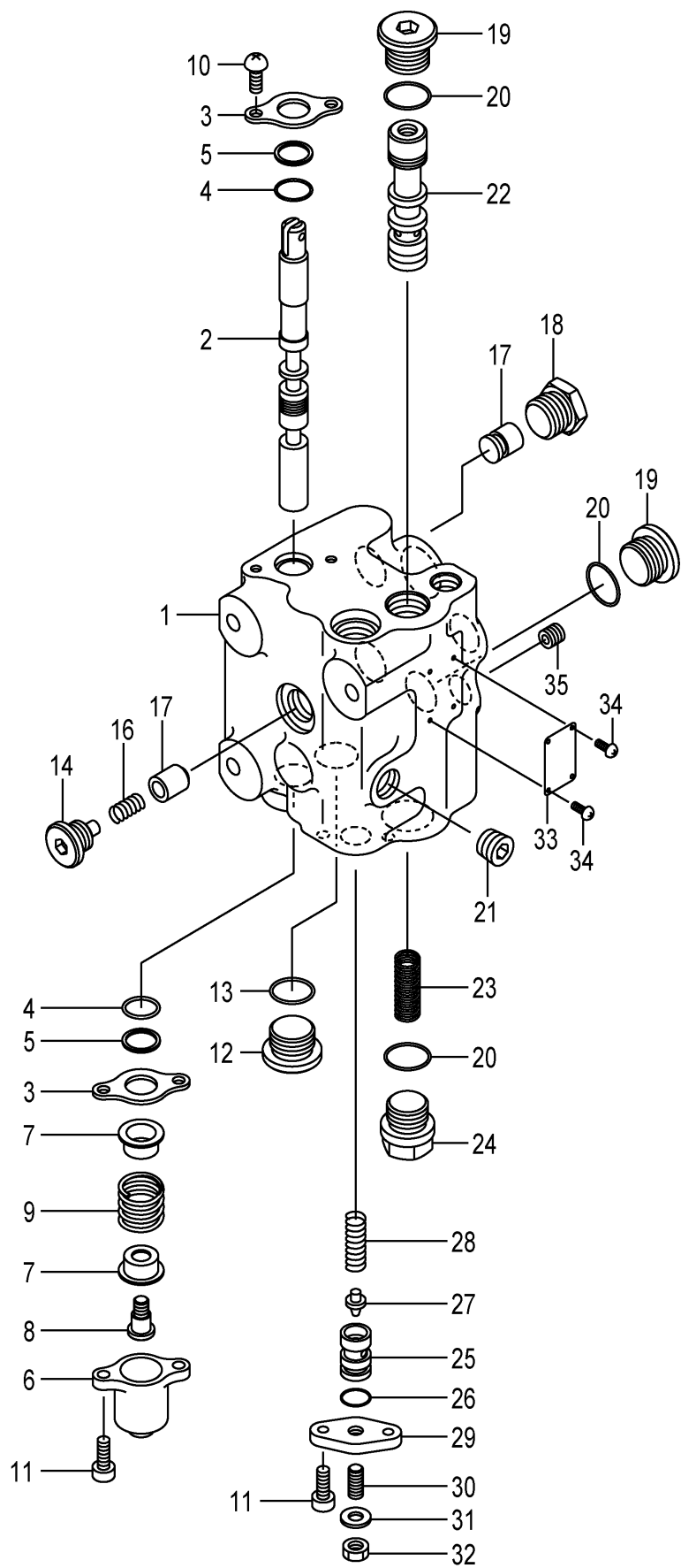
FIG.159 SPOOL SECTION (LIFT)[VLS] (F7Z173V0) スプールセクション
