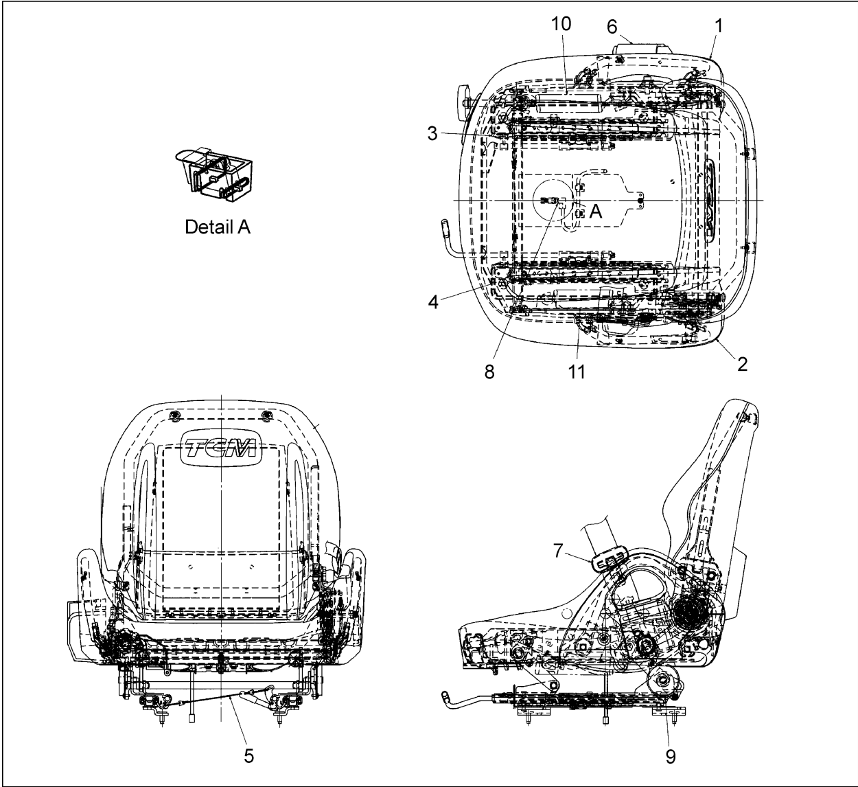
FIG.136 SEAT [SIL] (F7Z16830) シート
