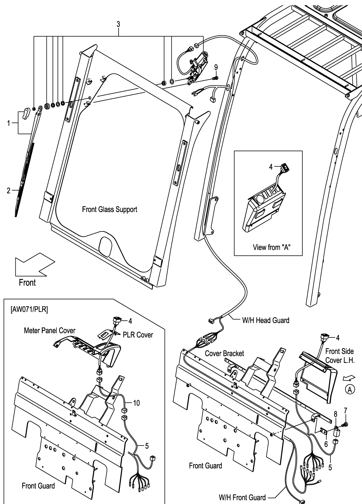
FIG.180 FRONT GLASS WIPER [AW061][AW071] (F7Z19320) フロントガラスワイパ°
