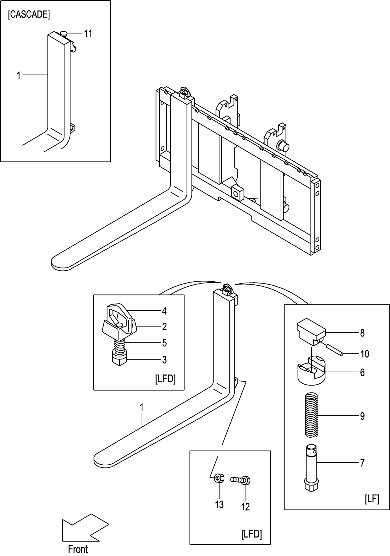
FIG.199 FORK [VFHM0A7] (M7018130) フォーク
