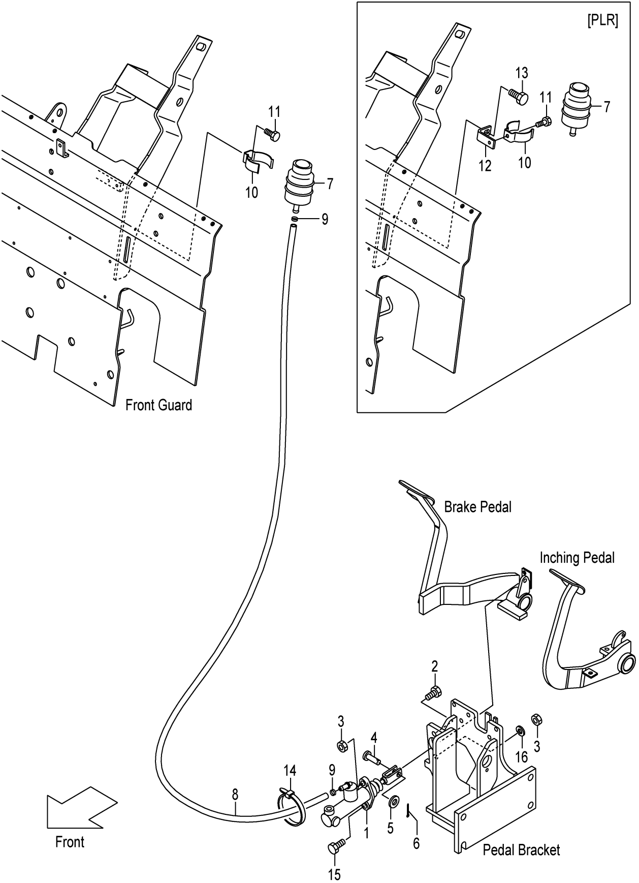
FIG.110 FOOT PEDAL CYLINDER (TOR-CON) (F7Z15450) フットペダルシリンダ
