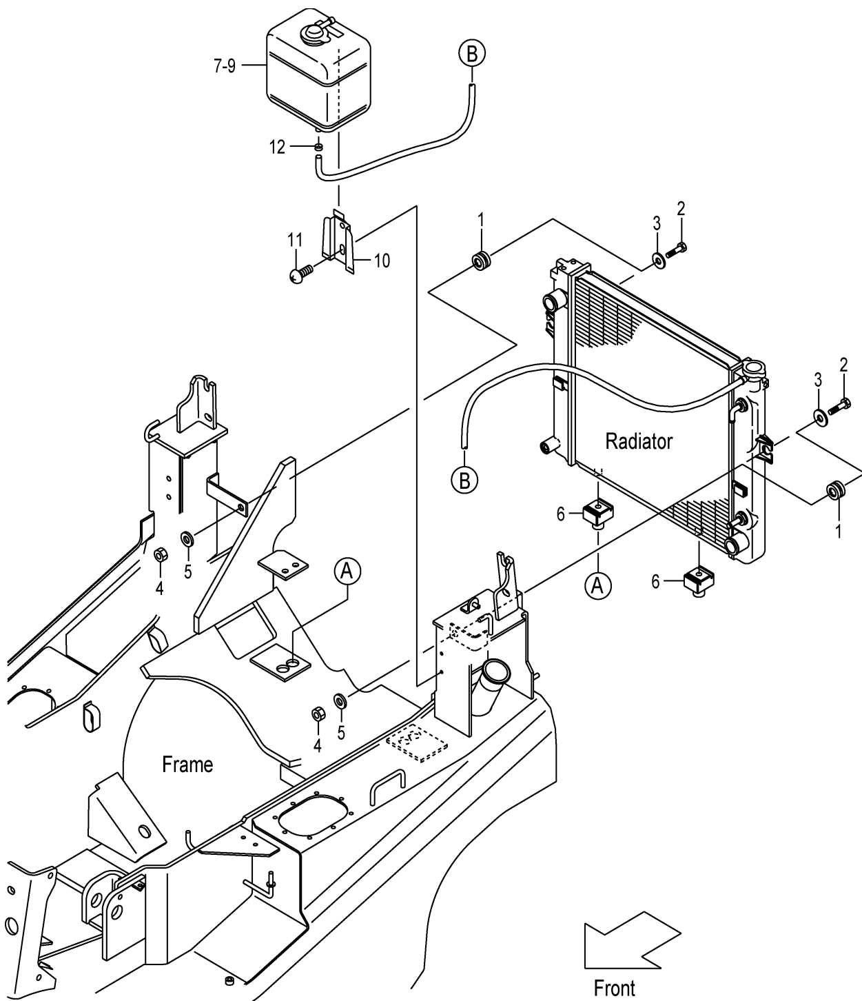
FIG.7 RADIATOR PARTS & RESERVE TANK (F7Z12150) ラジエータパーツ&リザーブタンク
