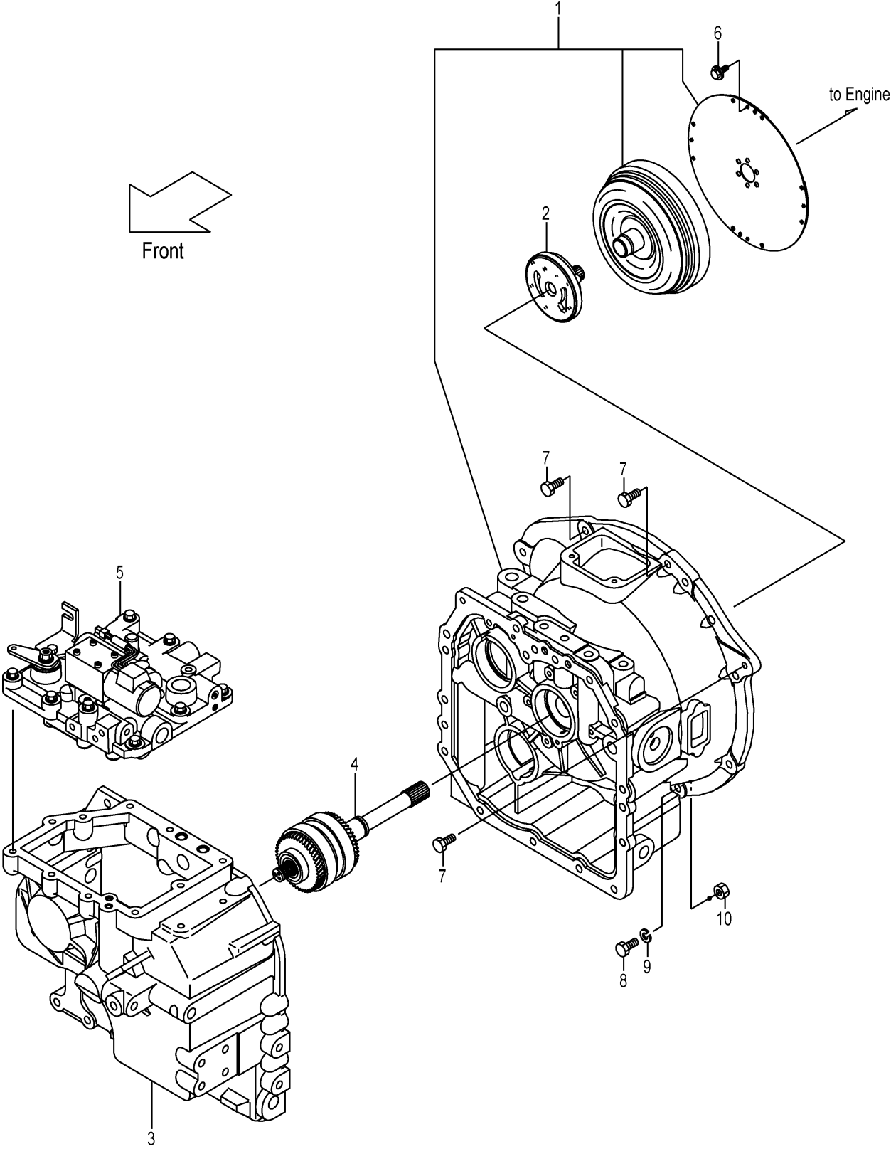
FIG.49 DRIVE UNIT MOUNT (TOR-CON) (F7Z12520) ドライブユニットマウント
