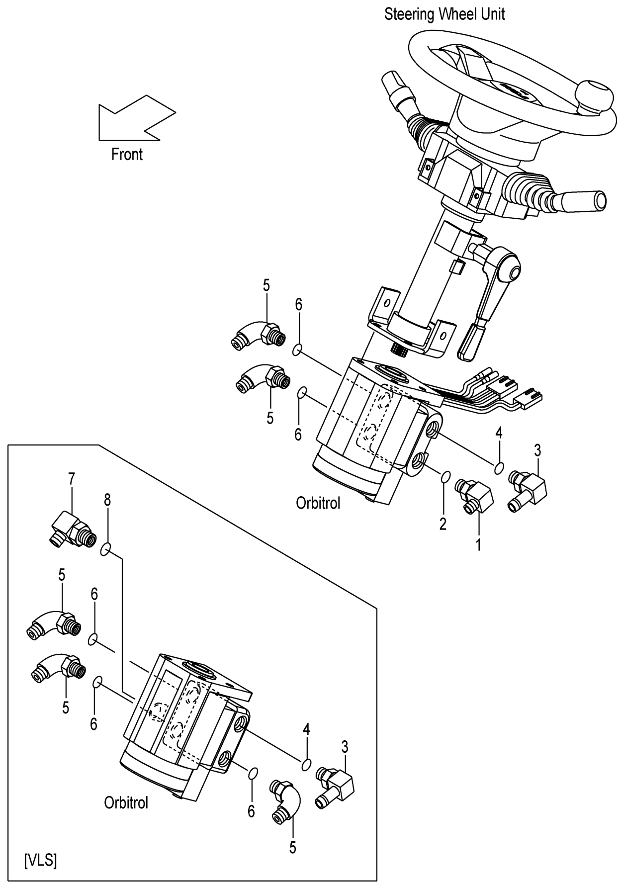
FIG.69 ORBITROL FITTING (F7Z14140) オービットロールフィッティング
