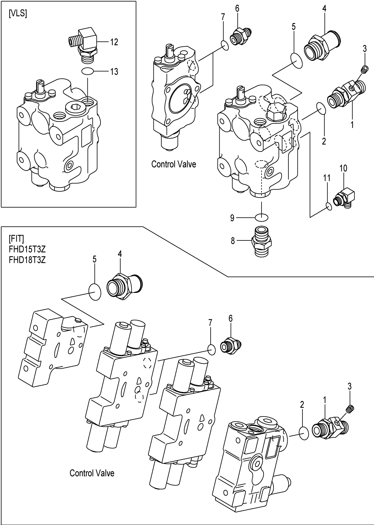
FIG.146 CONTROL VALVE FITTING (F7Z17390) コントロールバルブフィッティング
