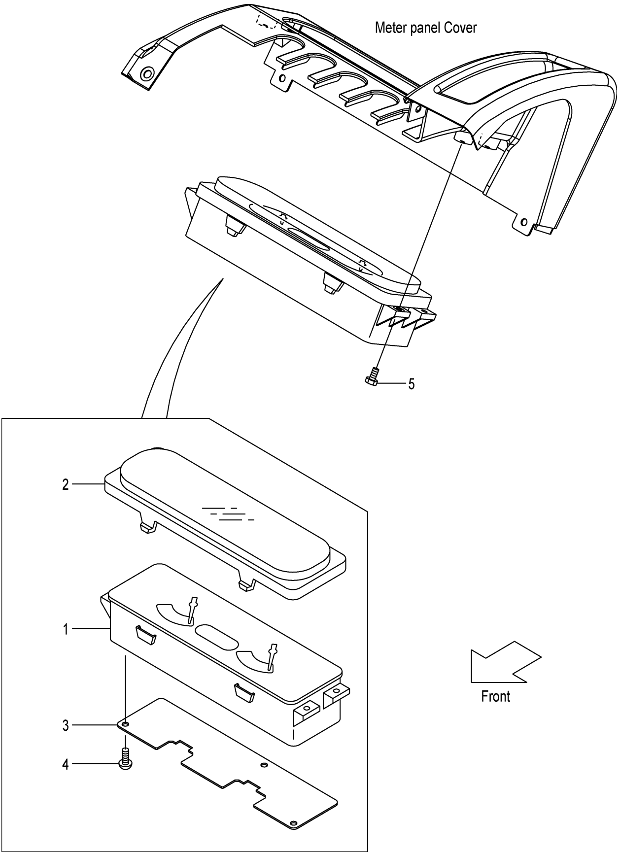
FIG.12 COMBINATION METER (F7Z12410) コンビネーションメータ
