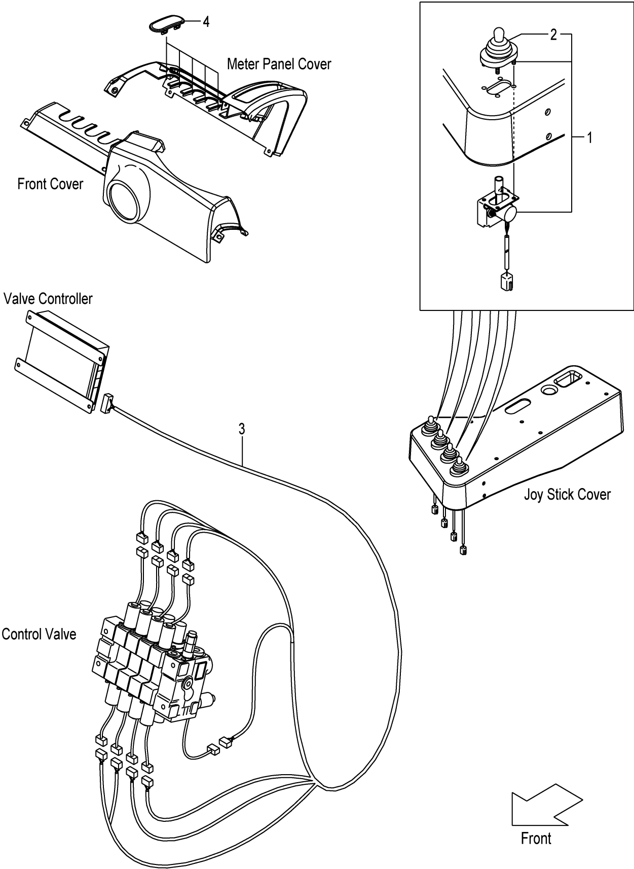
FIG.153 VALVE CONTROL (TOR-CON):[4SV/FIT] (F7Z173G0) バルブコントロール
