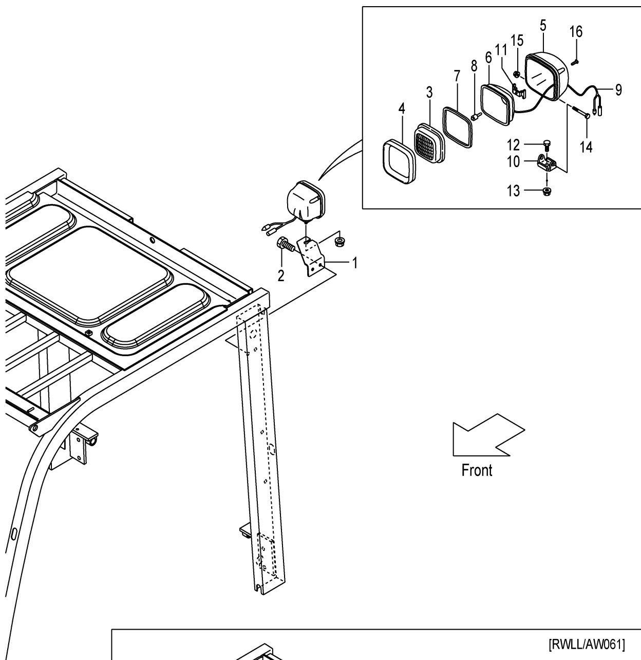
FIG.24 REAR WORKING LIGHT [RWLL] (F7Z124Q0) リヤワーキングライト
