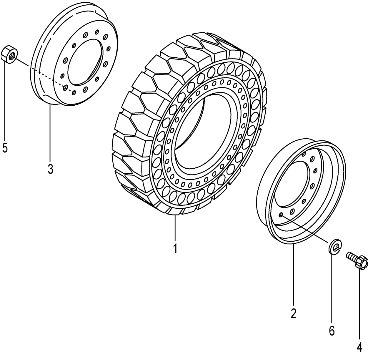
FIG.95 REAR WHEEL [TRAR] (F7Z144Q0) リヤホイール
