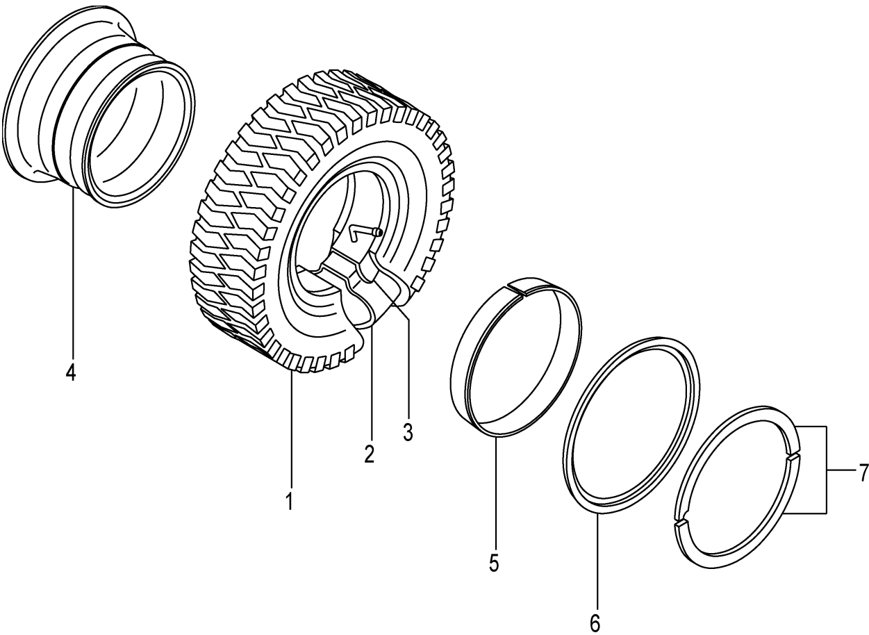
FIG.75 FRONT WHEEL (1.8T) (F7Z14440) フロントホイール
