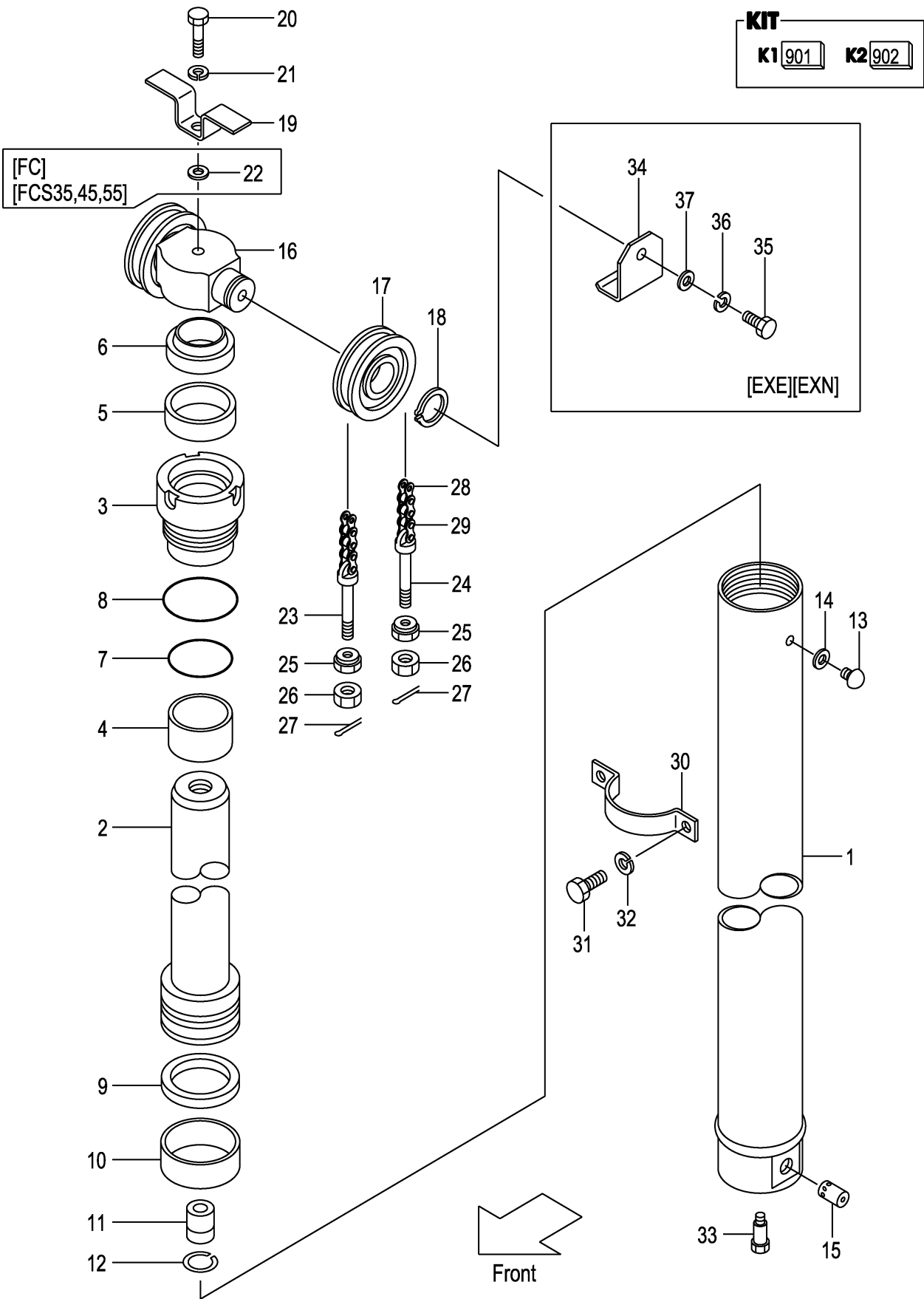
FIG.196 LIFT CYLINDER (FRONT)[VFM0A7] (M7010510) リフトシリンダ(フロント)
