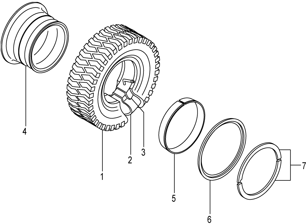
FIG.90 REAR WHEEL [DR R] (F7Z144K0) リヤホイール
