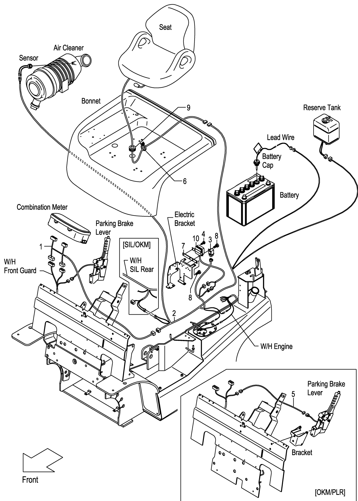
FIG.45 OK MONITOR [OKM] (F7Z126J0) OKモニター
