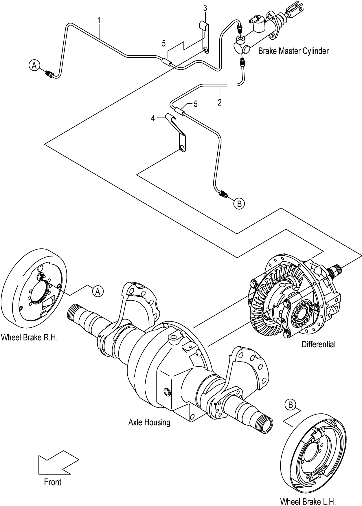
FIG.112 BRAKE PIPE (TOR-CON) (F7Z154A0) ブレーキパイプ
