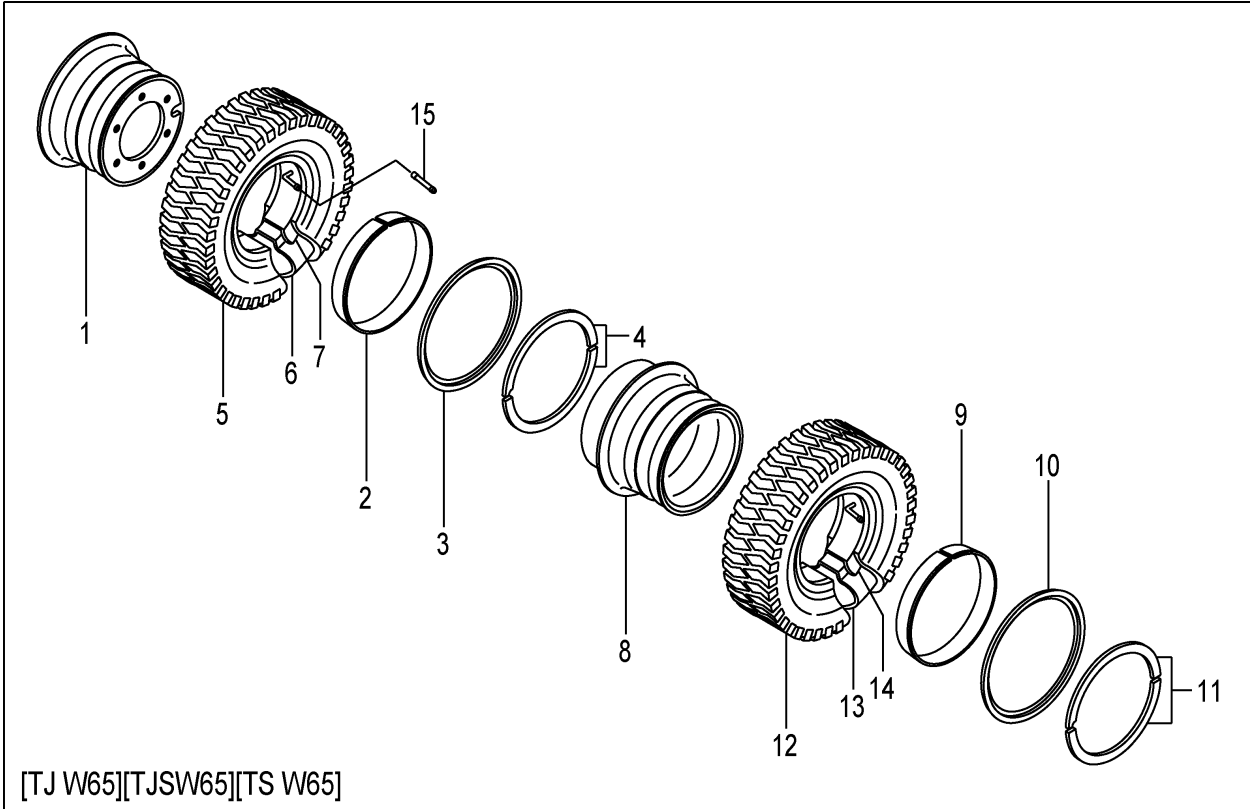
FIG.87 FRONT WHEEL [TJ W65][TJSW65][TW65][TS W65] (F7Z144G0) フロントホイール
