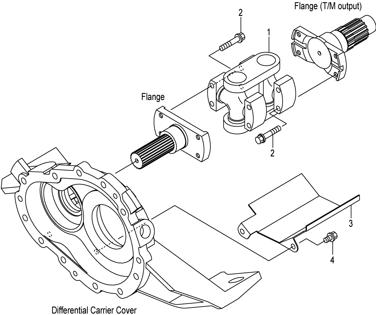
FIG.61 PROPELLER SHAFT (F7Z13310) プロペラシャフト
