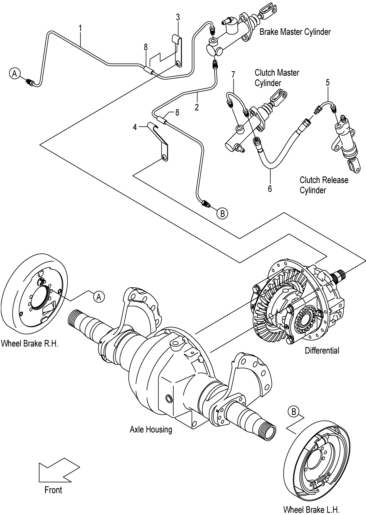
FIG.111 BRAKE PIPE (CLUTCH) (F7Z15490) ブレーキパイプ
