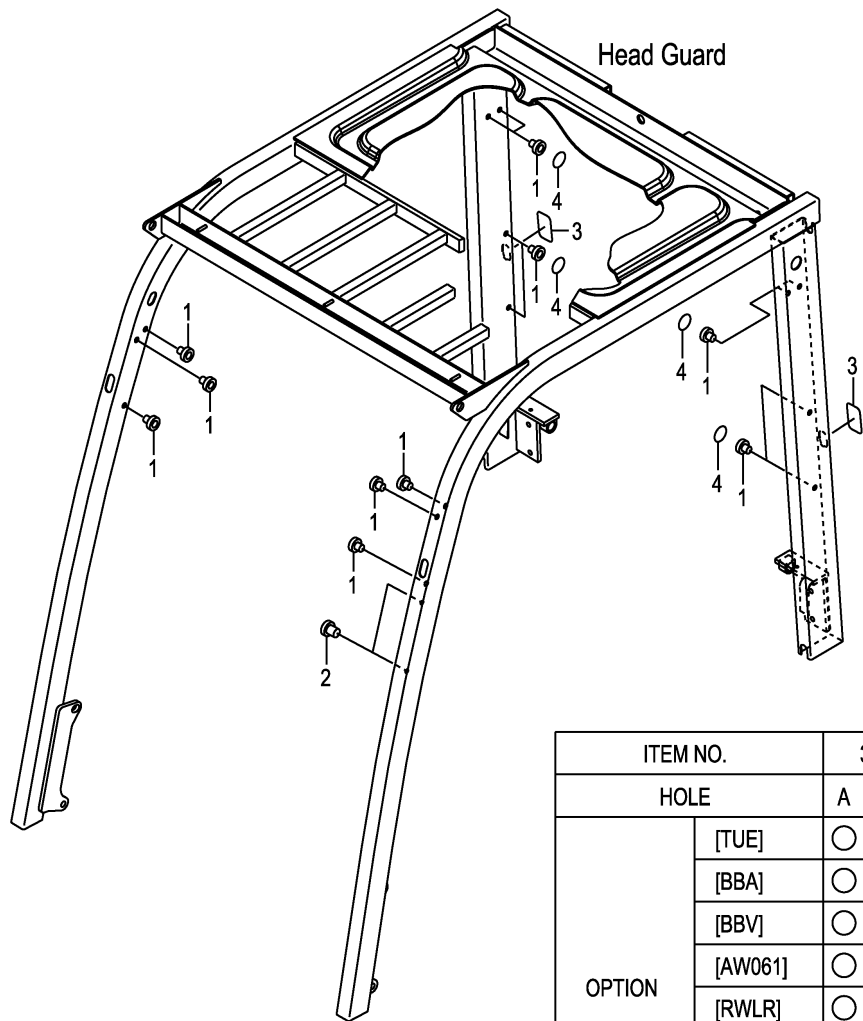
FIG.105 POP RIVET [TUE][BBA][BBV][AW061][RWL][RRE][FE] (F7Z151C0) ポップリベット
