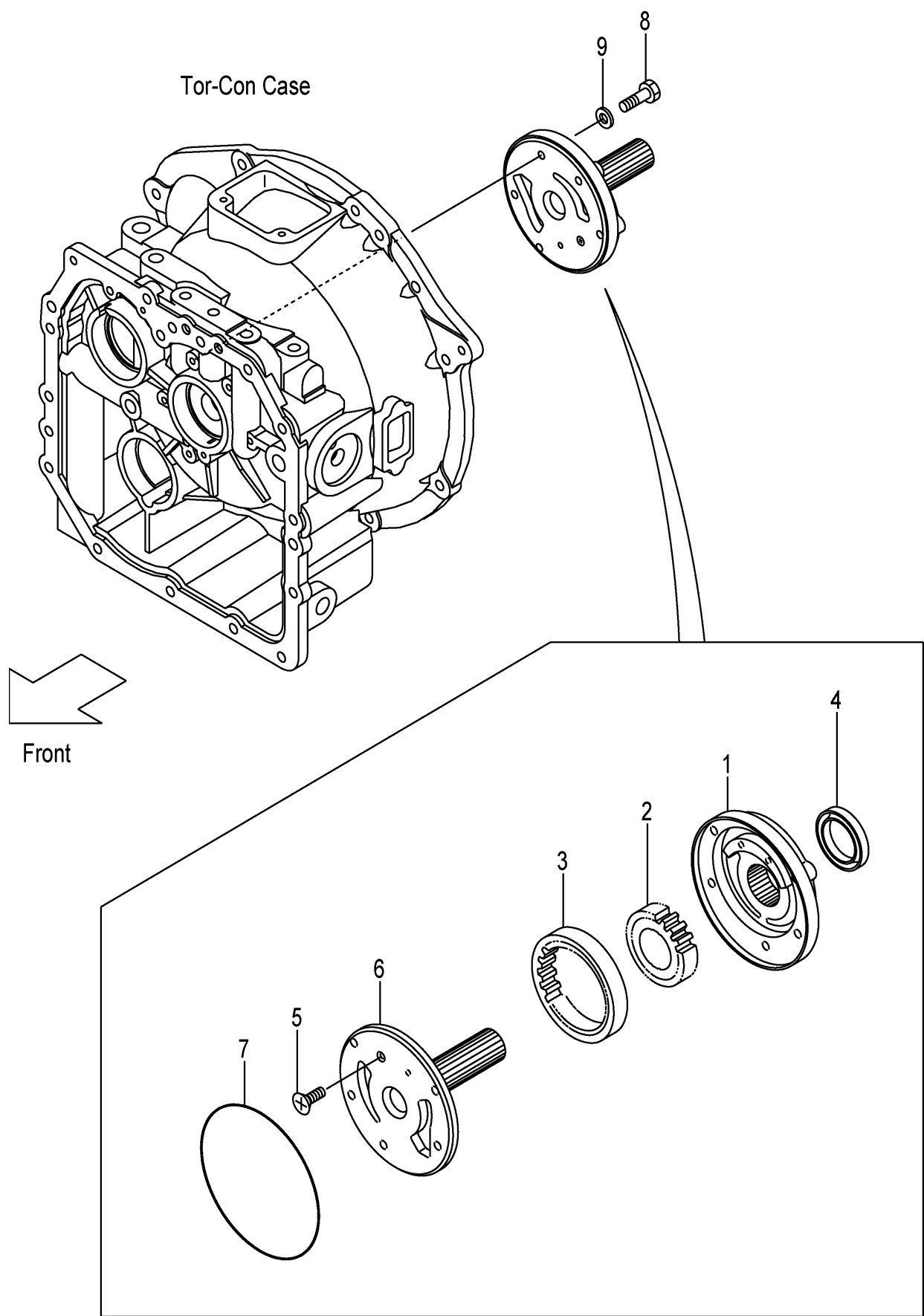
FIG.55 CHARGING PUMP (TOR-CON) (F7Z12590) チャージングポンプ°
