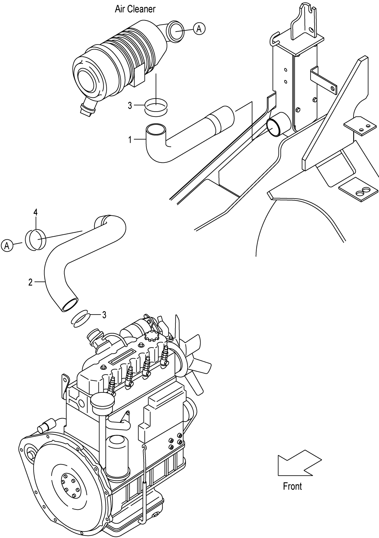
FIG.3 AIR DUCT (F7Z11060) エアークラウド
