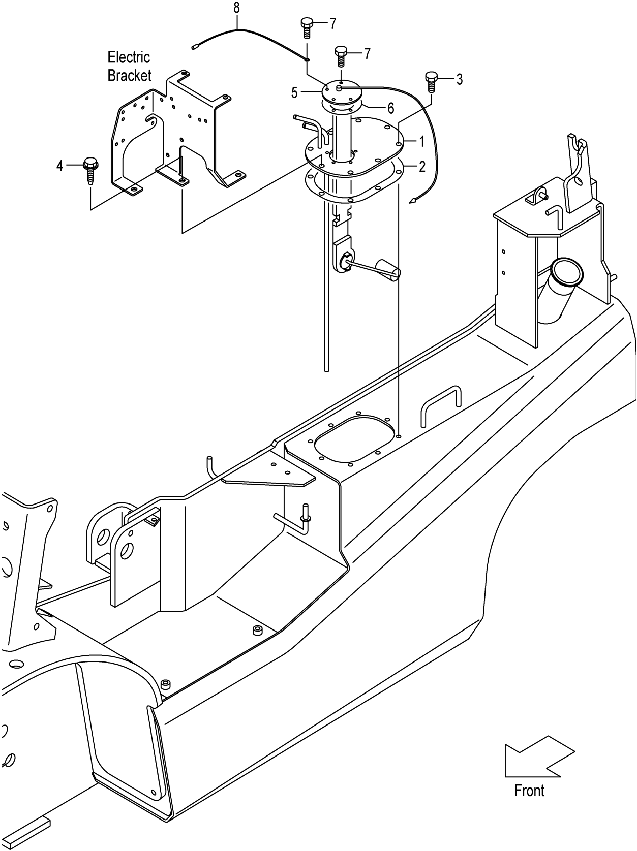
FIG.121 FUEL TANK (F7Z16150) フューエルタンク
