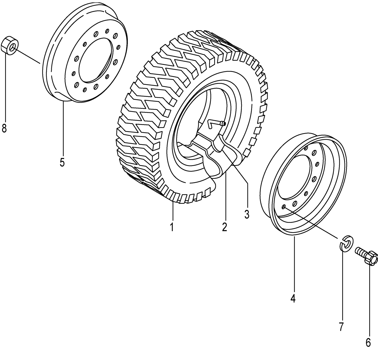
FIG.74 FRONT WHEEL (1.5T) (F7Z14430) フロントホイール
