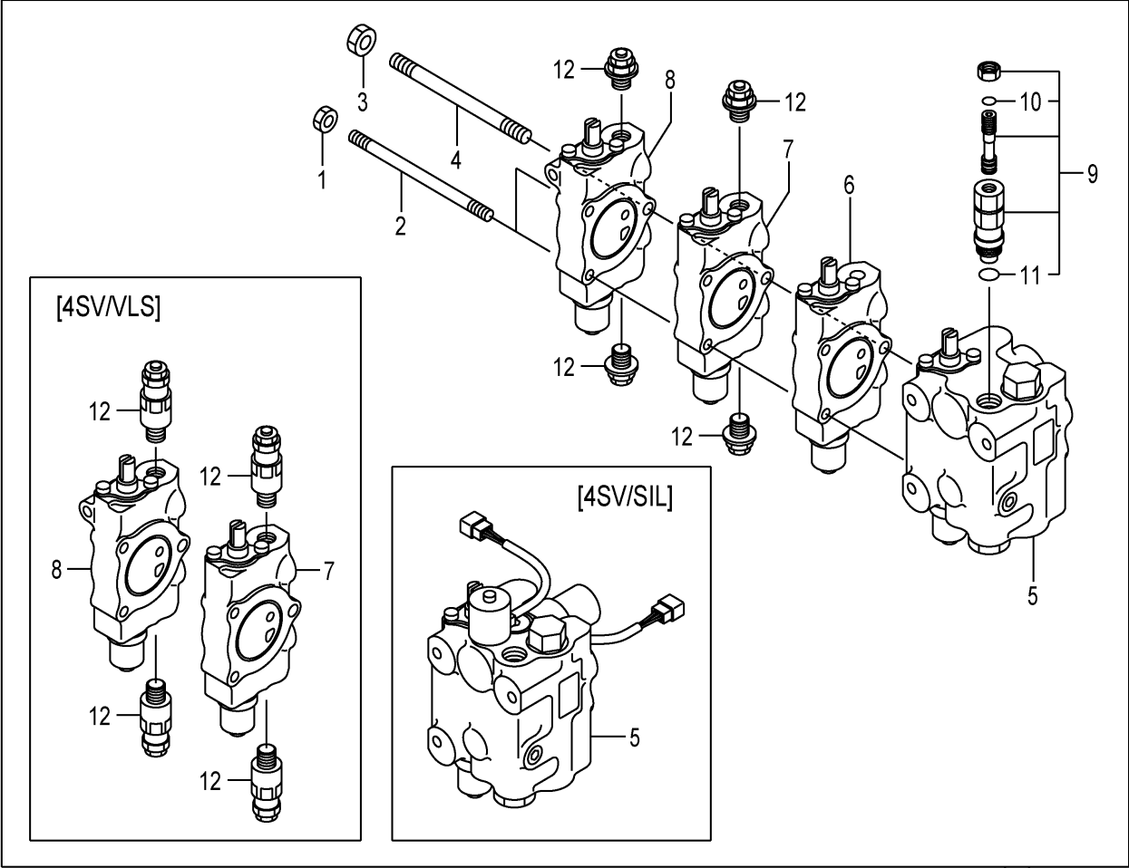
FIG.141 CONTROL VALVE [4SV] (F7Z17330) コントロールバルブ
