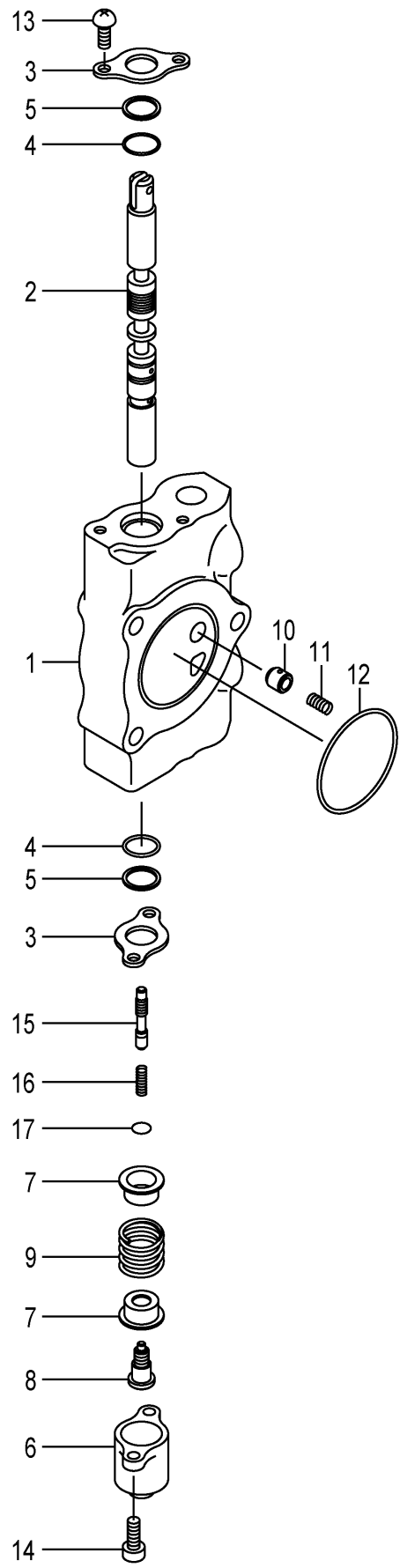
FIG.160 SPOOL SECTION (TILT) (F7Z173N0) スプールセクション
