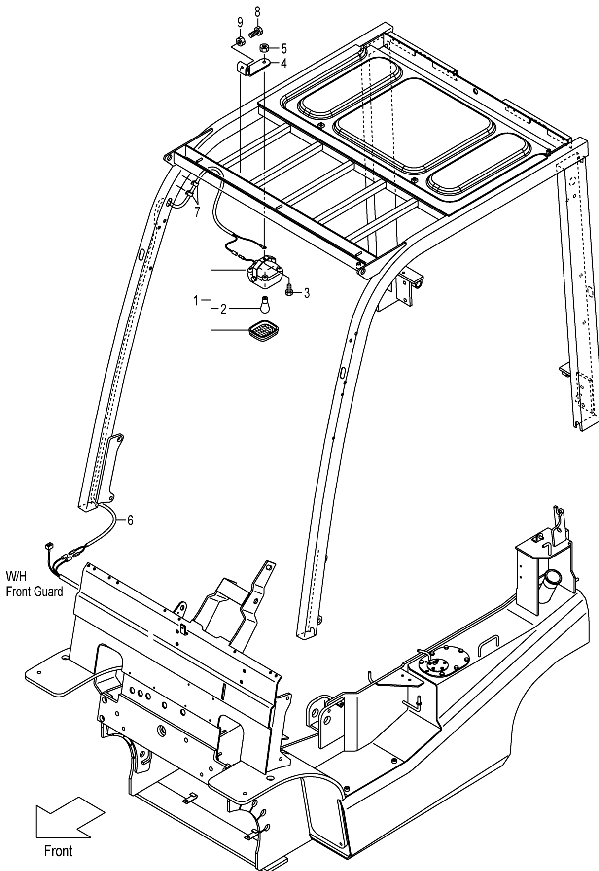
FIG.31 SPOT LIGHT [SPL] (F7Z12640) スポットライト
