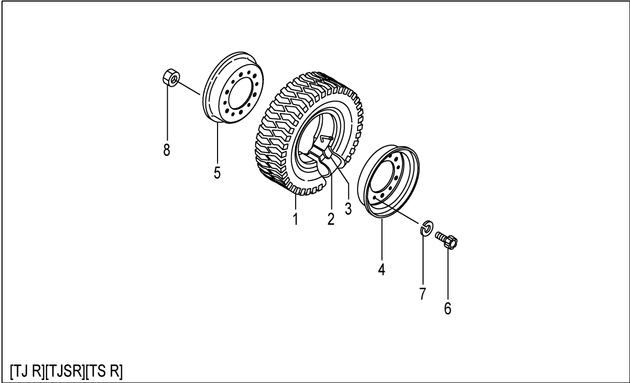
FIG.91 REAR WHEEL [TJ R][TJSR][TR][TS R] (F7Z144L0) リヤホイール
