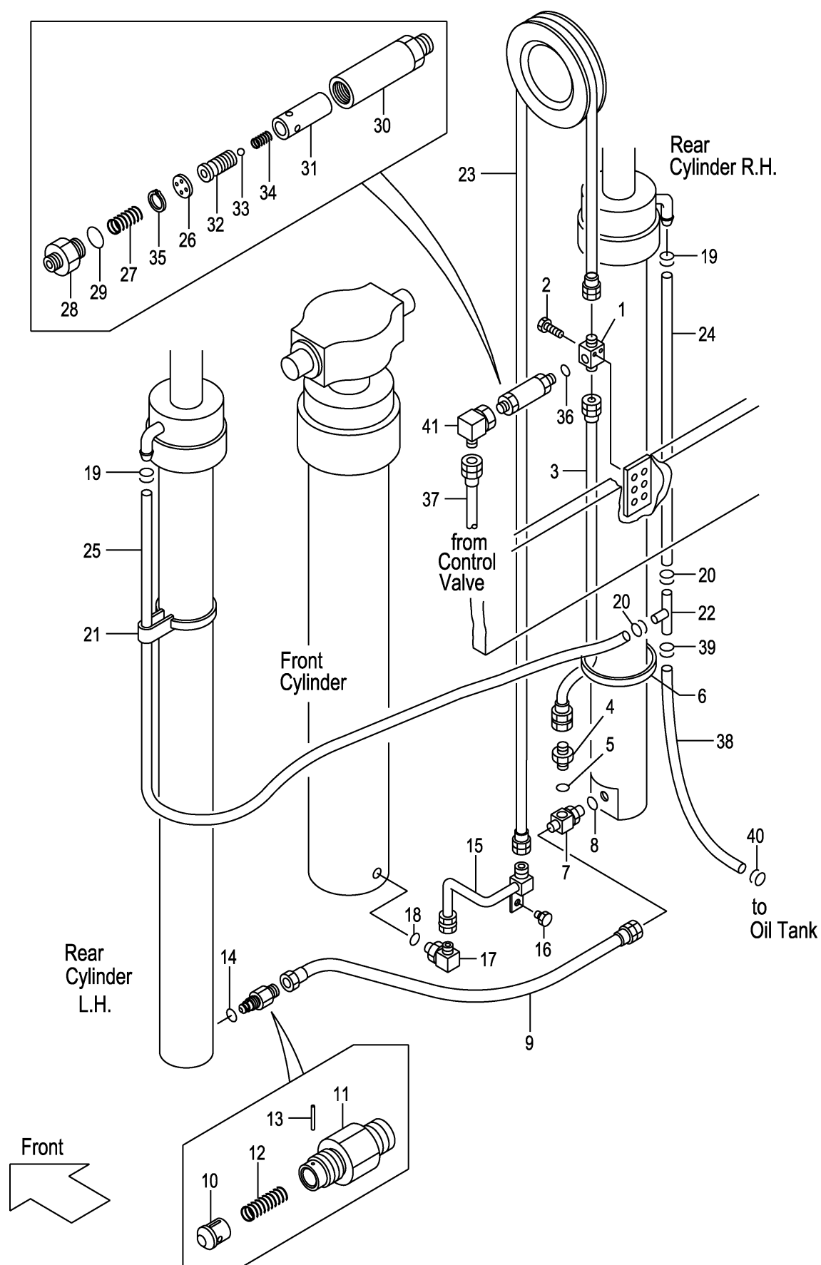
FIG.205 MAST PIPING [VFHM0A7] (M7010830) マストパイピング
