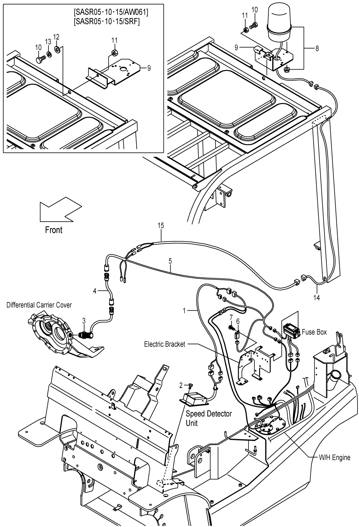
FIG.43 SPEED ALARM SYSTEM [SASR] (F7Z126G0) スピード・アラームシステム
