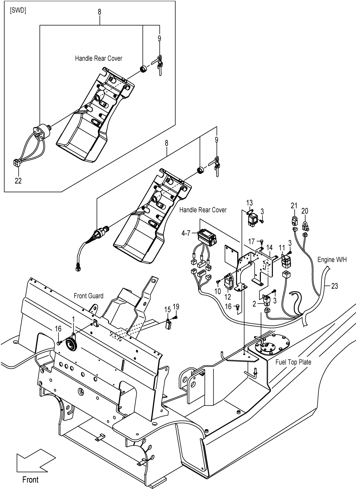
FIG.17 ELECTRIC PARTS (CLUTCH) (F7Z12480) エレクトリックパーツ
