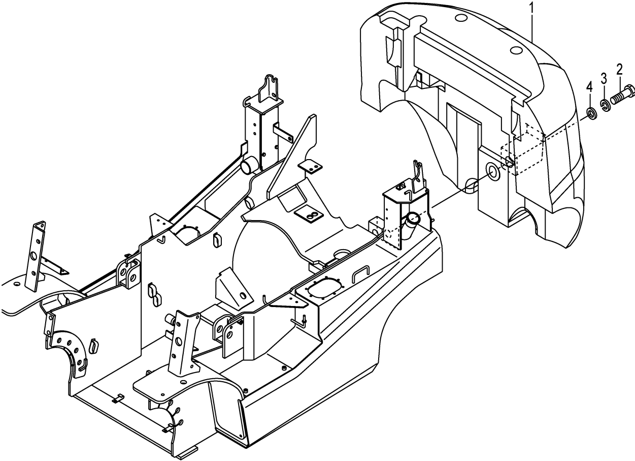
FIG.122 BALANCE WEIGHT (F7Z16310) バランスウェイト
