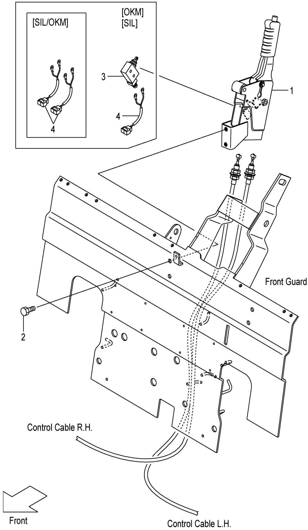
FIG.117 BRAKE LEVER (F7Z15510) ブレーキレバー
