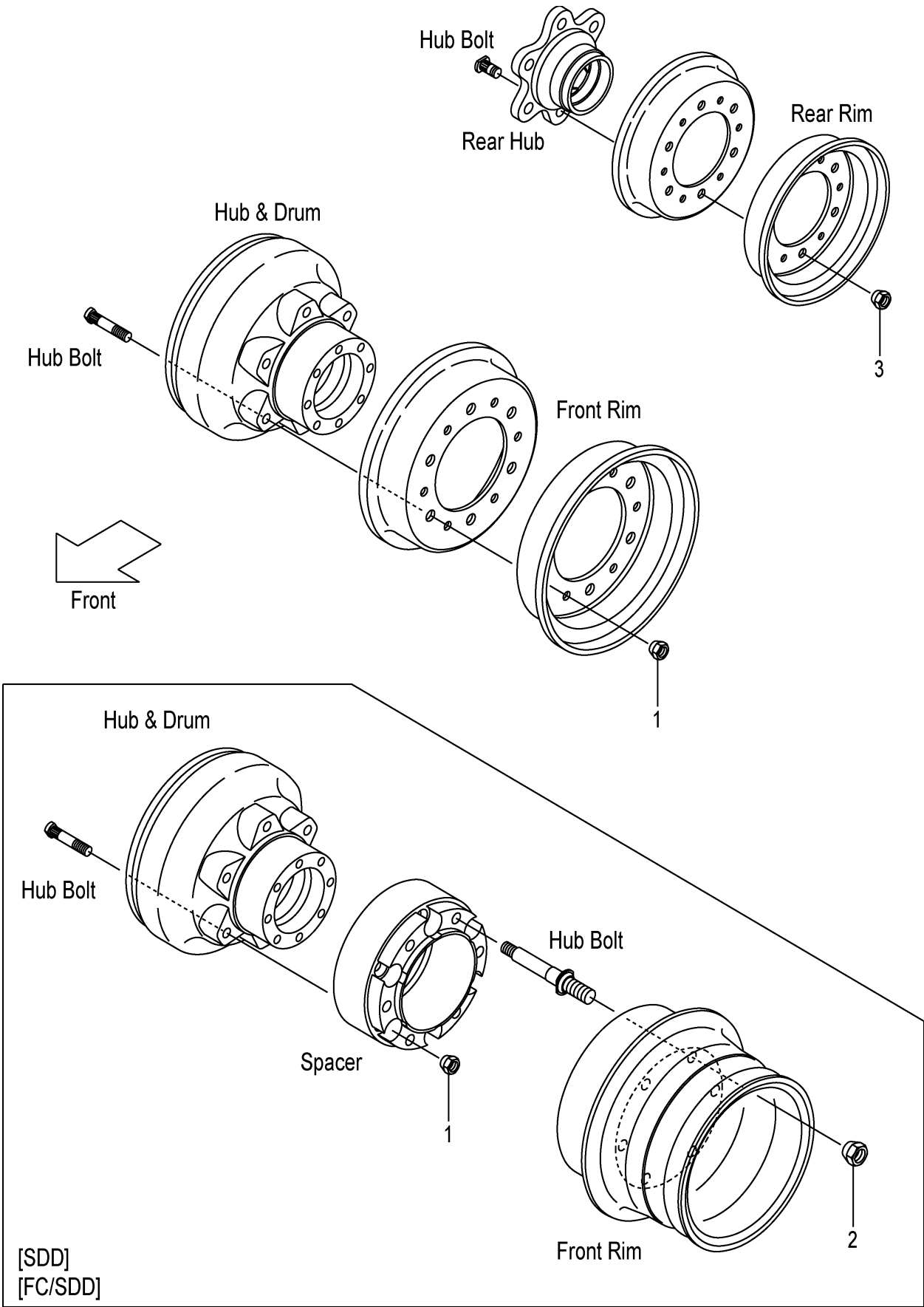
FIG.72 HUB NUT (F7Z14410) ハブナット
