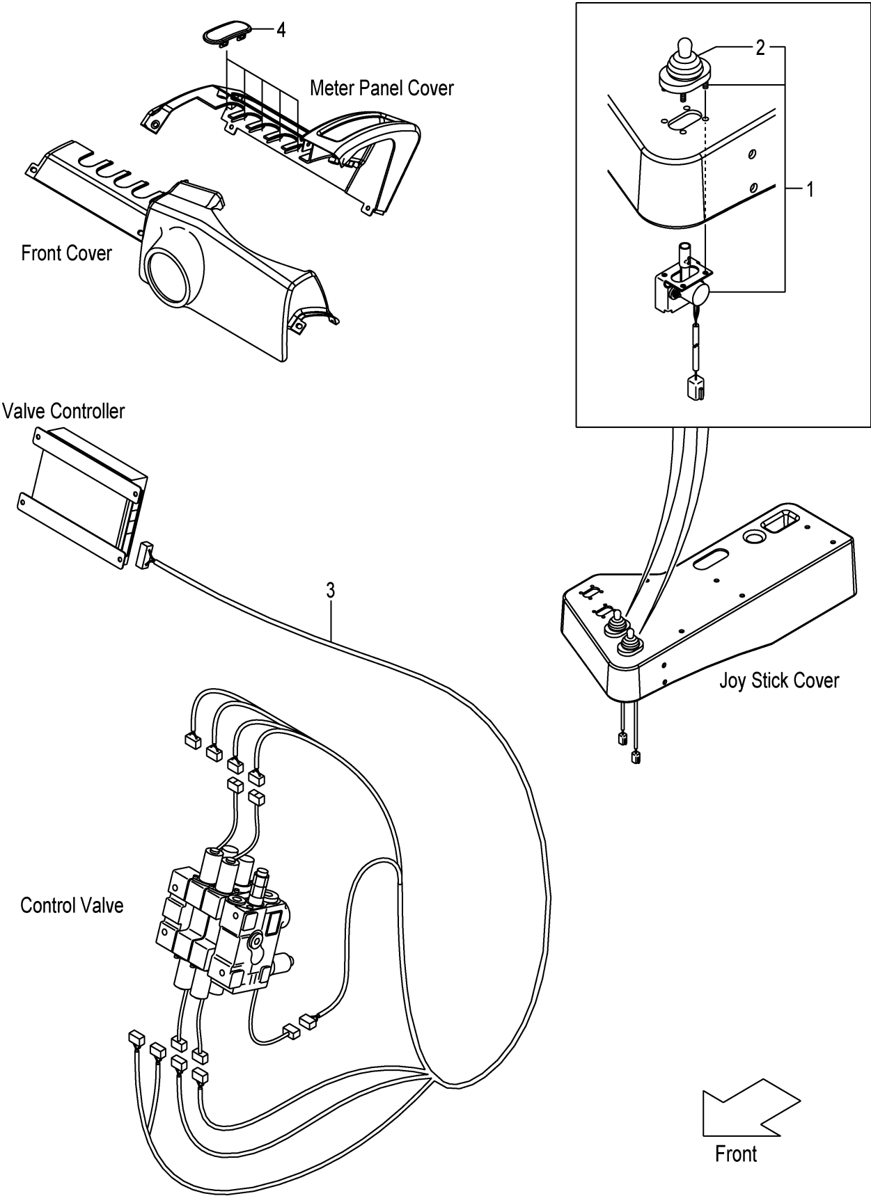
FIG.151 VALVE CONTROL (TOR-CON):[FIT] (F7Z173E0) バルブコントロール
