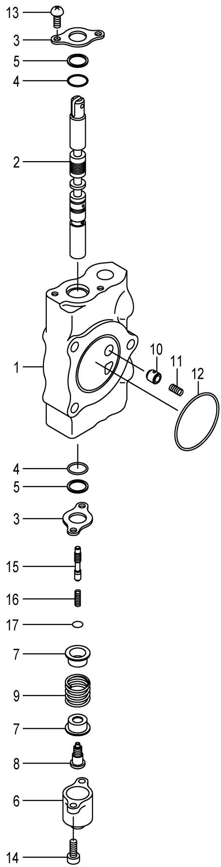
FIG.162 SPOOL SECTION (TILT)[VLS] (F7Z173W0) スプールセクション
