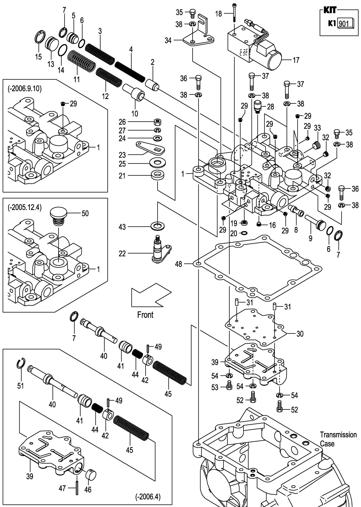
(F7Z125C0) コントロールバルブ
