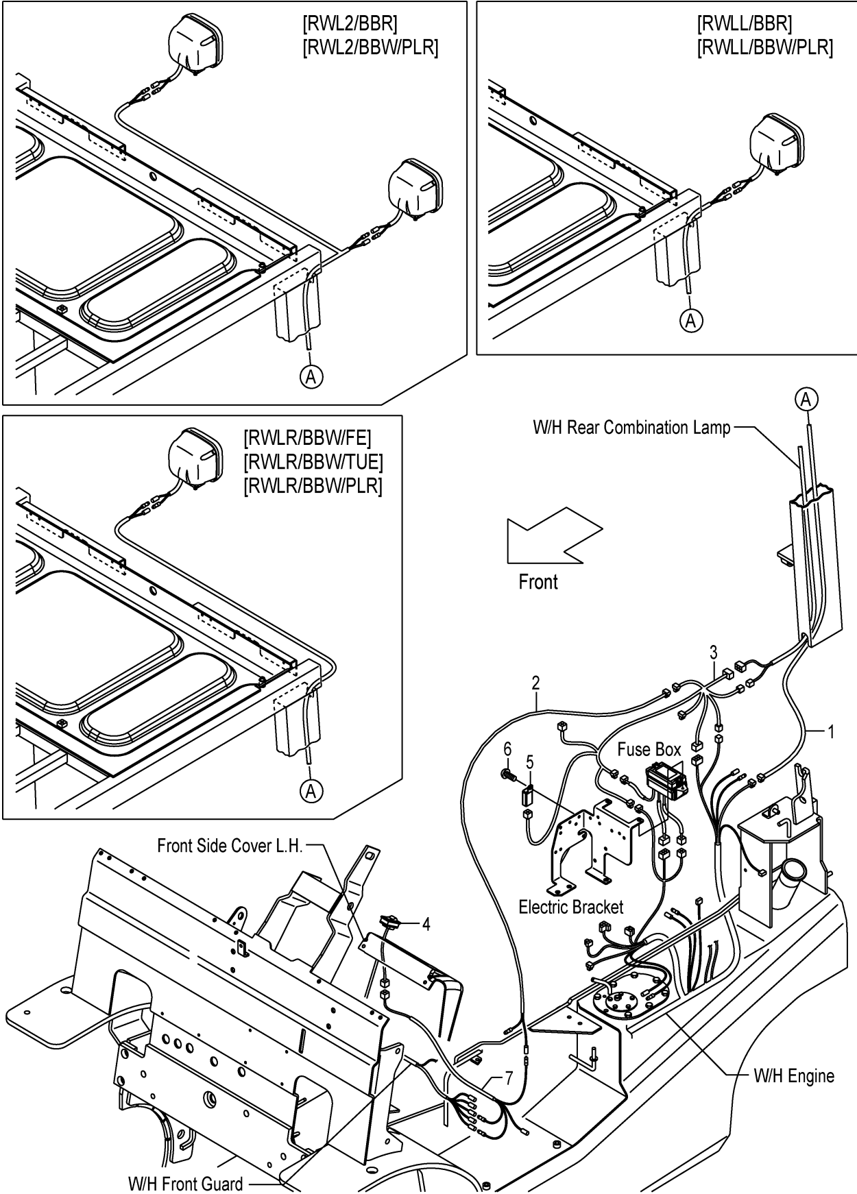
FIG.28 REAR WORKING LIGHT WIRE HARNESS [RWL/BBR] (F7Z124U0) リヤワーキングライトワイヤハーネス
