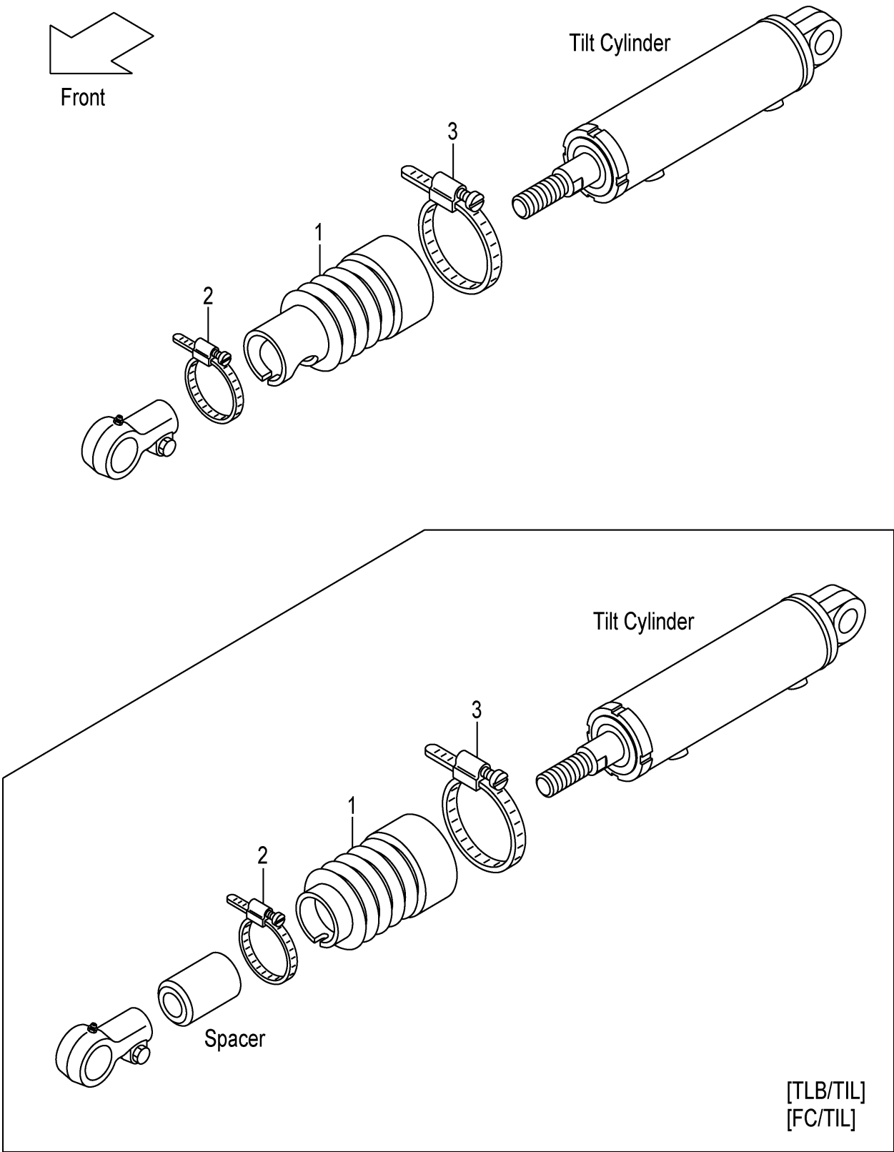
FIG.173 TILT BOOT [TLB][FC] (F7Z18520) ティルトブーツ
