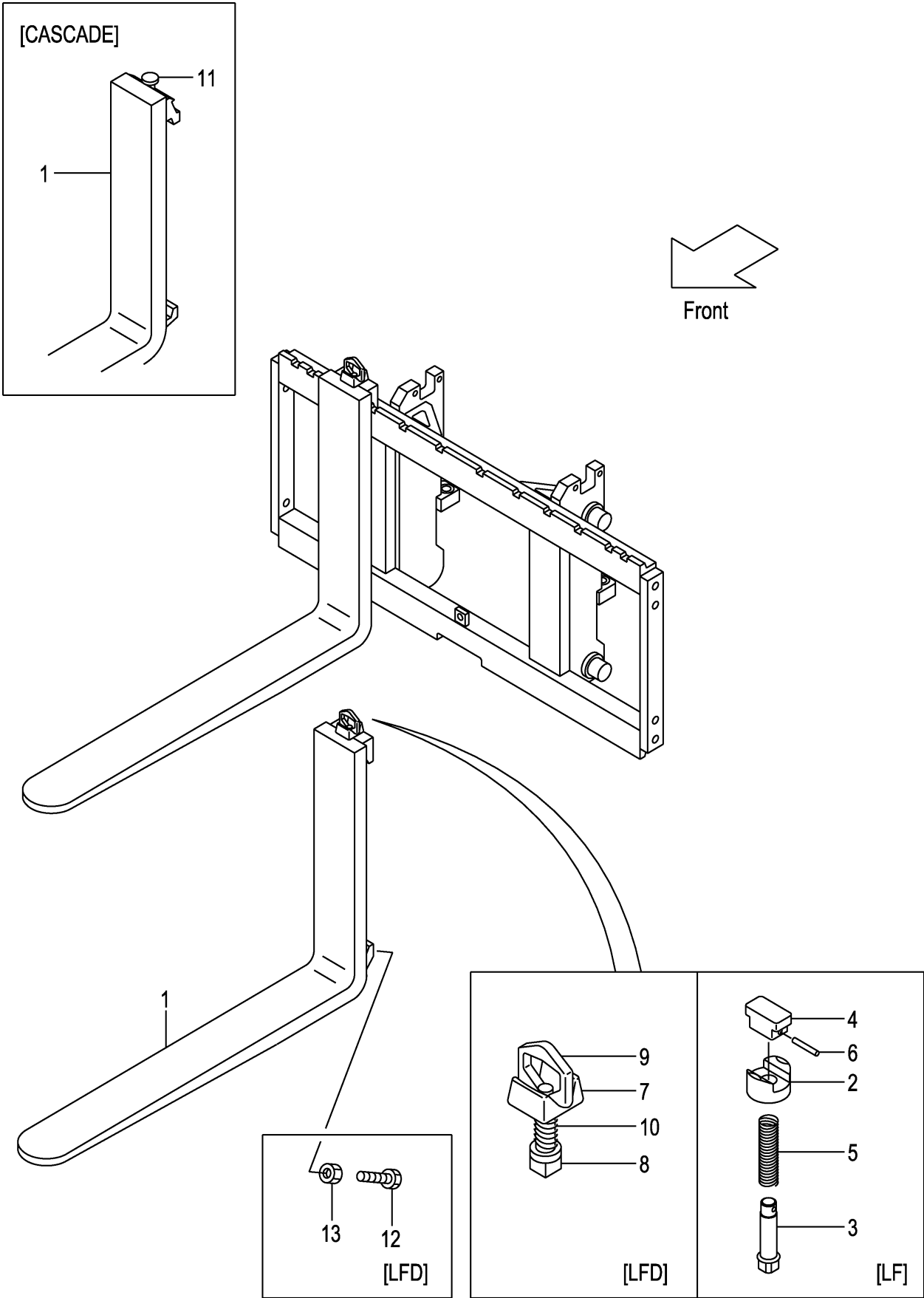
FIG.185 FORK [VM0A7,VM0A9] (M7018110) フォーク
