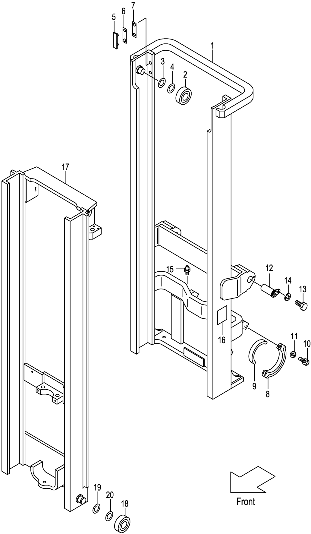
FIG.195 MAST [VFM0A7] (M7010410) マスト
