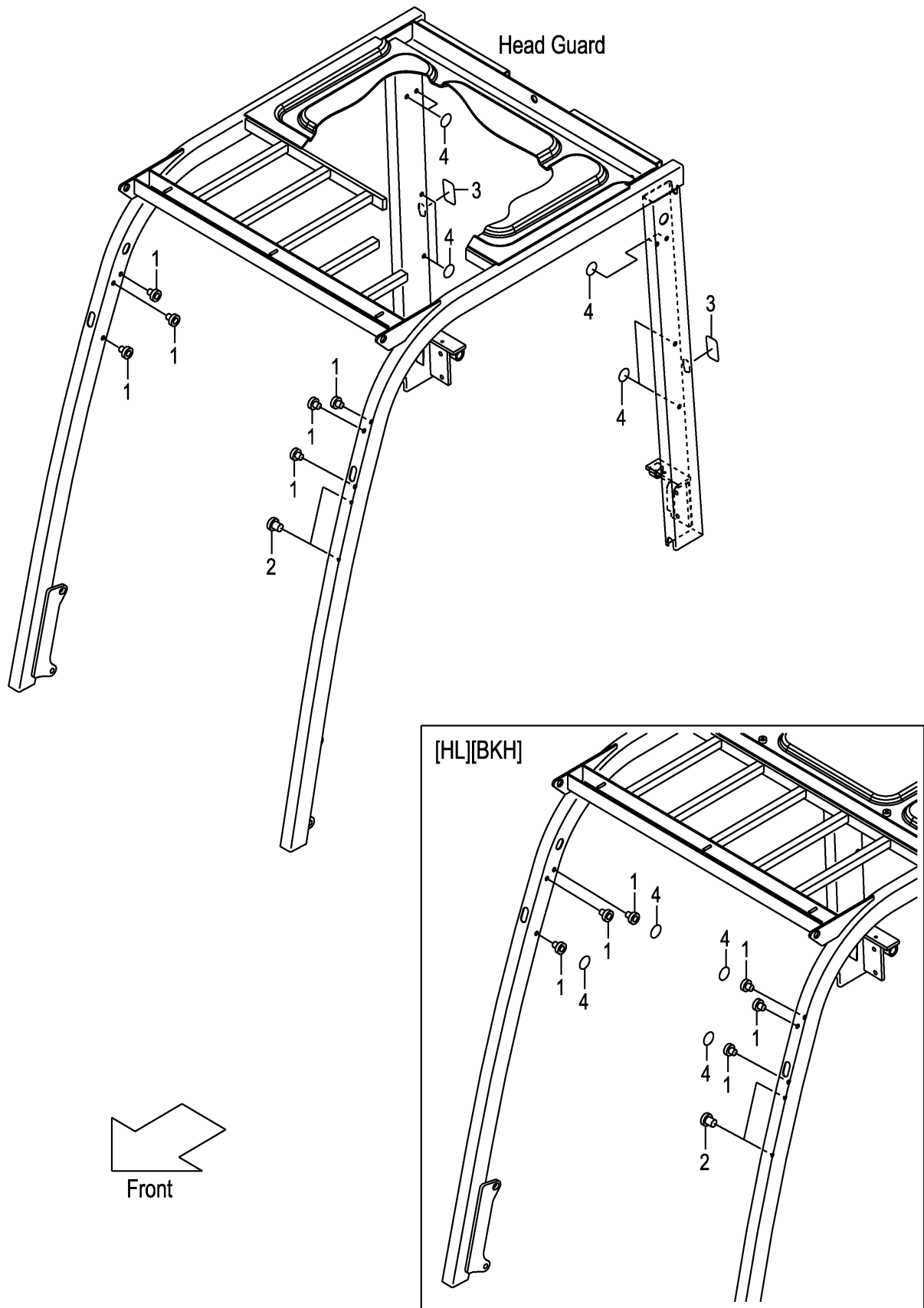
FIG.104 POP RIVET (F7Z151B0) ポップリベット
