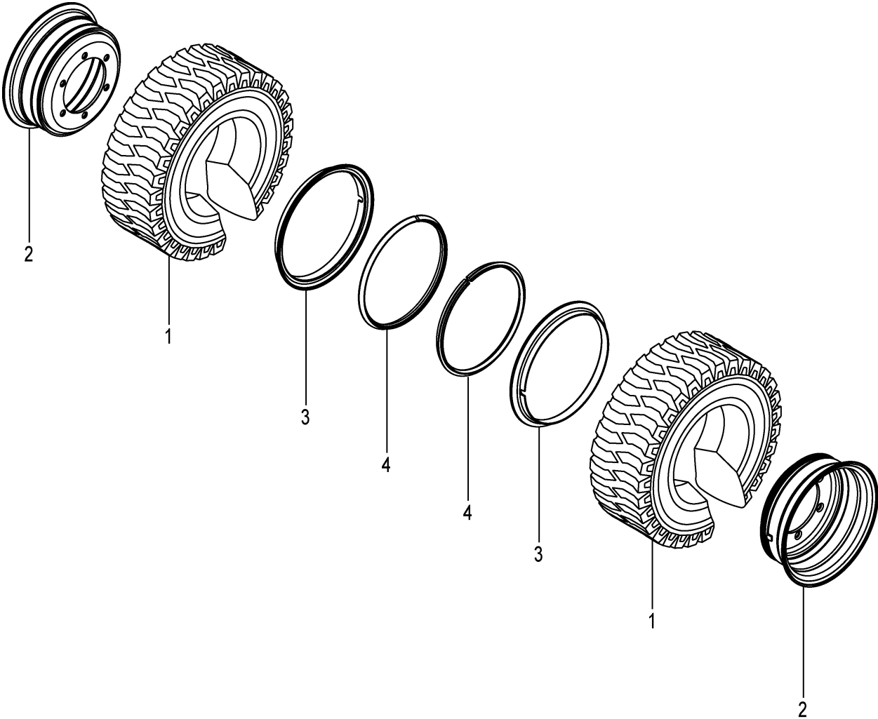
FIG.86 FRONT WHEEL [TUJW][TUSW][TUWW][TUGW] (F7Z144F0) フロントホイール
