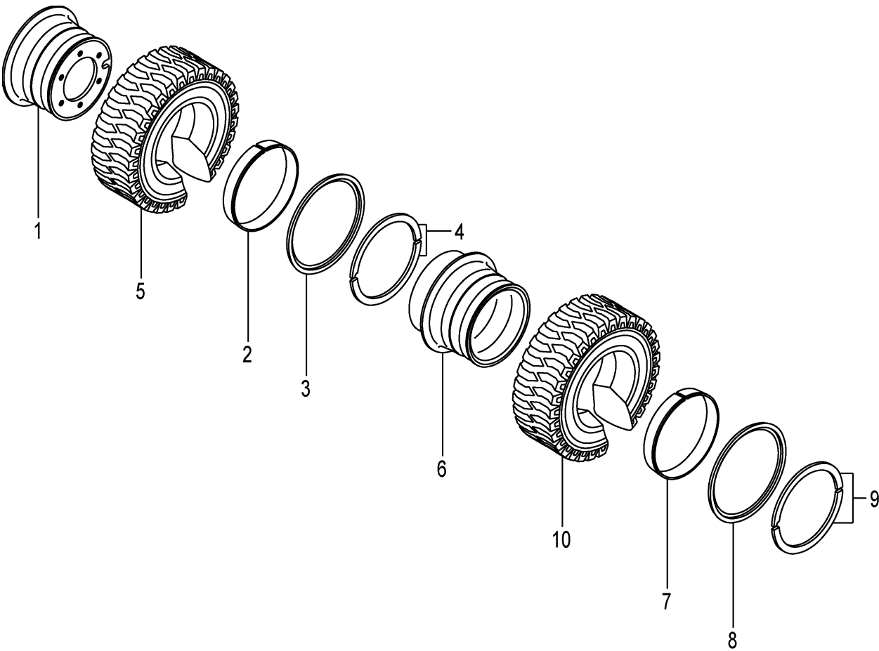
FIG.88 FRONT WHEEL [TUJW65][TUSW65][TUWW65][TUGW65] (F7Z144H0) フロントホイール
