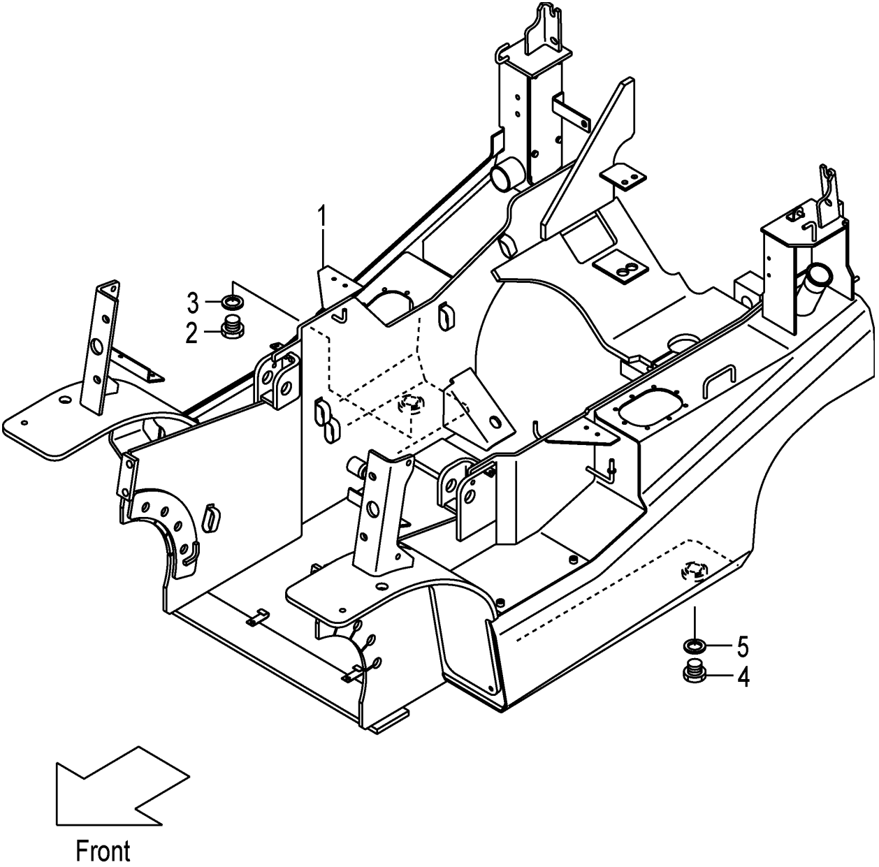
FIG.118 FRAME (F7Z16110) フレーム
