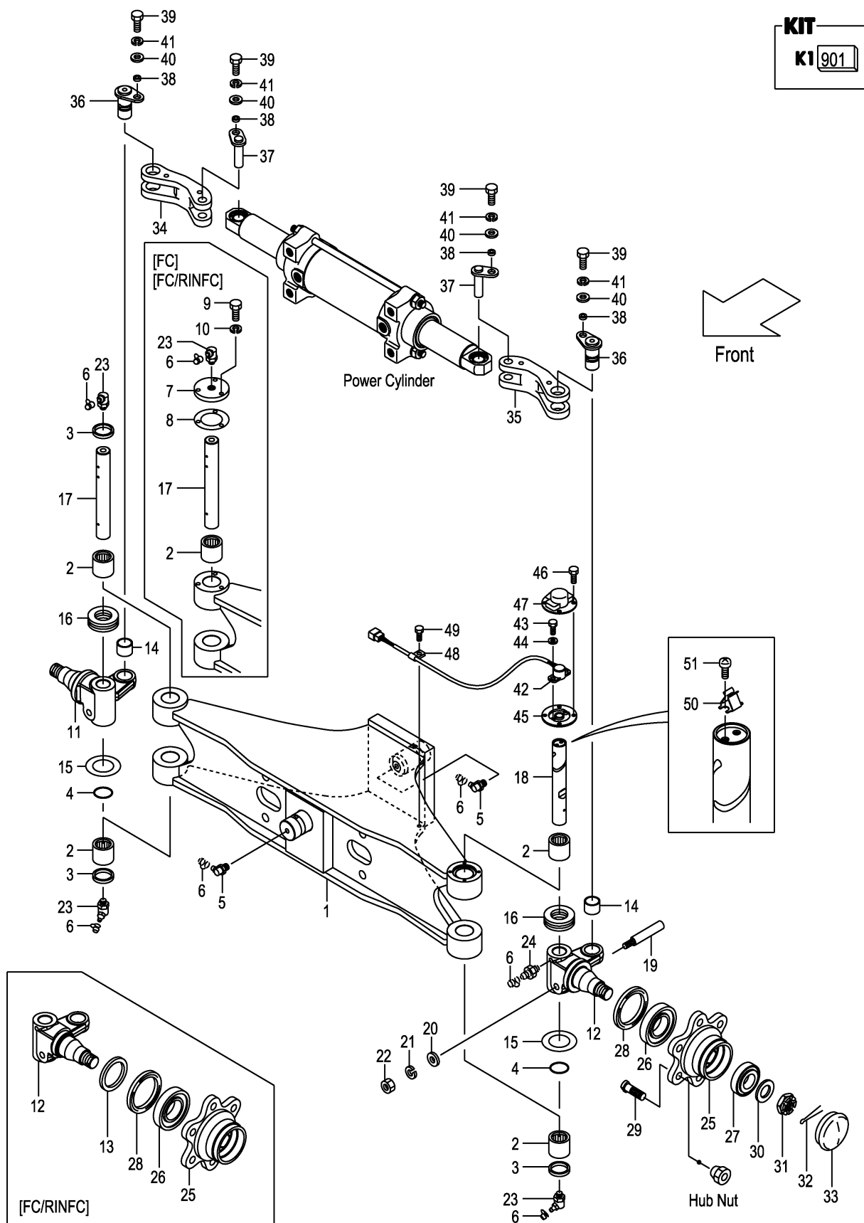
(F7Z14310) ステアリング・アクスル
