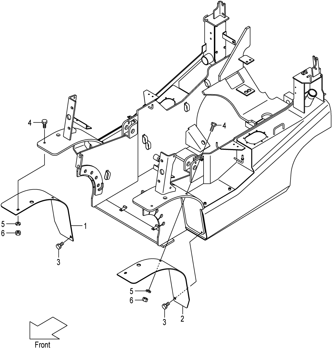
FIG.73 FENDER [DD][SDD] (F7Z14420) フェンダ
