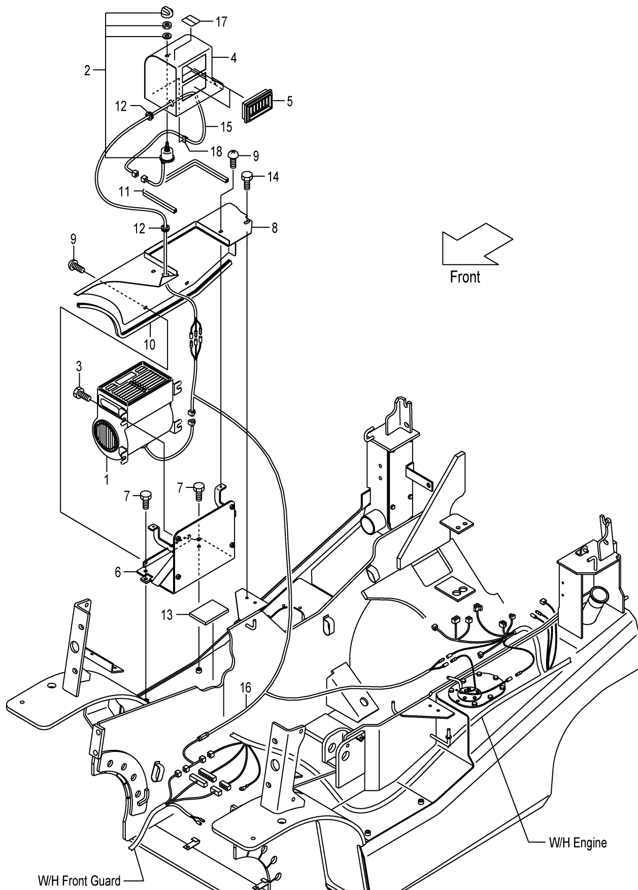
FIG.33 HEATER UNIT [HR] (F7Z124Y0) ヒータユニット
