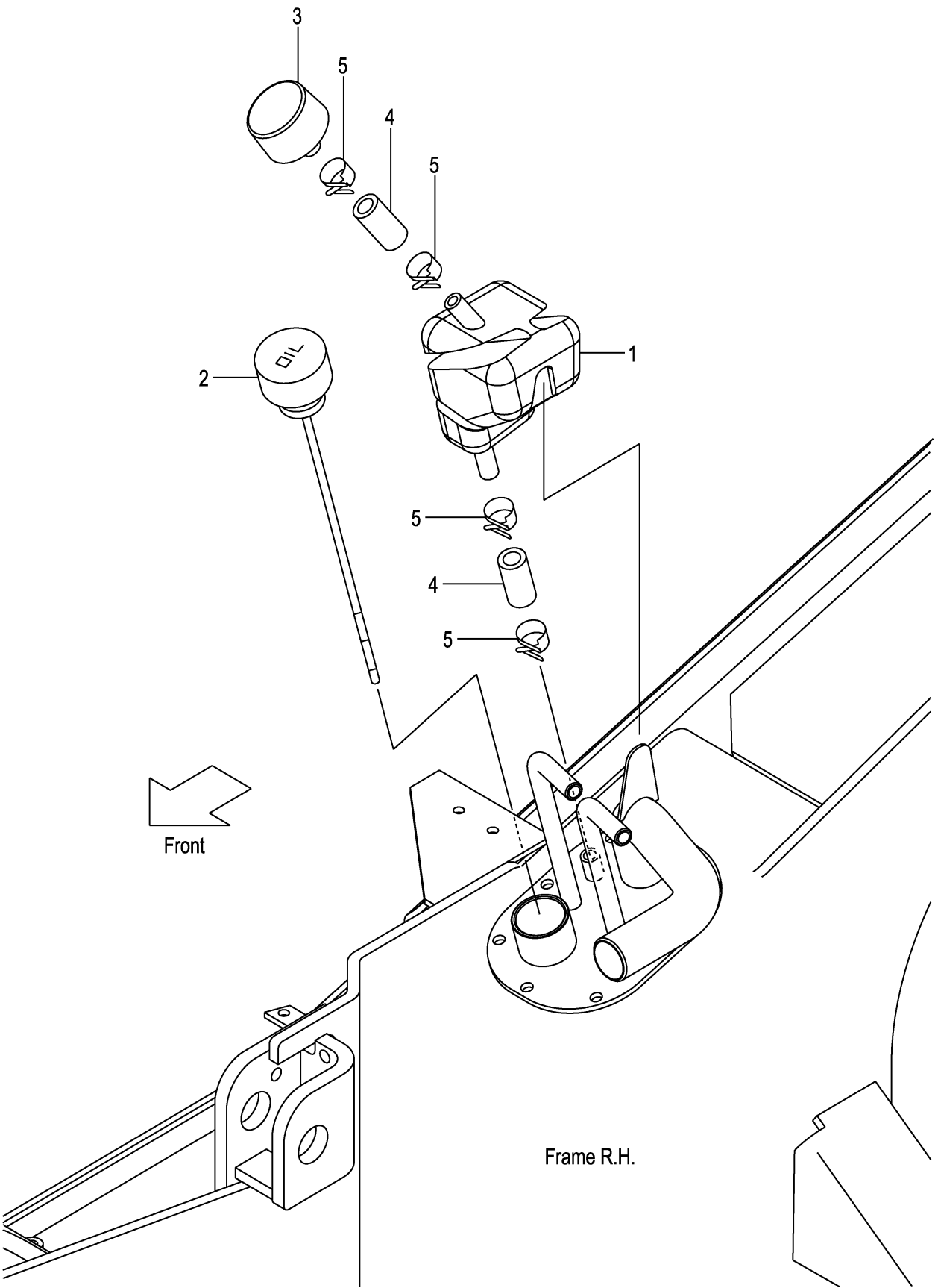
FIG.120A OIL CAP & LEVEL (F7Z16131) オイルキャップ&レベル
