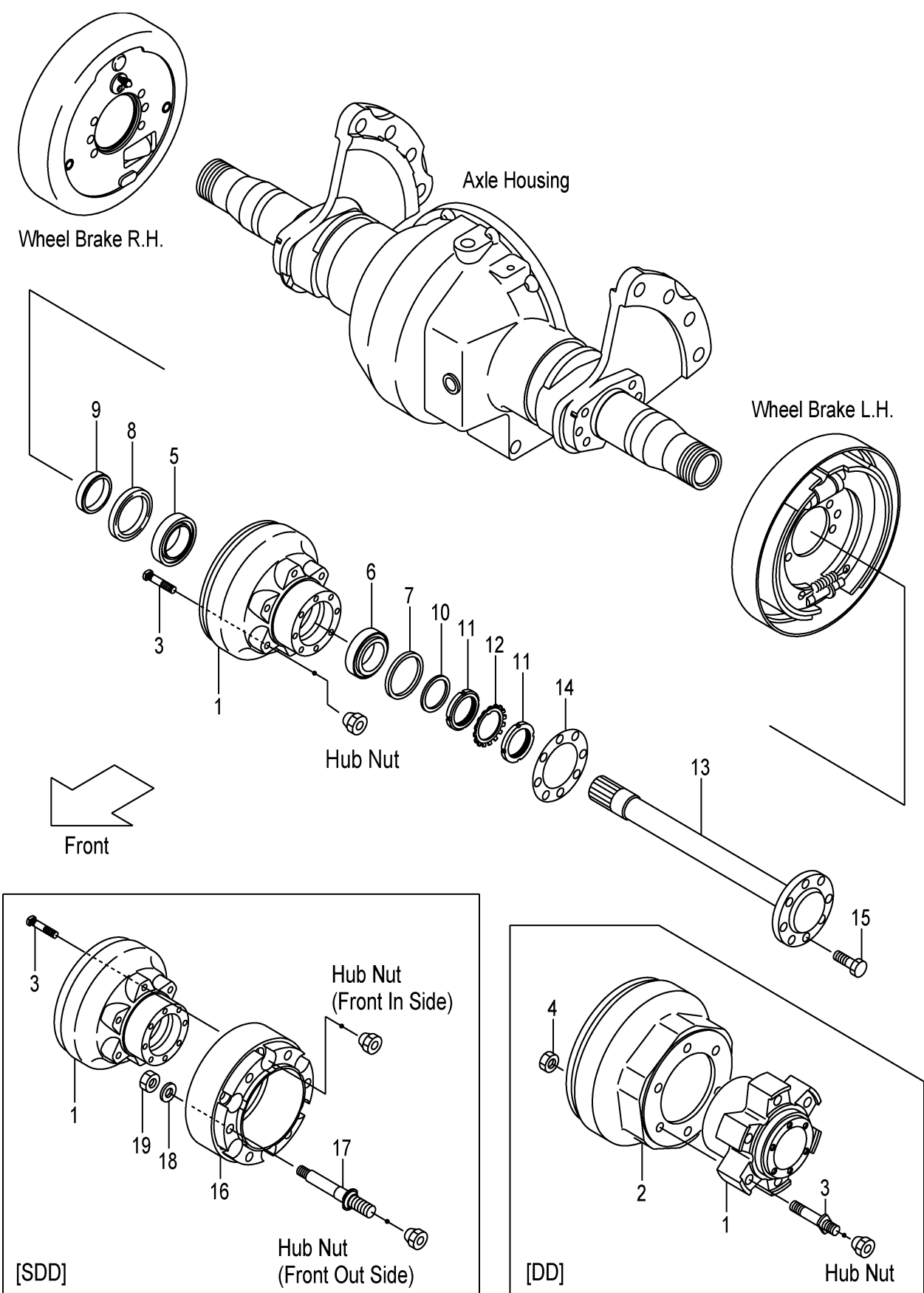
FIG.60 DRUM HUB (F7Z13020) ドラムハブ
