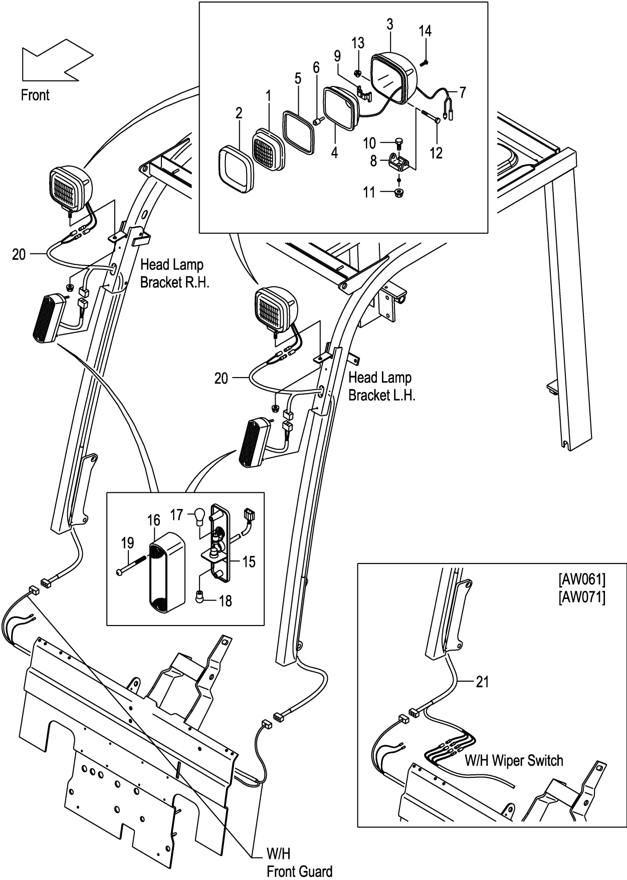
FIG.20 HEAD LAMP & FRONT COMBINATION LAMP (F7Z124G0) ヘッドランプ&フロントコンビネーションランプ
