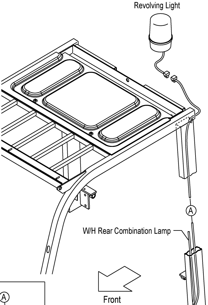
FIG.30 REVOLVING LIGHT WIRE HARNESS [RLY][RLR] (F7Z124W0) リボルビングライトワイヤハーネス
