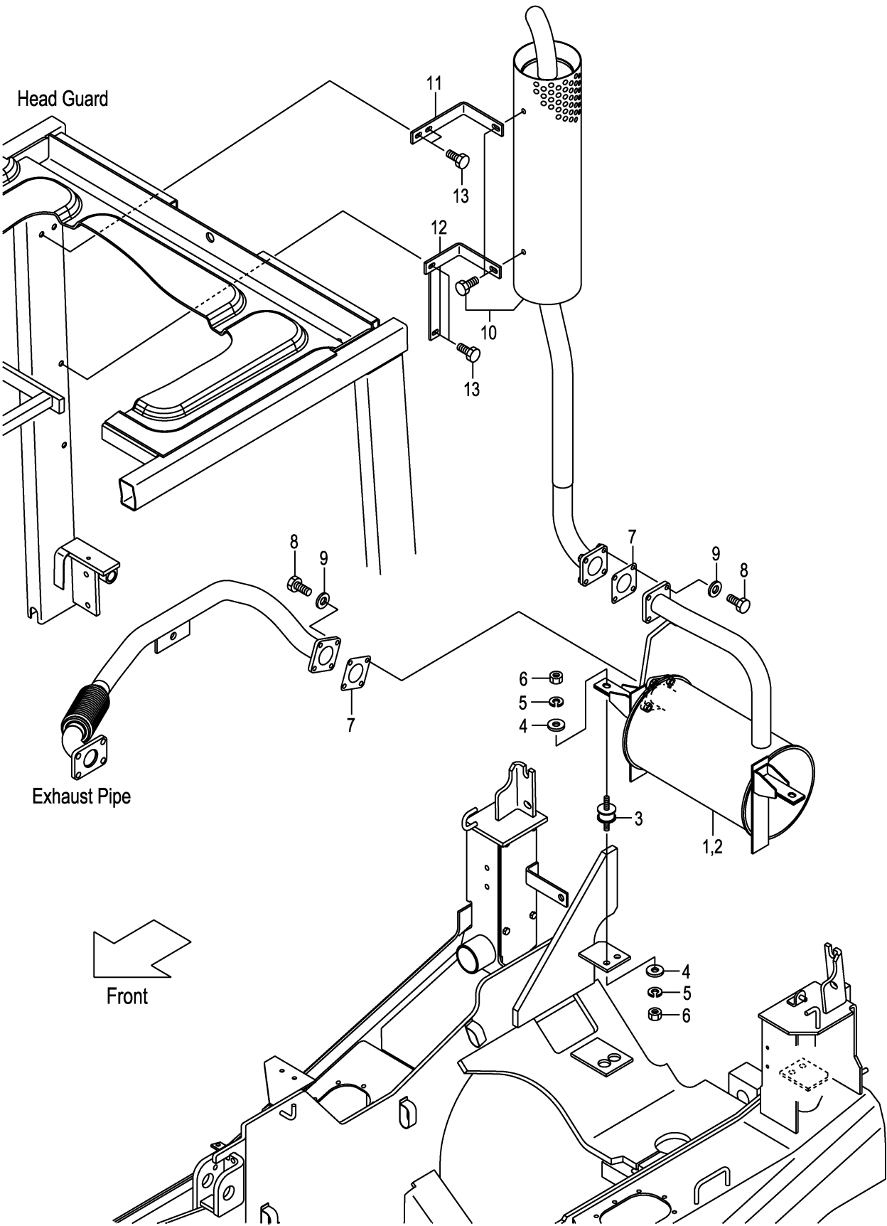
FIG.10 EXHAUST SYSTEM [TUE] (F7Z12330) エキゾーストシステム
