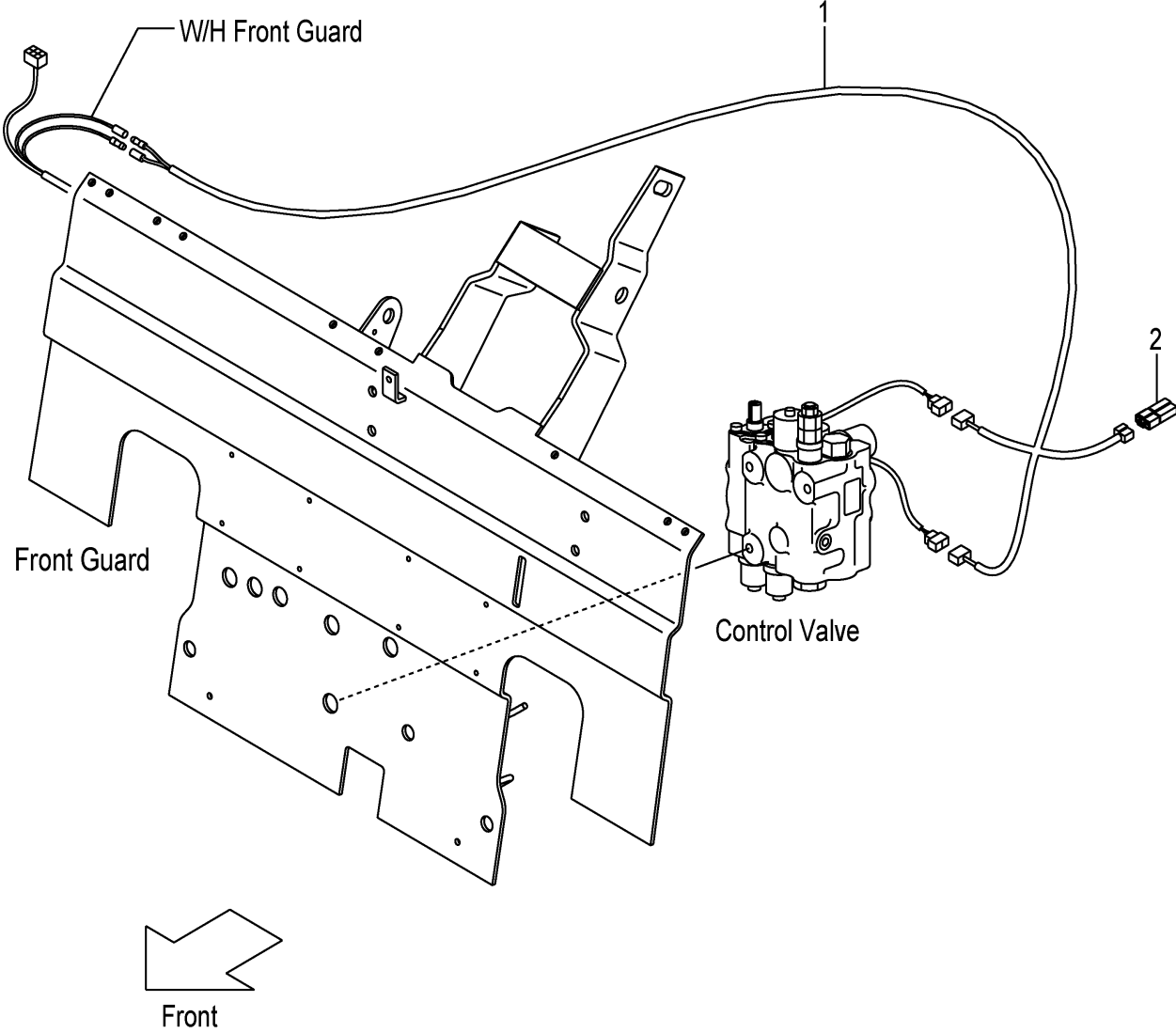
FIG.36 LIFT LOCK VALVE WIRE HARNESS [VLL] (F7Z12660) リフトロックバルブワイヤハーネス
